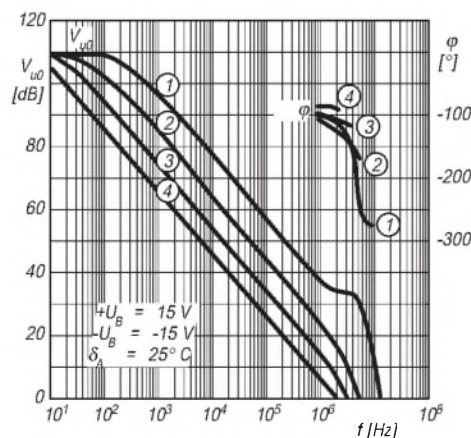
Bild 1: Leerlaufverstärkung und Phasenverschiebung über der Frequenz (1 Leerlauf, 2...3 R_L = 2 kW, C_L = 30 pF, 2 C_C = 15 pF, 3 C_C = 47 pF, 4 C_C = 150 pF)
