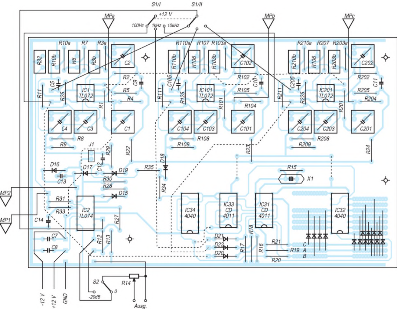
Bild 10: Bestückungsplan
