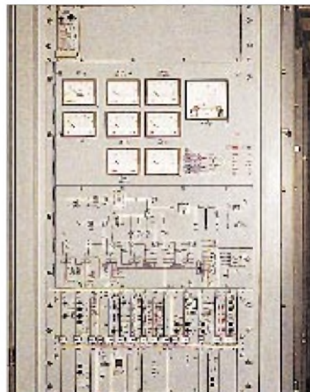
Bedienteil des Mittelwellensenders – oben Meßinstrumente für Leistungsanpassung und Röhrenkenngößen, in der Mitte Statusanzeigen, unten die Parametrierung
