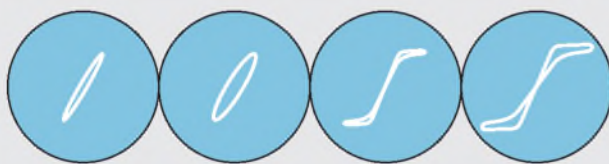
Bild 15: Formen der Aussteuerungskennlinien unterschiedlicher Verstärker bei zu großer Eingangswechselspannung (= Übersteuerung)
