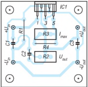
Bild 7: Die Bestückungsseite der Platine
