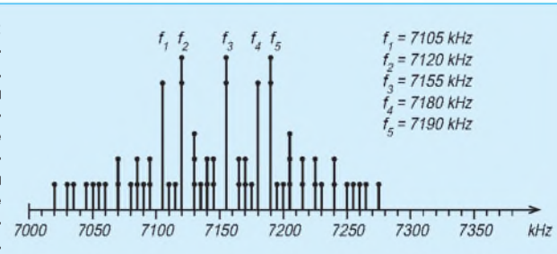
Bild 11: Fünftön-Intermodulation. Die doppelten Punkte symbolisieren die Spannungsüberhöhung durch mehrfache Intermodulationsprodukte.
