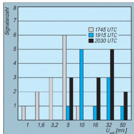
Bild 5: Pegelverteilung der Sender von Bild 1 bis Bild 3 im Bereich 7100 bis 7200 kHz
