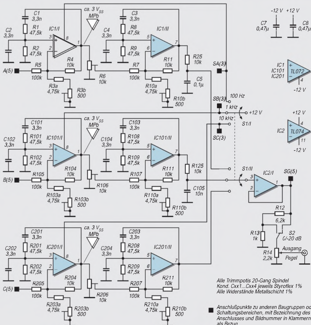
Bild 6: Doppelwienbrückenfilter für drei Frequenzen
