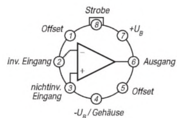
Bild 3: Anschlußbelegung Gehäuse TO-5
