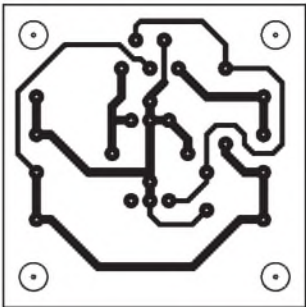
Bild 6: Die Lötseite der Platine. Bohrlöcher minimiert
