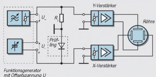
Bild 7: Skizze zur oszillografischen Darstellung der Kennlinien von Dioden oder Gleichrichtern mit und ohne einer Vorspannung in Sperr-Richtung
