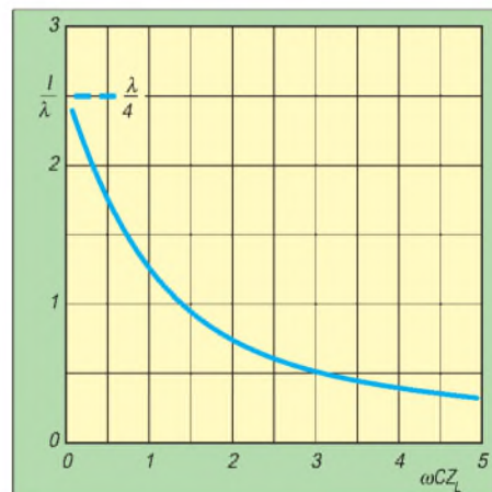
Bild 3: Topfkreislänge als Funktion der Abstimmkapazität, jeweils normiert. Z_L ist der Wellenwiderstand des Resonanzsystems, C die Last- (Abstimm-)kapazität. Das Produkt \omega C \cdot Z_L ist ohne Dimension.
