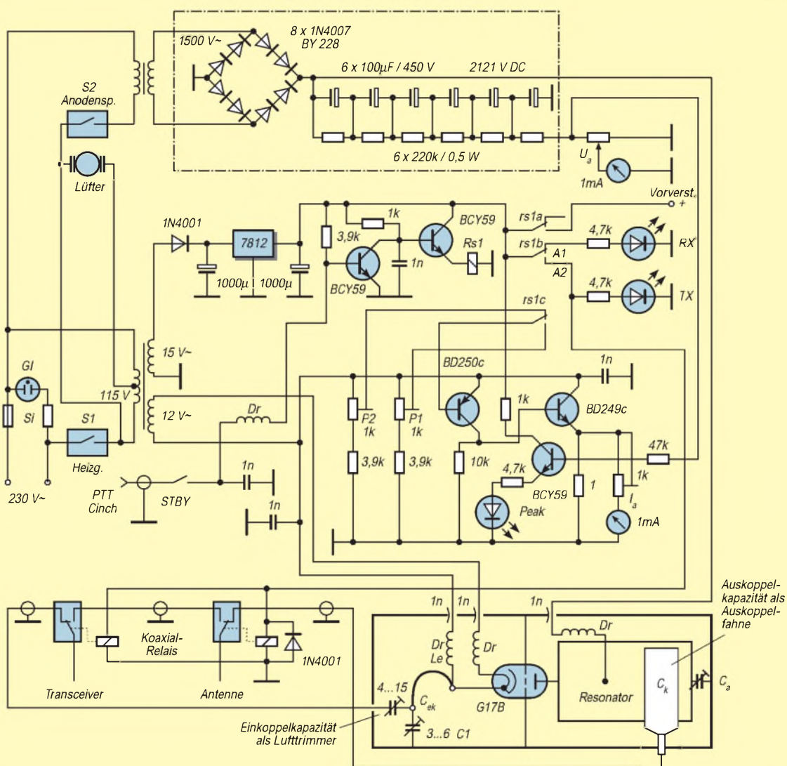
Bild 6: Stromlaufplan der 70-cm-Endstufe. Mit P1 wird der Vorwärm-, mit P2 der Ruhestrom im Sendebetrieb eingestellt. Die beiden Instrumente für Anodenstrom und -spannung wurden beim Mustergerät durch einen Umschalter ersetzt. Die Drosseln sind sämtlich sog. \lambda/4 -Drosseln, also 170 mm Draht zu einer freitragenden Spule gewickelt, L_e s. Text. Der Abstimmkondensator C_a wird ähnlich wie der Auskoppelkondensator C_k durch einen per Spindel verstellbaren Blechstreifen realisiert.
