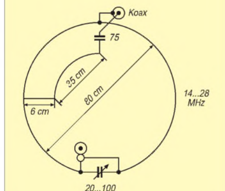
Bild 10: Aufbauskeizze einer Magnetantenne mit Gamma-Anpassung als Einkopplung [19]
