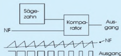
Bild 3: Ein Pulsbreitenmodulator vergleicht das Eingangssignal mit der aktuellen Amplitude des Sägezahnsignals.
