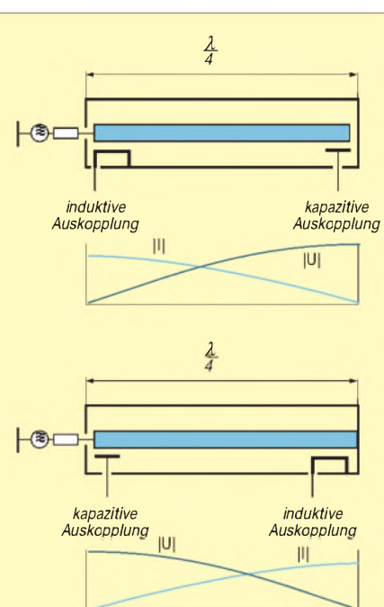
Bild 7: Mögliche Auskoppelstellen am \lambda/4 -Topfkreis; oben leerlaufender, unten kurzgeschlossener Resonator
