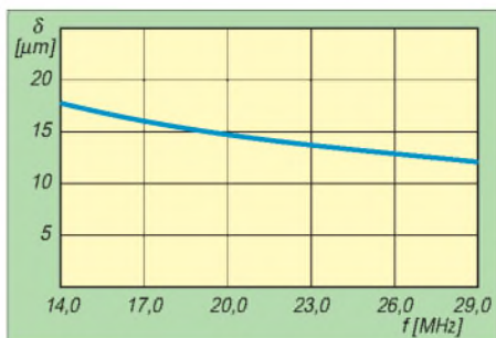
Bild 3: Eindringtiefe δ in Abhängigkeit von der Betriebsfrequenz
