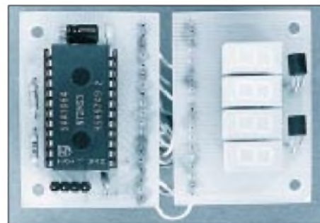
Bild 13: Die beiden Platines des Displays im aufgeklappten Zustand
