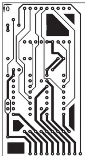
Bild 11: Leiterplatte Anzeige SSA (Lötseite)
