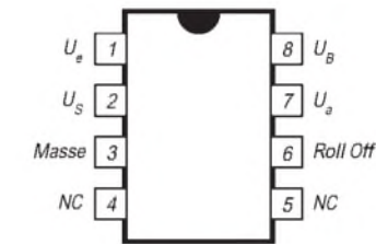
Bild 1: Anschlußbelegung
