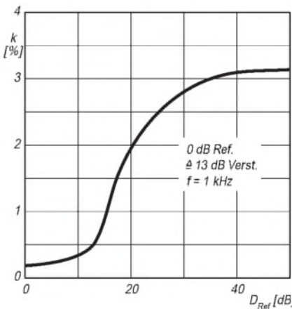
Bild 3: Klirrfaktor als Funktion der Dämpfung
