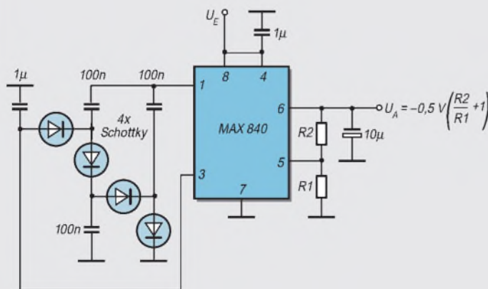
Bild 15: Die Ausgangsspannung des MAX 840 ergibt sich mit der internen Referenzspannung 500 mV sowie R_1 und R_2 , deren Werte im zweistelligen Kilohmbereich liegen können. Natürlich ist für eine bestimmte Ausgangsspannung eine minimale Eingangsspannung erforderlich.
