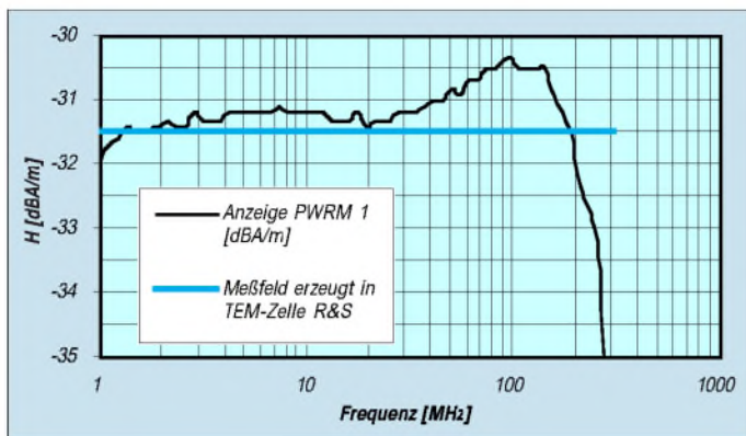
Bild 2: Magnetische Feldstärke, Referenzfrequenzgang: HFS1 mit PWRM1, Referenzpegel -31,5 dBu/m entspr. 10 V/m; Überlagerung des von der HFS1 abgegebenen Signals mit dem Frequenzgang des PWRM1; Messung in R&S-TEM-Zelle S-Line 700), Sonde direkt mit PWRM1 verbunden
