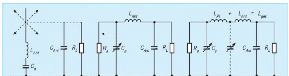
Bild 1: Veranschaulichung des fiktiven Antennenlastwiderstands R_L (strahlungsbedingt, zugeordnet), C_{Ant} – Antennenkapazität, L_{Ant} – Antennenverlängerungsspule (links)
