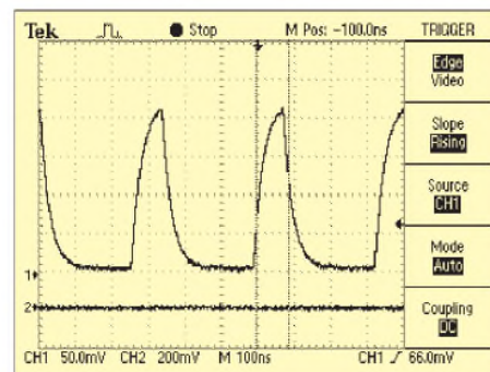
Bild 7: Testsignal von Bild 3 auf einem DSO ohne Runt-Trigger. Durch die geringere Erfassungshäufigkeit wird dieser Runt einfach nicht sichtbar.
