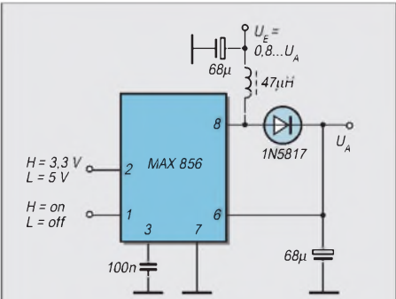
Bild 3: Standardapplikation für den MAX 856. Interne Strombegrenzung ermöglicht die relativ kleine Induktivität. Beim MAX 858 genügen 22-µF-Elkos.
