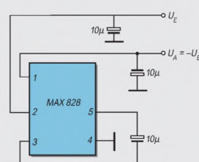
Bild 7: Der MAX 828 benötigt neben der U_E -Blockung prinzipiell nur zwei Elektrolytkondensatoren als Außenbeschaltung. Beim MAX 829 können alle Kondensatoren auf 4,7 µF oder 3,3 µF verkleinert werden.
