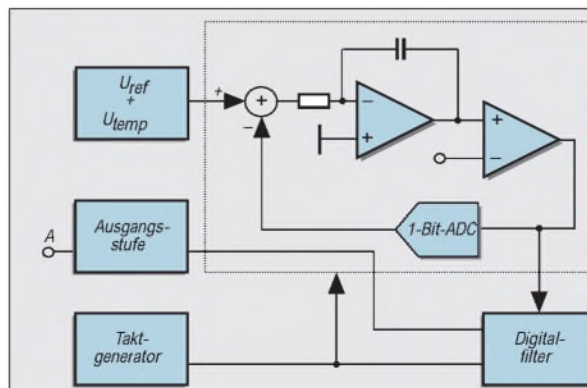
Bild 2: Prinzipielle Innenschaltung der Temperatursensor-ICs TMP 03/TMP 04
