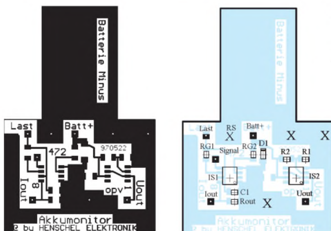
Bild 2: Platinenlayout
