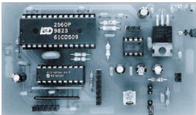
Bild 6: Foto der Platine MEM-C 03, bestückt und betriebsbereit
