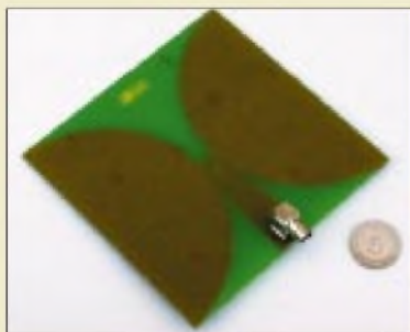
Die neue E-Feld-Sonde EFS-1 ist zum Amateurpreis erhältlich und wird kalibriert ausgeliefert, so daß der Anerkennung der gewonnenen Meßwerte nichts im Wege steht. Werkfoto
