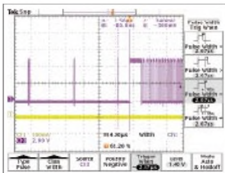
Bild 3: Triggerung auf eine kritische Impulsbreite mit der Puls-Width-Triggerart des DPO TDS 3034. Es sind auch noch sehr schmale Impulse klar erkennbar.
