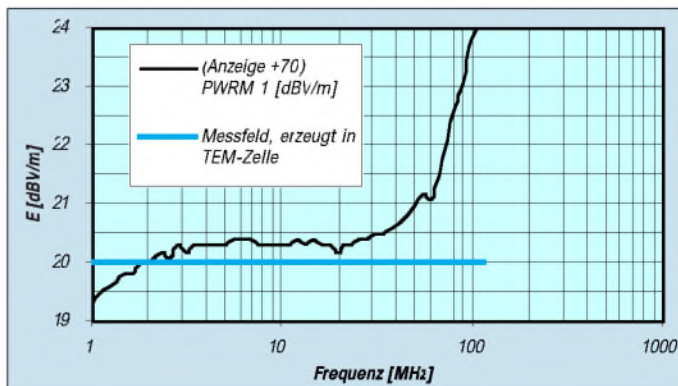
Bild 4: Elektrische Feldstärke, Referenzfrequenzgang: EFS1 mit PWRM1, Referenzpegel +20 dBV/m entspr. 10 V/m; Überlagerung des von der EFS1 abgegebenen Signals mit dem Frequenzgang des PWRM1; Messung in R&S-TEM-Zelle S-Line 700), Sonde direkt mit PWRM1 verbunden
