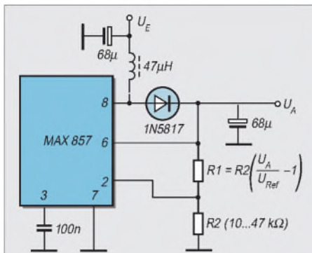
Bild 4: Standardapplikation für den MAX 857. Die kleine Induktivität wird durch interne Strombegrenzung möglich. Beim MAX 859 genügen 22 µF für die Elkos.
