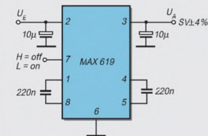
Bild 13: Der MAX 619 ist ein geregelter Ladungspumpen-IC. Seine Stromergiebigkeit richtet sich nach der Eingangsspannung.
