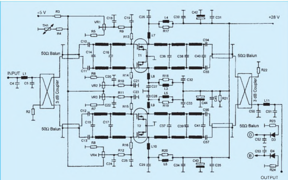
Bild 3: Schaltbild des HF-Teils der 300-W-Linearstufe. Die Aufspaltung des Signals für die Doppeltransistoren erfolgt über Powersplitter, während jeder einzelne Transistor von einem Koaxkabel-Balun aus versorgt wird.
