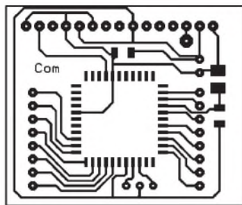
Bild 9: Die Platine für den Empfänger läßt sich in vielen Geräten nachrüsten.
