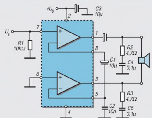
Bild 18: Brückenschaltung – einfacher geht's nicht
