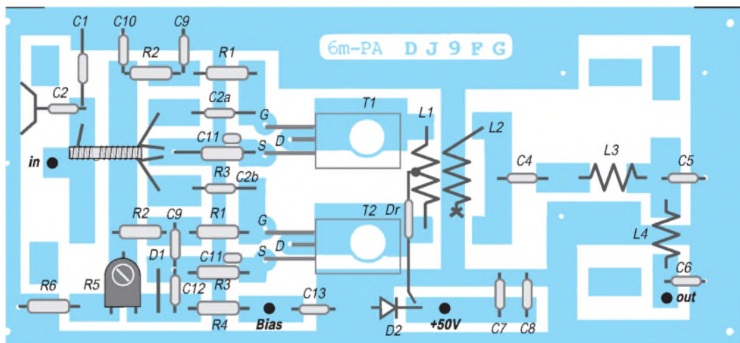
Bild 12: Bestückungsplan des Gegentaktverstärkers – die Bestückung erfolgt bis auf T1 und T2 auf der Leiterseite, Massepunkte sind durchzukontaktieren! L2 ist am masseseitigen Ende separat durchzukontaktieren. Die SMD-Kondensatoren C11a und C11b sind vor R3a bzw. R3b einzulöten. Notfalls eignen sich auch Scheibenkondensatoren bis 47 nF mit soweit wie möglich gekürzten Anschlußbeinen.
