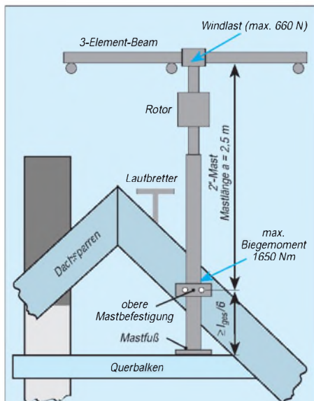
Bild 2: Prinzipskizze der Mastbefestigung für eine drehbare Antenne ohne Abspannung am Dachstuhl. Freie Zugänglichkeit des Laufsteges zum Schornstein ist eine Selbstverständlichkeit. Nach [4] darf ein Mastrohr oberhalb des Rotors maximal 1 m lang sein, wenn kein Oberlager zum Einsatz kommt.
