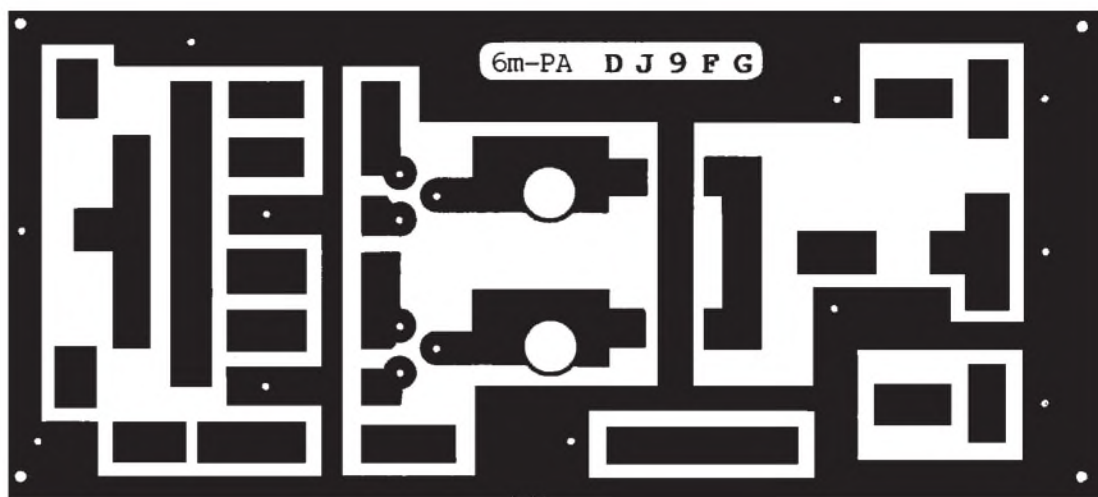
Bild 11: Leiterseite der Platine der Linearverstärker mit zwei Transistoren; sie eignet sich ggf. auch für eine Gleichaktvariante. Die Oberseite ist wieder eine durchgehende Massefläche. Die Platine ist so bemessen, daß sie in ein Standard-Weißblech- gehäuse mit den Maßen 74 mm x 148 mm x 50 mm paßt.
