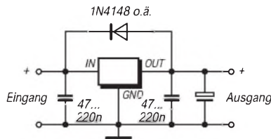
Bild 15: Grundbeschaltung der Festspannungsregler, positiv
