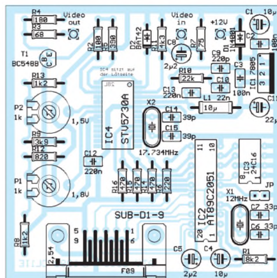
Bild 5: Bestückungsplan der Baugruppe ATV-LOGO; IC4 ist auf der Leiterseite untergebracht – seine Montage erfordert eine ruhige Hand und ein gutes Auge.
