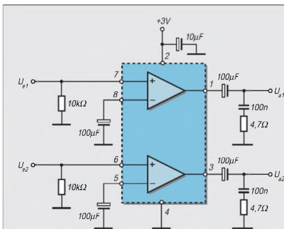
Bild 17: Der Mini-Doppelverstärker im Stereobetrieb
