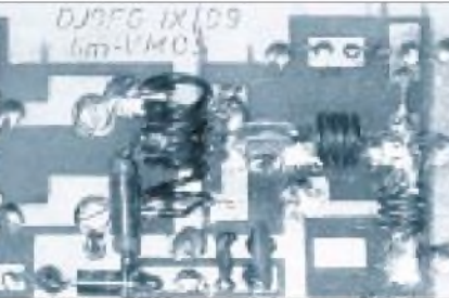
Bild 10: Blick auf den Ausgangsschwingkreis L1/L2 und die Draindrossel Dr
