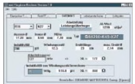
Bild 4: Berechnungsseite Epcos-Ringkerne
