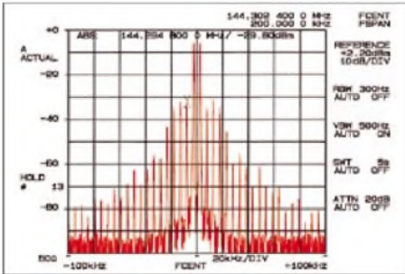
Bild 9: Ausgangsspektrum der Röhren-PA XL-144 bei Nennleistung, d.h., Speisung mit zweimal 64 W. IM3 beträgt -32 dBc; höhere IM-Produkte steigen im Pegel z.T. wieder an.
