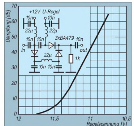
Bild 9: Dämpfung des aus drei PIN-Dioden bestehenden Dämpfungsglieds
