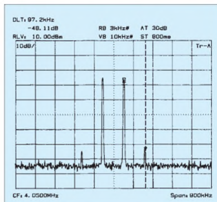
Bild 12: Intermodulationsprodukte mit -48 dBc im abgeregelten Zustand
