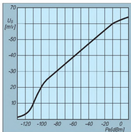
Bild 16: Gemessene S-Meterkurve mit beachtlichen 120 dB Anzeigeumfang
