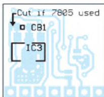
Bild 5: Bestückung auf der Oberseite (links)
