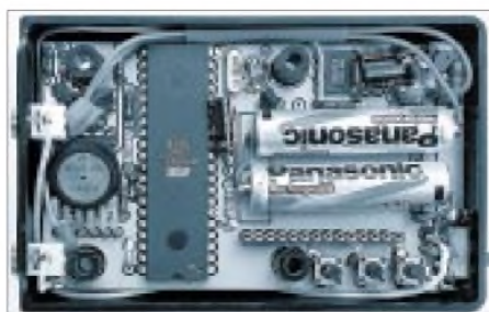
Bild 8: Die Stromversorgung wird durch zwei NiMH-AAA-Batterien realisiert.
