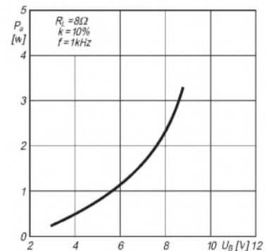
Bild 11: Brücken-Ausgangsleistung und Versorgungsspannung
