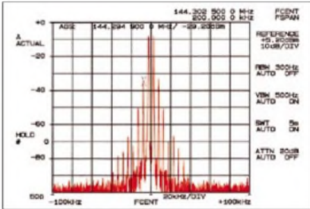
Bild 7: Ausgangsspektrum der HLV-600 bei 1,5 dB unter Nennleistung, d.h. Speisung mit zweimal 106 W. IM3 sinkt auf -34 dBc, und das Spektrum wirkt noch sauberer.
