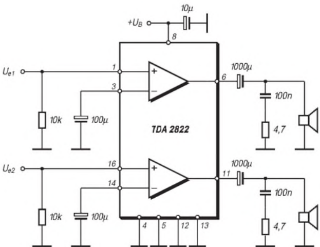
Bild 2: Die typische Stereokonfiguration verstärkt mit je 39 dB.
