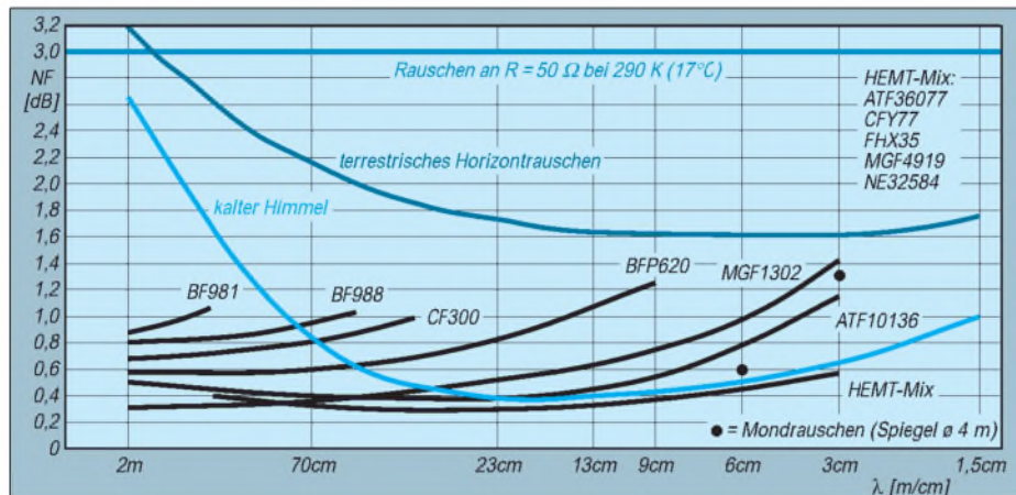
Bild 3: Rauschmaß NF (nicht zu verwechseln mit Niederfrequenz !) einiger Halbleiter 1 über den Frequenzbereich von 144 MHz bis 24 GHz im Vergleich zu anderen Rauschquellen 1 ) Hersteller: ATF36077/10136 Agilent, BF981 Philips; BF988, CF300 Telefunken; BFP620, CFY77 Infineon; FHX35 Fujitsu; MGF4919 Mitsubishi; NE32584 NEC
