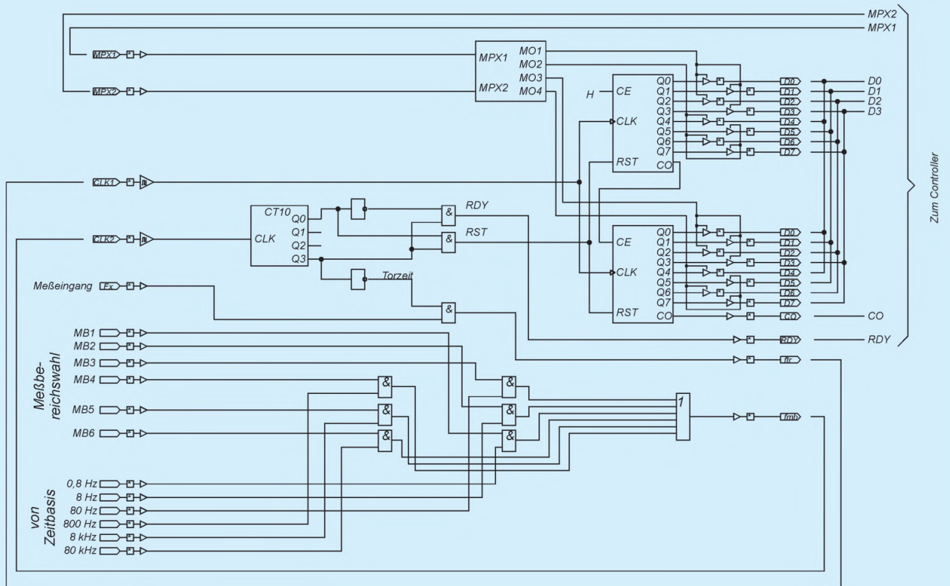
Bild 58: Die Gesamtschaltung des Zählers zeigt das Innenleben. Die äußere Beschaltung ist angedeutet.
