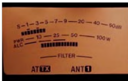
Das Balken-Meter zeigt sogar Kompressionsgrad des Sprachprozessors sowie SWR bis einschließlich 6 m an. Interessant: Ein Teilstrich am S-Meter symbolisiert jeweils 4 dB.
