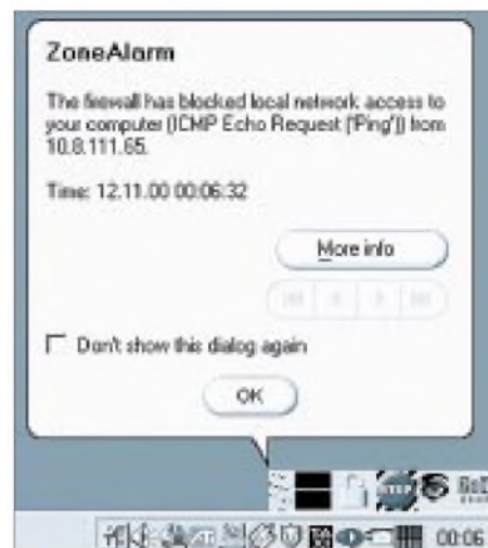
Bild 4: Erfolgt von außen auf Ihren Computer ein Zugriff, gibt ZoneAlarm eine Warnmeldung aus.
