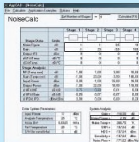
Bild 3: Die Gratisgabe AppCAD der Entwicklungsingenieure von HP (jetzt Agilent) läßt sich intuitiv bedienen und erspart lästige manuelle Rechnungen. Screenshot: DL2RD
