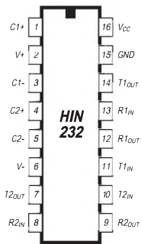
Bild 1: Pinbelegung
