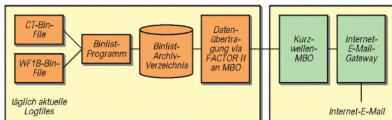
Bild 1: Datenfluß zur Erzeugung und Übertra- gung von Logdaten für die Online- Suche
