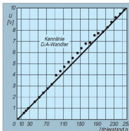
Bild 3: Kennlinie D/A-Wandler
