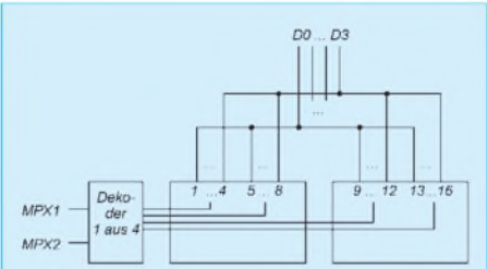
Bild 57: Beim Multiplexbetrieb mit 4 x 4 Bit benötigen wir insgesamt sechs Leitungen.
