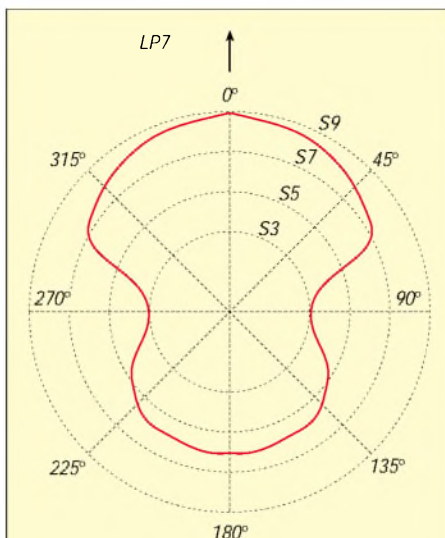
Bild 6: Richtdiagramm der LP7, aufgenommen mit einem kalibrierten S-Meter; tnx auch an Josef, DL4ZU, für die Mithilfe beim Messen.
