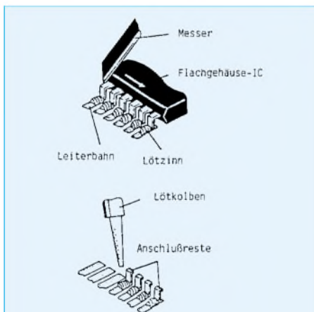
Bild 6: Hier werden die Anschlüsse mit einem Messer durchtrennt und die Pins dann einzeln herausgelötet.
