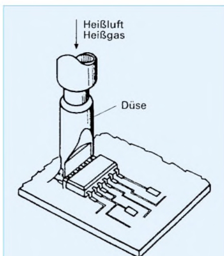
Bild 3: Die Heißluftdüse – eine sinnvolle Löthilfe
