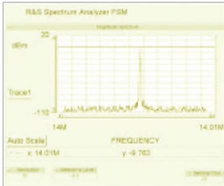
Bild 12: Das Spektrumanalysebild zeigt bei 14 MHz auch in Trägnähe niedrige Rauschwerte.
