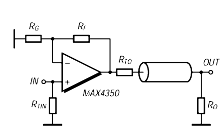
Bild 13: Konfiguration als nichtinvertierender Verstärker
