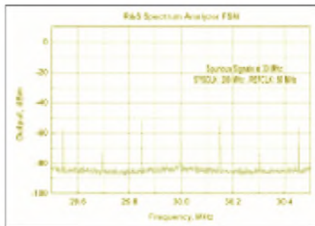
Bild 14: Die in der Nähe von 30 MHz Ausgangsfrequenz beobachteten Nebenlinien (ca. -45 dB) stören im Direktmischempfänger nicht, da sie bereits außerhalb des Audio-Filterbereichs liegen.
