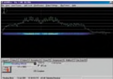
Bild 8: Screenshot einer Telemetriedatenauswertung mit AO40Rcv, V 1.40, von AE4JY
