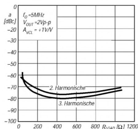
Bild 12: Verzerrungseigenschaften bei f_0 = 5 \text{ MHz} und A_{VCL} = +1 \text{ V/V} als Funktion des Lastwiderstands
