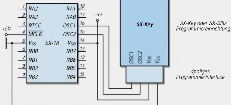
Bild 8: „SX-Key“, das Bindeglied zwischen seriellen PC-Port und dem SX, notwendig zur einfachen Programmierung des Bausteins und zum Softwaretest über den PC.
