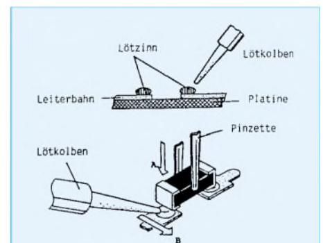
Bild 7: Grundsätzliches Vorgehen beim Einlöten von SMD-Bauteilen
