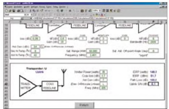
Bild 10: Tabellenkalkulation des U-Uplinks mit 30 W HF an einer linear polarisierten 10-Element-Yagi
