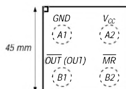
Bild 1: Pinbelegung des 4-Bump-Chipgehäuses (Miniaturlbauform, 70% kleiner als SC70-Bauform)
