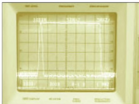
Bild 13: VFO-Frequenzgang von 40...70 MHz in spektraler Max-Hold-Einstellung
