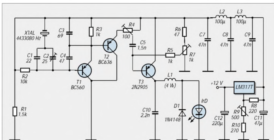
Bild 3: Senderschaltung mit Oszillator, Spannungsverstärker und Stromtreiber
