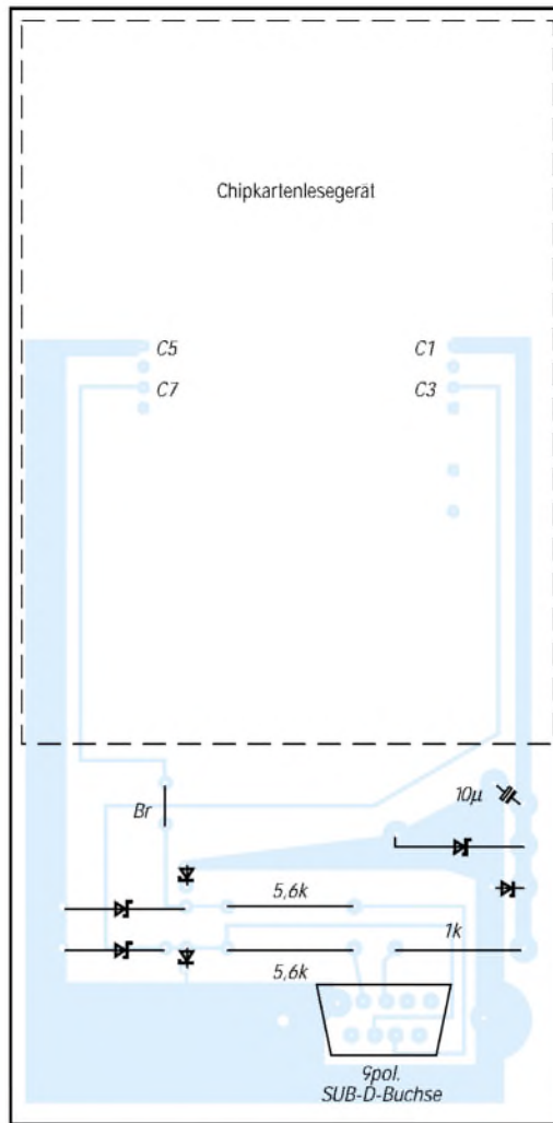
Bild 3: Bestückungsplan
