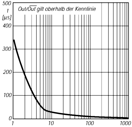
Bild 6: Maximale Transientendauer in Abhängigkeit von der Schaltschwellenüberlagerung U_{TH} - U_B (in mV)
