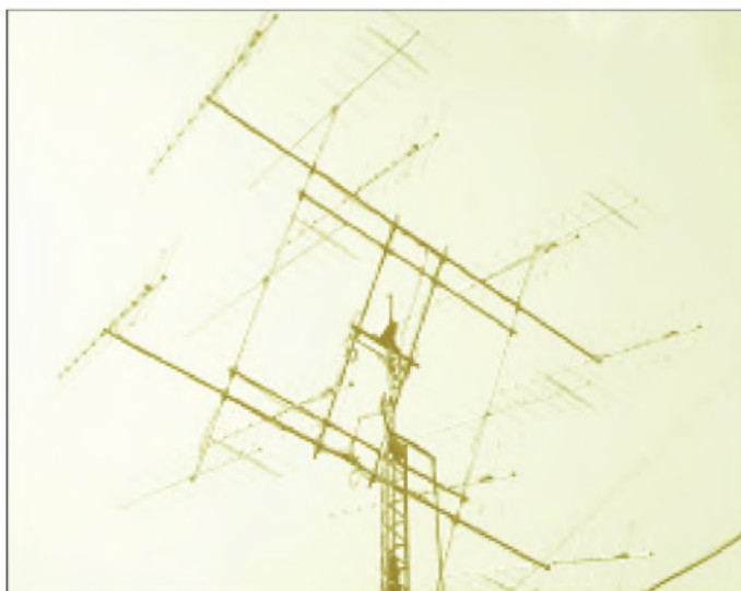
Bild 12: Zwei ineinander verschachtelte Antennensysteme, bestehend aus sechs Horizontal- und acht Vertikalyagis, bei JN1CSO
