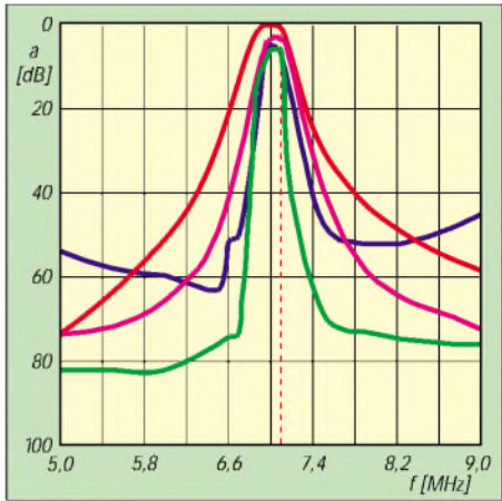
Bild 25: Durchlaßkurven von 40-m-Bandpaßfiltern; rot – LC-Filter, dreikreisig, simuliert bzw. lila – realisiert; blau: Piezofilter, einfache Variante (Bild 23), grün mit LC-Kreisen (Bild 24)
