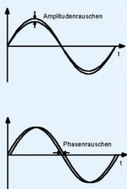
Bild 7: Phasen- und Amplituden- rauschen eines Oszillatorsignals im Zeitbereich
