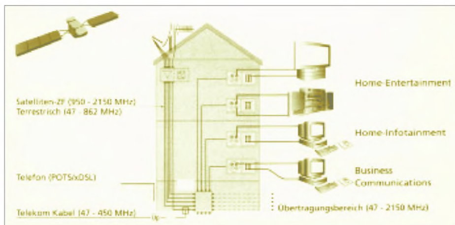
Bild 3: Kabelfernsehen und Sat-ZF-Verteilung ergänzen sich nach einem Astra-Vorschlag Quelle: Astra-Marketing-GmbH
