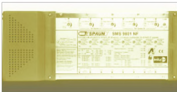
Bild 4: Multischalter SMS 9940NF von SPAUN zur Durchschleifung und Verteilung von acht SAT-ZF-Ebenen (z.B. viermal Astra 19° und viermal Eutelsat 13°) sowie eines terre- strischen oder Kabel-TV-Signals von 47-862 MHz
