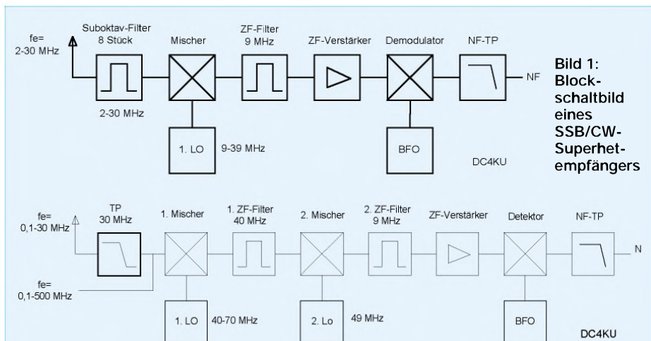
Bild 2: Blockschaftbild eines SSB/CW-Doppel-Superhetempfängers mit hochliegender 1. ZF
