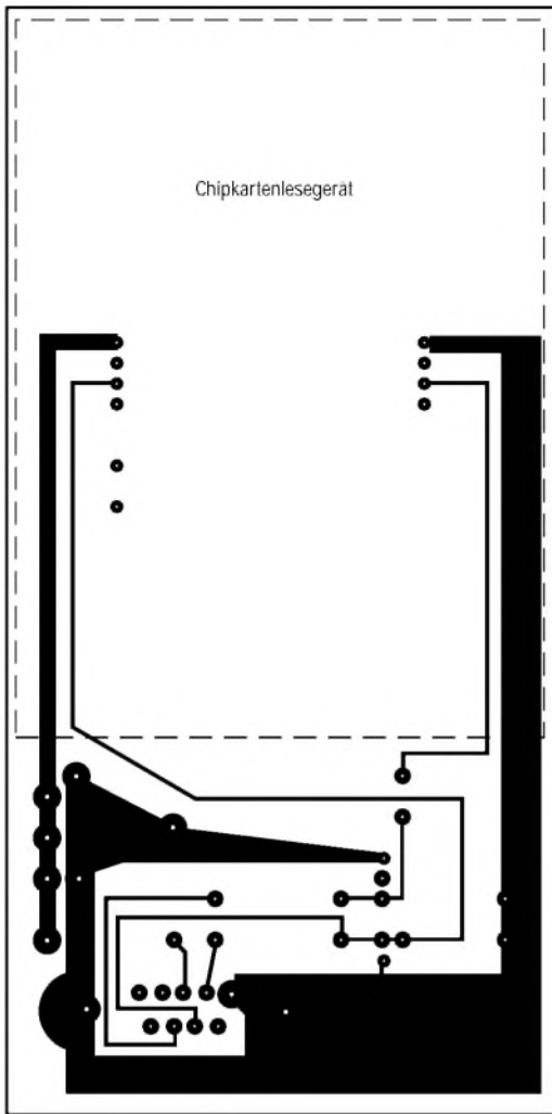
Bild 2: Platinenlayout
