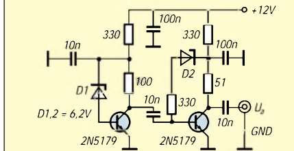
Bild 6: Rauschgenerator mit zwei Z-Dioden (5,1 bis 6,2 V) als Rauschquelle [17]
