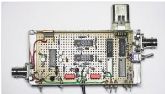
Bild 18: DAFC-Aufbau, links Zählereingang, rechts Eingang für die externe Referenz (TCXO)
