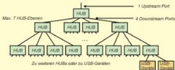
Bild 10: Zum Anschluß mehrerer Geräte an USB sind HUBs erforderlich. Sieben HUB-Ebenen sind zulässig. An ein Downstream-Port kann entweder ein HUB oder ein USB-Gerät angeschlossen werden.
