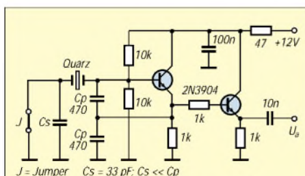
Nach Berechnung der Ziehkondensatoren und der Abschlußimpedanzen für ein CW- und SSB-Filter nach [7] hatte ich den Frequenzgang mit HF-Generator und HF-Millivoltmeter punktweise aufgenommen. Das CW-Filter zeigte einen brauchbaren Verlauf, leider konnte der Frequenzgang
