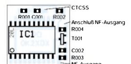
Bild 11: Bestückung der Zusatzplatine nach Bild 10; Bestückung auf der Leiterseite!
