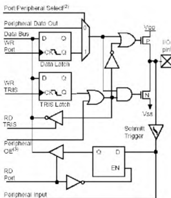
Bild 8: Blockdiagramm von RC<2:0> und RC<7:5>. (1) Die I/O-Pins besitzen Schutzdioden nach VDD und Masse. (2) Hier erfolgt die Umschaltung zwischen Portdaten und peripherem Output. (3) OE ist nur aktiviert, wenn (2) aktiv ist.
