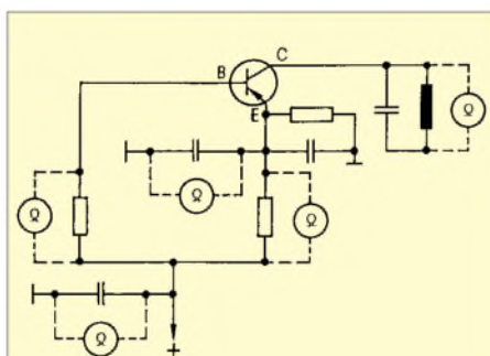
Bild 11: Widerstandsanalyse an einer ZF-Stufe
