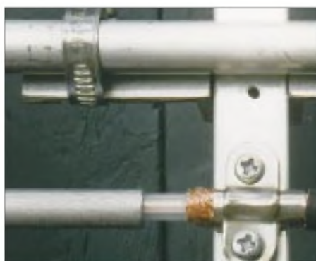
Bild 2: Befestigung des Speisekabels beim HB9QQ-Gammamatch Fotos: DL7HG
