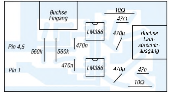
Bild 4: Bestückungsplan
