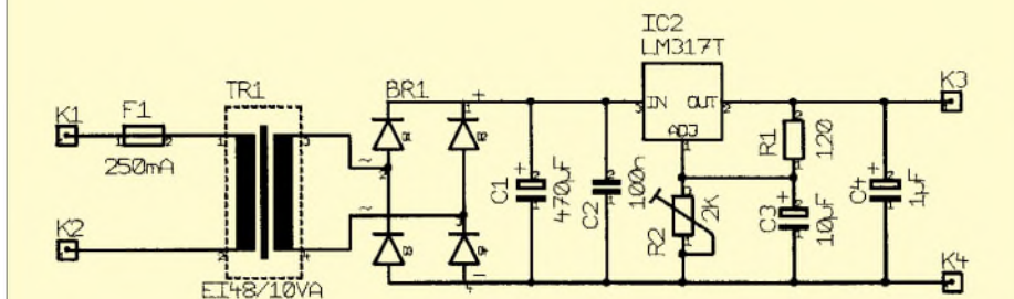
Bild 2: Festspannungserzeugung mit dem LM317
