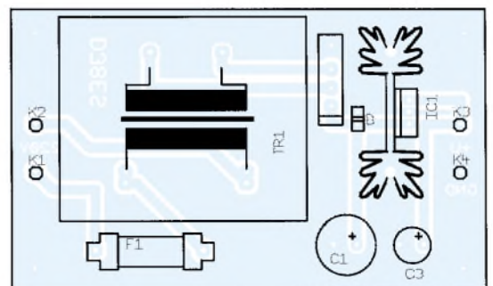
Bild 4: Bestückungsplan zu Bild 3
