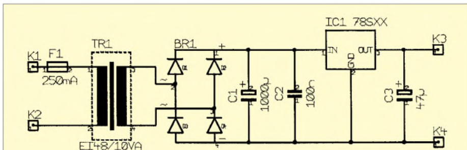
Bild 1: Festspannungserzeugung mit dem Reglertyp 78Sxx
