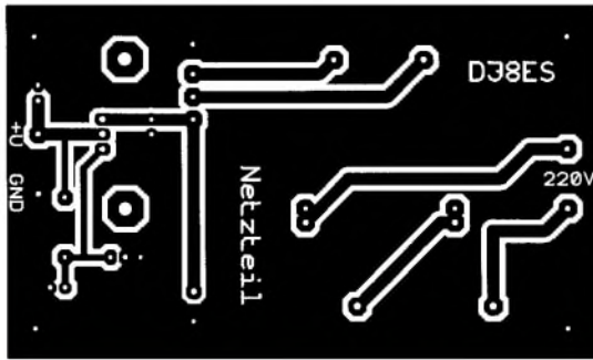
Bild 5: Platinenlayout zur Schaltung aus Bild 2
