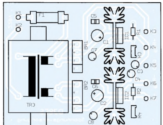
Bild 8: Platinenlayout zur Schaltung gemäß Bild 7
