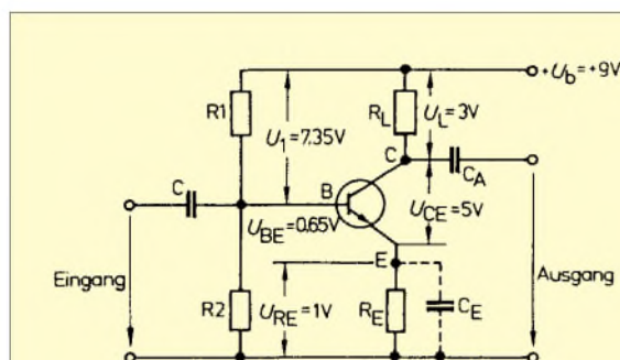
Bild 18: Spannungsverhältnisse an einer Transistor- Verstärkerstufe
