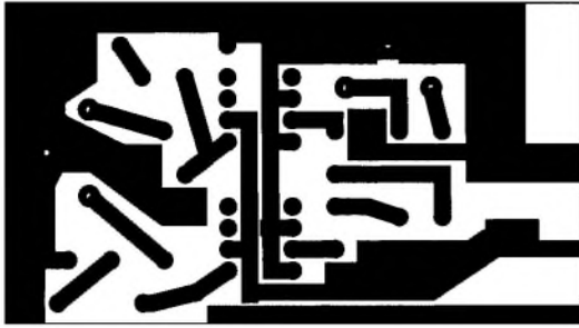
Bild 3: Platinenlayout
