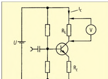
Bild 10: Indirekte Messung des Kollektorstroms
