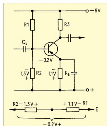
Bild 12: Entstehung der Basisspannung für einen Transistor
