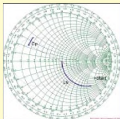
Bild 10: Anpassung mit Kondensatoren und Spulen, Startpunkt innerhalb des rechten Anpassungskreises
