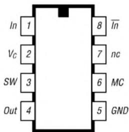
Bild 1: Pinbelegung
