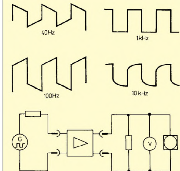
Bild 36: Verstärkerprüfung mit Rechteckspannung
