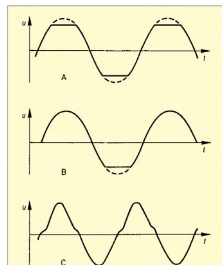
Bild 22: Kontrolle der Leistungsendstufe mit dem Oszilloskop:
