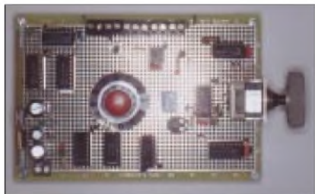
Bild 2: In der Mitte der Drehgeberplatine wählt der Stufenschalter die gewünschte Signalfolge aus.
