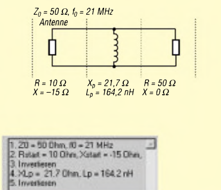
Bild 11: Vereinfachte Anpassungsschaltung mit einem Rest-SWR = 1,5
