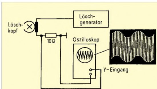
Bild 32: Überprüfung der Vormagnetisierung eines Recorders mit dem Oszilloskop
