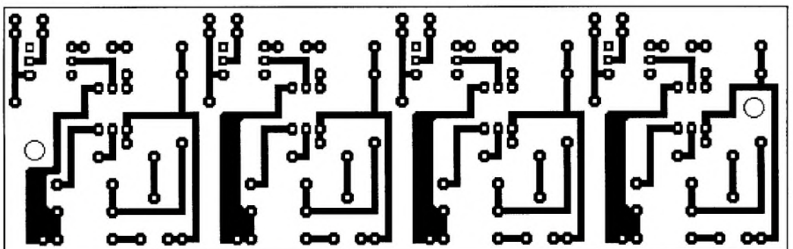
Bild 9: Layout Tiefentladungsschutz
