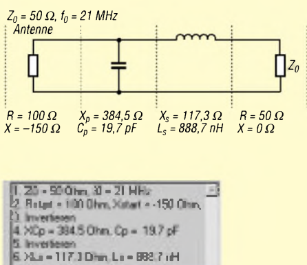
Bild 10: Anpassung mit Kondensatoren und Spulen, Startpunkt innerhalb des rechten Anpassungskreises
