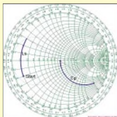
Bild 9: Anpassung mit Kondensatoren und Spulen, Startpunkt innerhalb des linken Anpassungskreises
