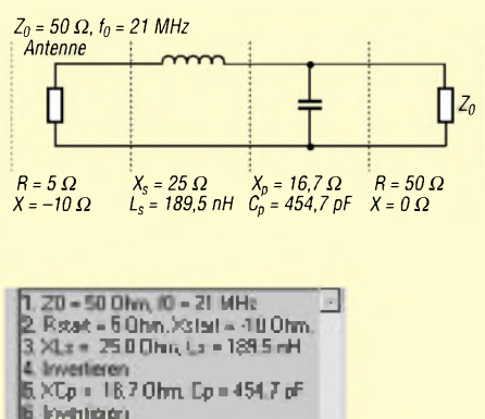
Bild 9: Anpassung mit Kondensatoren und Spulen, Startpunkt innerhalb des linken Anpassungskreises
