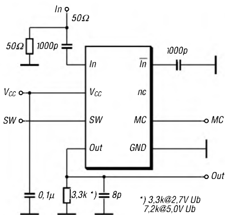
Bild 3: Typische Außenbeschaltung des SA 701
