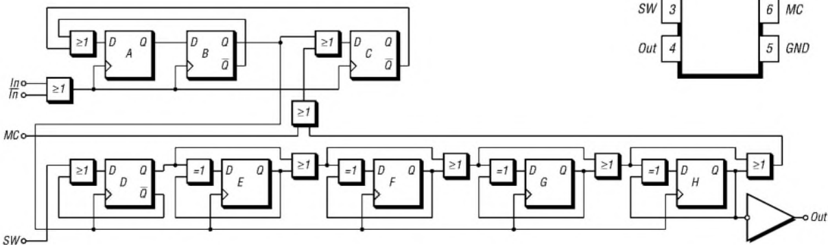
Bild 2: Blockschaltbild
