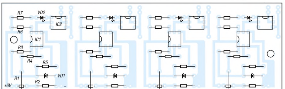
Bild 10: Bestückung Tiefentladungsschutz
