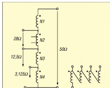
Bild 3: Aufbau des Anpaßübertragers. N1....N4: viermal 6 Windungen mit Kupferlackdraht 2 mm Durchmesser parallel auf Ringkern 61 mm Außendurchmesser, Permeabilität 200...300, z. B. Amidon FT 240-61. N2 hat Anzapfungen bei 1 und 5 Windungen.
