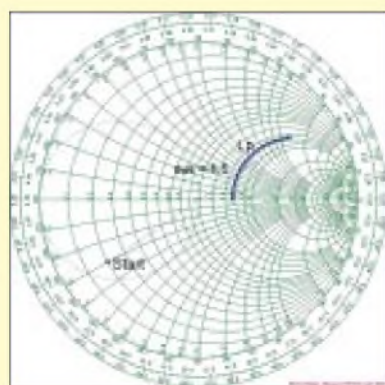
Bild 11: Vereinfachte Anpassungsschaltung mit einem Rest-SWR = 1,5
