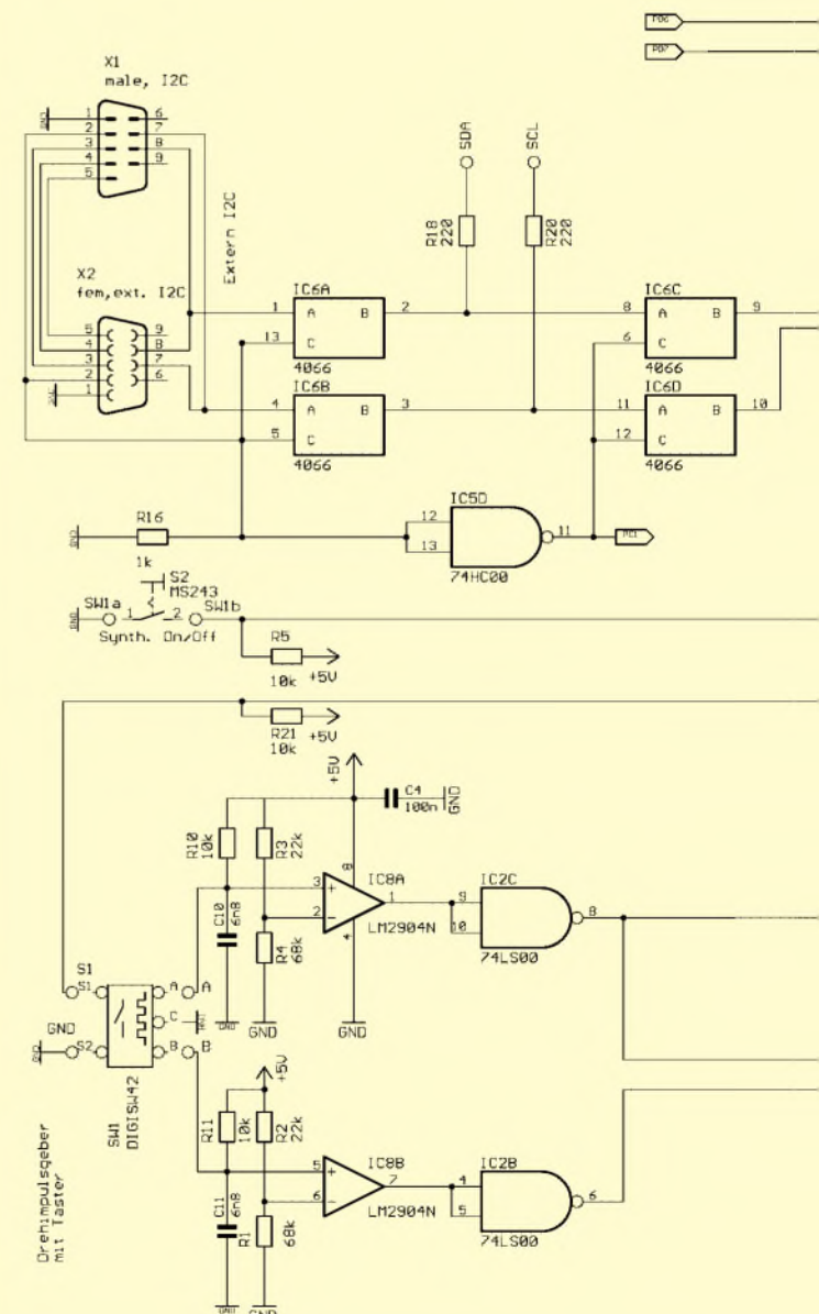
Bild 9: Schaltplan der Steuerungseinheit für den HF-Synthesizer
