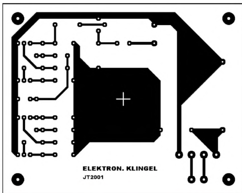
Bild 5: Platinen- layout der Klingel
