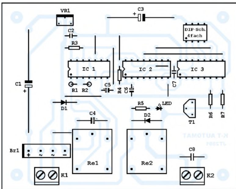
Bild 3: Bestück- ungsplan KT-Automat
