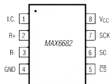
Bild 1: Pinbelegung (Draufsicht) des ICs im μMAX-Gehäuse
