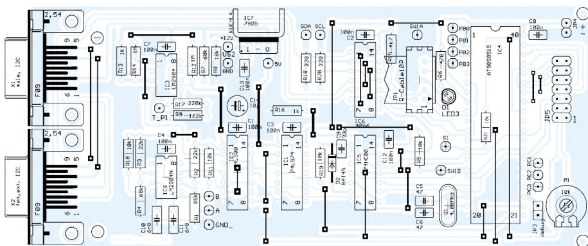
Bild 11: Bestückungsplan für die Steuerungseinheit des Synthesizers. Die Drahtbrücken sind zuerst zu bestücken!
