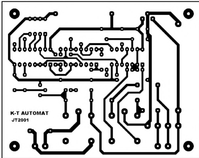
Bild 2: Platinen- layout KT-Automat
