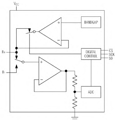
Bild 2: Blockschaftbild des MAX6682
