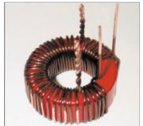
Bild 2: Zur Verdrahtung vorbereitete Spule. Den Kern besser vorm Wickeln mit etwa 1 mm dicker Isolierschicht versehen, um Erwärmung zu vermeiden. Fotos: DK5NOA
