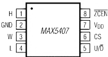
Bild 1: Pinbelegung (Draufsicht) des ICs im SOT-23-Gehäuse
