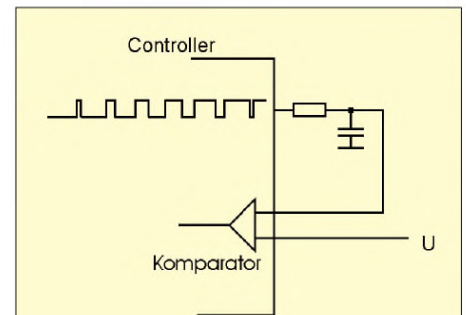
Bild 60: Mit einem Komparator läßt sich ein einfacher, aber sehr präziser AD-Wandler aufbauen.
