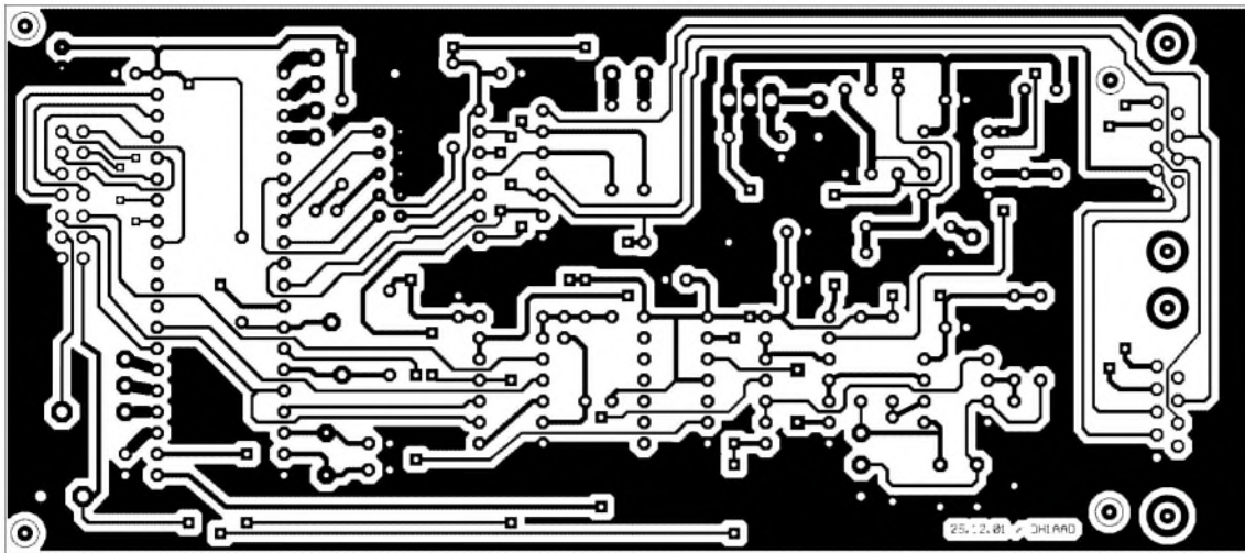
Bild 8: Leiterseite der Leiterplatte für die Steuerungs- einheit des Synthesizers
