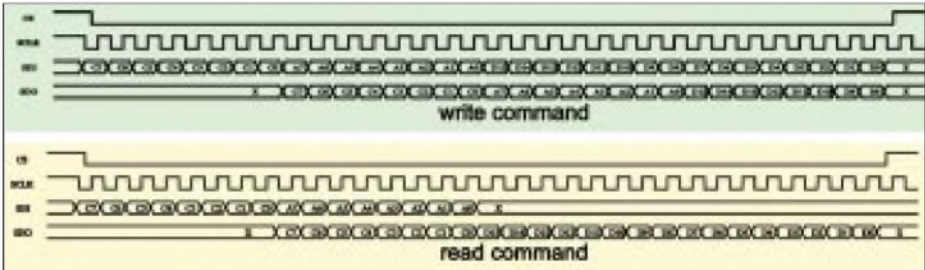
Bild 11: Das SPI-Interface entspricht dem SPI-Standard-Protokoll.
