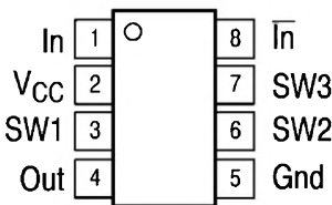
Bild 2: Pinbelegung (Draufsicht) des MC12080
