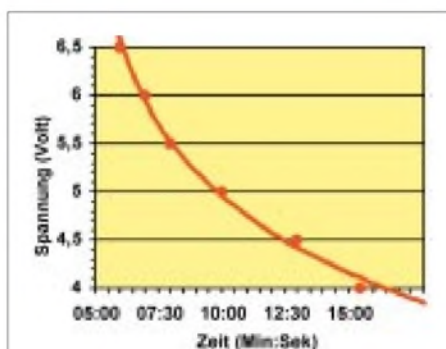
Bild 12: Theoretische zehninminütige Pause beim AT90xx2343 in Abhängigkeit von der Betriebsspannung bei 24 °C
