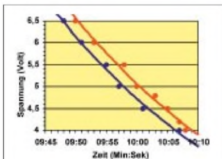
Bild 11: Theoretische zehninminütige Pause beim ATtiny12 in Abhängigkeit von der Betriebsspannung. Roter Graph: 24 °C, blauer Graph: 4 °C
