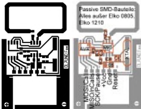
Bild 7: Platinenlayout und Bestückungsplan
