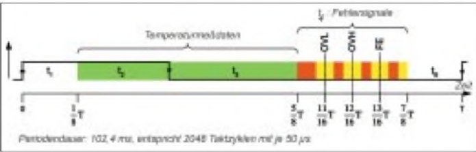
Bild 10: In das PWM-Signal sind zusätzliche Informationen eingeblenDET.
