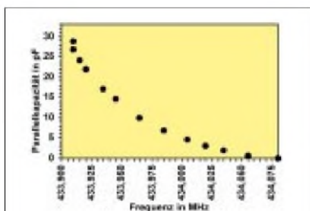
Bild 10: Frequenzeinstellung
