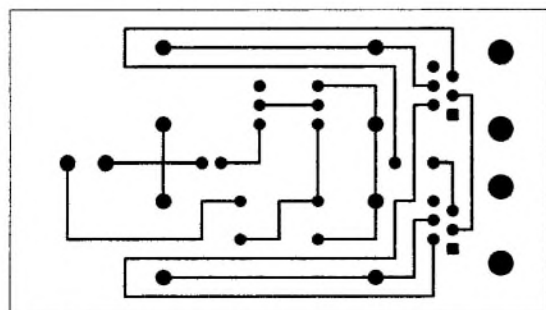
Bild 2: Platinenlayout
