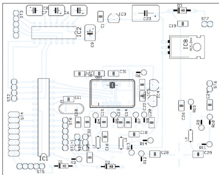
Bild 11: Bestückungsseite der Hauptplatine
