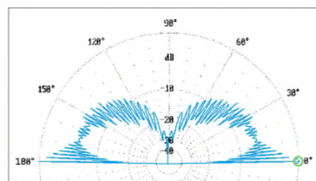
Bild 5: Elevationsdiagramm eines Vertikaldipols auf 435 MHz in 10 m Höhe über realem Grund mittlerer Leitfähigkeit; 0 dB \pm 7,59 dBi, Maximum bei 1,0°
