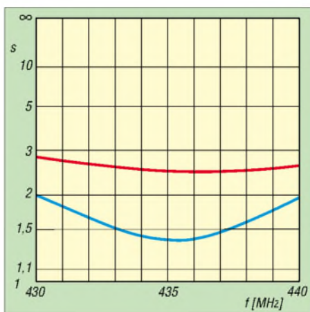
Bild 6: Mit EZNEC simuliertes SWV der FK-Antenne bei Speisung mit 50 Ω (rot) bzw. 28 Ω (blau)
