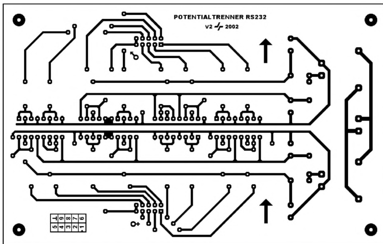
Bild 3: Platinenlayout
