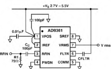
Bild 5: Grundbeschaltung Massereferenzmodus
