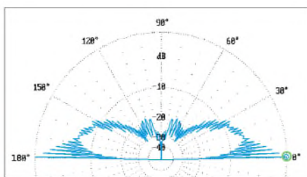
Bild 4: Elevationsdiagramm der FK-Antenne auf 435 MHz in 10 m Höhe über realem Grund mittlerer Leitfähigkeit; 0 dB \pm 9,61 dBi, Maximum bei 1,0°
