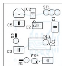
Bild 8: Bestückung der Meßkopfplatine; nicht masseführende Löcher der Massefläche sind freizusenken.
