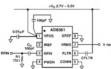
Bild 6: Grundbeschaltung Internereferenzmodus
