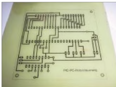
Der Toner läßt sich problemlos auf die Platine übertragen und ist ätzfest.
