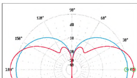
Bild 3: Freiraum-Elevationsdiagramm der FK-Antenne (rot) im Vergleich zu einem Vertikaldipol (blau); 0 dB \pm 2,14 dBi; Maximum 4,16 dBi bei 0°, also 2,02 dBd
