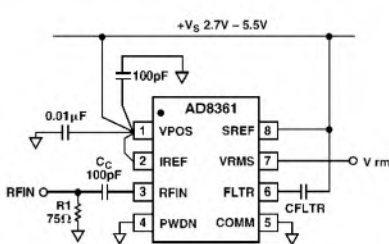
Bild 7: Grundbeschaltung Betriebs-spannungsreferenzmodus
