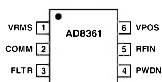
Bild 1: Pinbelegung (Draufsicht) des AD8361 im micro-SOIC- und SOT-23-6L-Gehäuse
