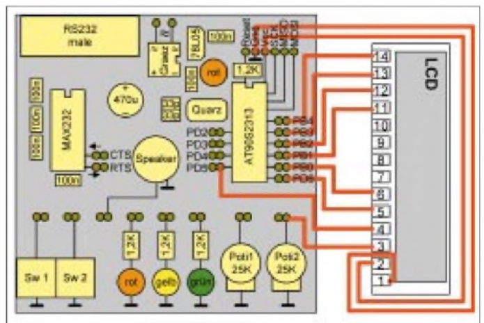
Bild 35: Verdrahtung
