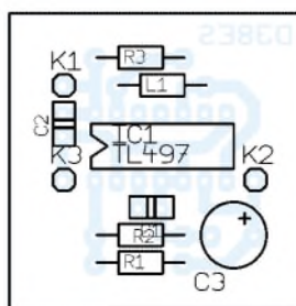
Bild 4: Bestückungsplan
