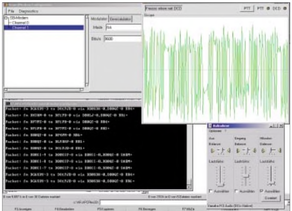
Bild 8: Soundmodem im Testbetrieb, hier in FSK mit 9600 Baud auf dem 70-cm-Benutzerzugang von DB0QT
