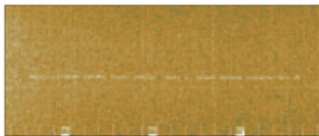
Eines der ersten auf dem britischen 73-kHz-Band übertragenen Signale in extrem langsamer Telegrafie (QRSS). Die Übertragung dieses Signals über eine Strecke von 392 km benötigte mehr als drei Stunden
