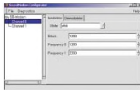
Bild 6: Das AFSK-Einstellmenü schlägt bereits die gebräuchlichen Kenntöne vor.
