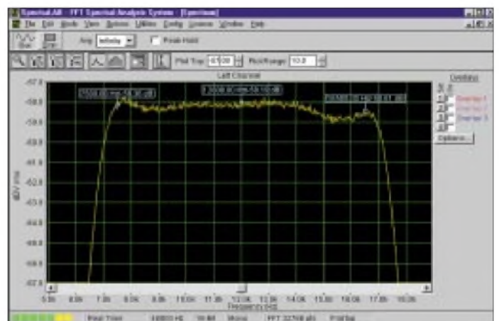
Bild 11: Filterkurve über alles an einem umgebauten AR-7030, dargestellt mit der Analysesoftware SpectraLab [10]
