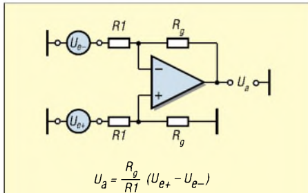
Bild 8: Der Subtrahierer. Am Ausgang erscheint die genaue Differenz der Eingangsspannungen, wenn alle vier Widerstände gleich groß sind.
