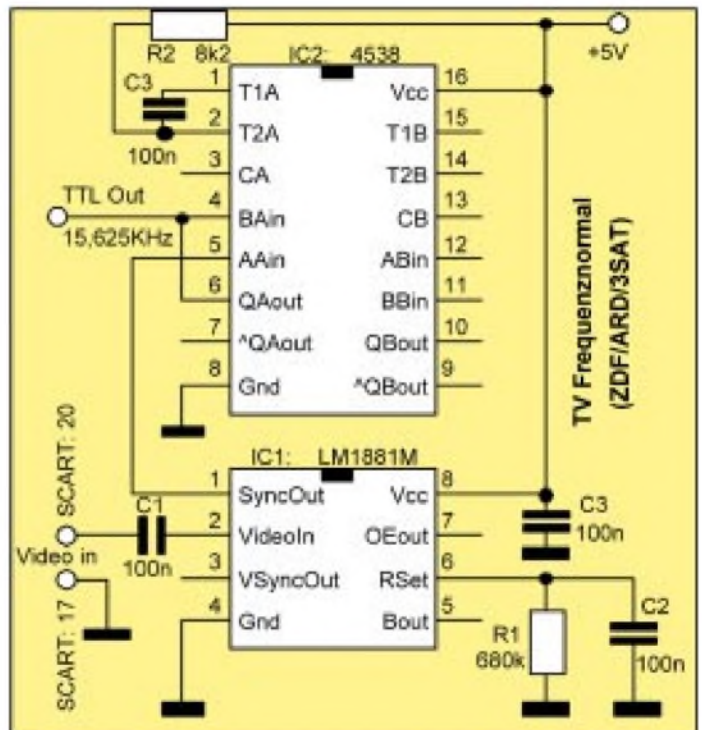
Bild 44: Das einfache Frequenznormal
