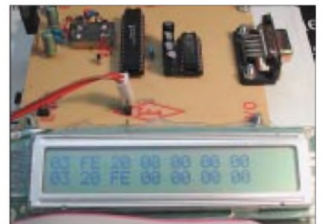
Bild 2: Ansicht des Versuchsaufbaus. Gut sichtbar der Quarzoszillator, er liegt auf dem Rücken und ist fliegend verdrahtet.
