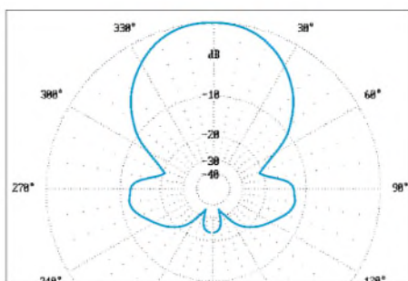
Bild 16: H-Diagramm der 5-Element-Yagi bei 50,15 MHz; 0-dB-Ring \hat{=} 8,62 dBd
