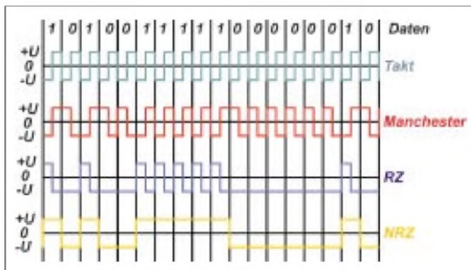
Bild 2: Für die optische Übertragung eignen sich insbesondere solche Verfahren ohne Gleichspannungsanteil im Signal, wie zum Beispiel der Manchestercode.
