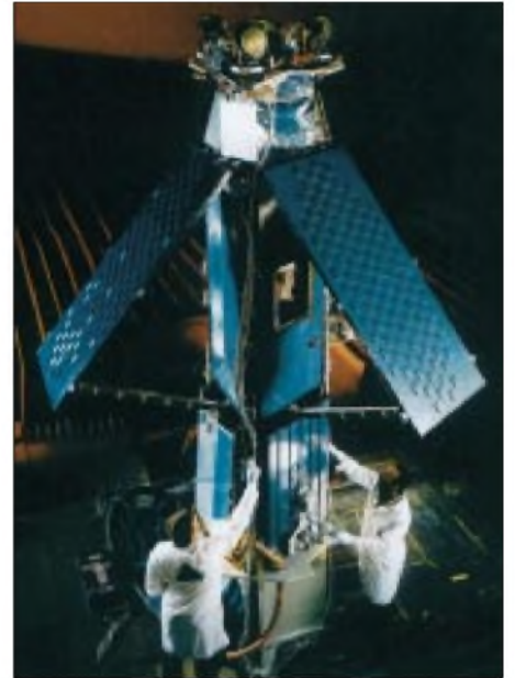
Bild 2: Iridium-Satellit in der Montagehalle Foto: Motorola
