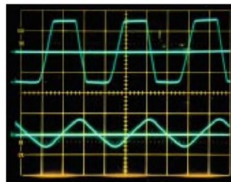
Bild 16: Oszillogramm des Multivibrators bei 150 kHz: Die Impulsflanken benötigen eine Zeit von über 1 \mu\text{s} . C = 1\text{ nF} , R = 10\text{ k}\Omega , R_2 = 6,8\text{ k}\Omega , R_m = 100\text{ k}\Omega . Der untere Kurvenzug zeigt U_e ; y = 2\text{ V/skt} , x = 2\text{ }\mu\text{s/skt} . Der obere Kurvenzug zeigt U_a ; y = 5\text{ V/skt} , x = 2\text{ }\mu\text{s/skt} .
