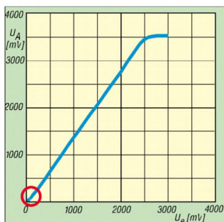
Bild 4: Angezeigte Gleichspannung in Abhängigkeit von der HF-Eingangsspannung; zwischen 100 und 2000 mV Eingangsspannung ist die Anzeige annähernd linear.
