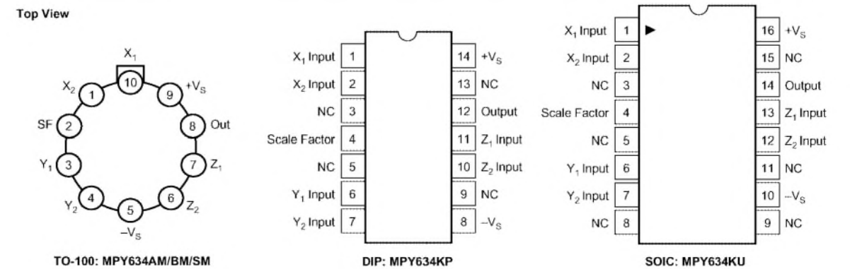
Bild 1: Pinbelegung (Draufsicht) der drei verschiedenen Gehäusevarianten des MPY634
