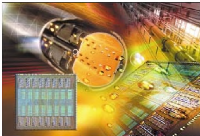
Am CERN in der Nähe von Genf (Schweiz) entsteht der weltgrößte atomare Teilchenbeschleuniger LHC.
