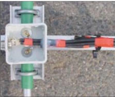
Bild 2: Anpassleitung mit RG59-Kabeln in bzw. neben der Strahlerdose
