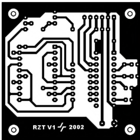
Bild 2: Platinenlayout des RZT
