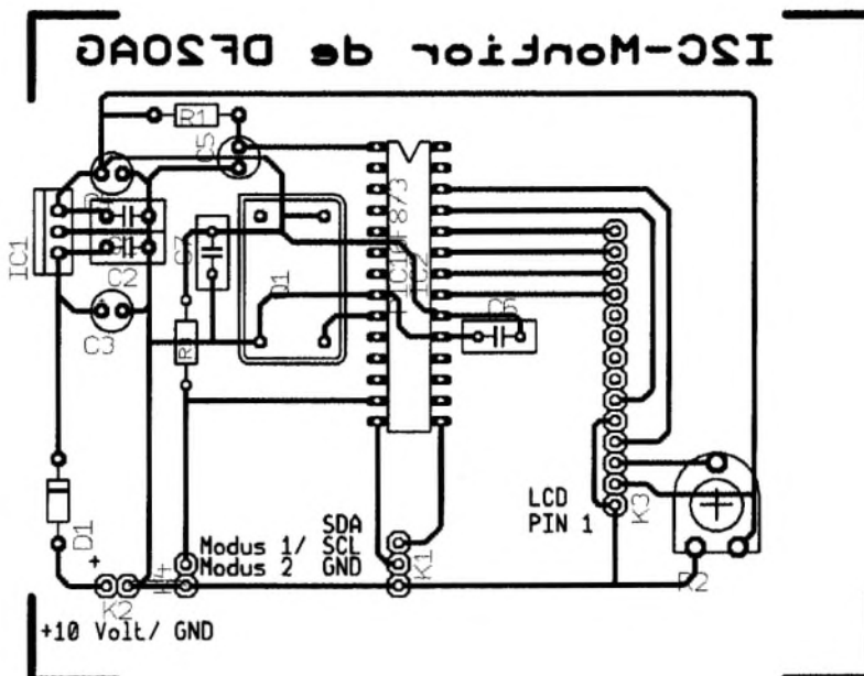
Bild 4: Bestückungsplan
