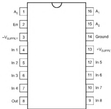
Bild 2: Pinbelegung (Draufsicht)
