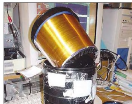
DF6NM's 1-H-Jogurtbecher-Spule für 8970 Hz
