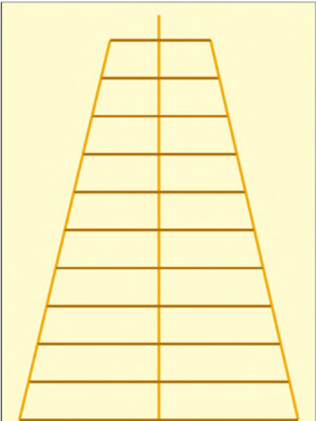
Bild 3: Hilfskonstruktion für den Bau des Widerstandskegels (Hilfsstreben orange, Trägringe braun)
