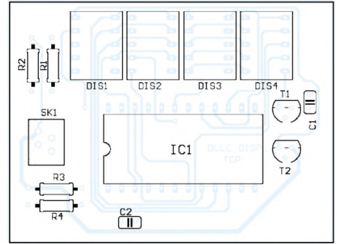
Bild 5: Als Steckverbinder wird der Typ MICS 4polig eingesetzt.
