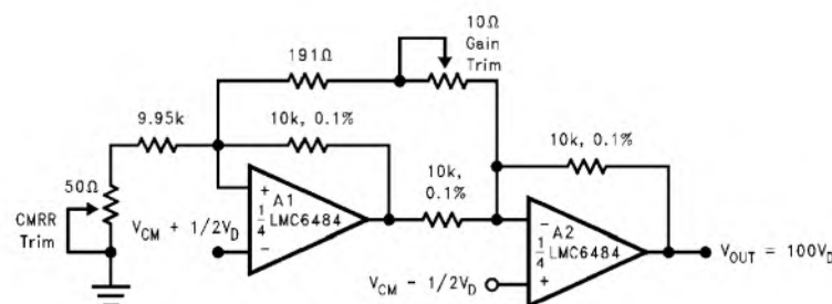
Bild 5: Low-Power-Instrumentenverstärker
