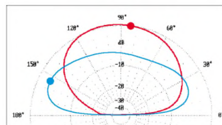
Bild 5: Vertikaldiagramm des Slopers über realem Grund mittlerer Leitfähigkeit ohne (blau) und mit (rot) Beam auf dem Mast, 0 dBd = +1,0 dBd
