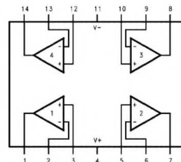
Bild 2: Pinbelegung
