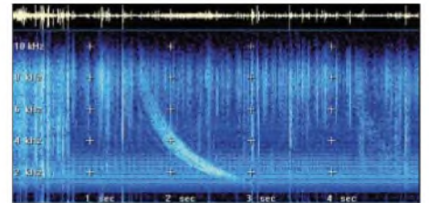
Bild 8: Spektrogramm eines Multiple-Path-Whistlers
