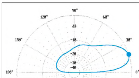
Bild 7: Elevationsdiagramm des 30-m-V-Dipols ( 0 \text{ dB} = 1,7 \text{ dBd} bei 18^\circ )
