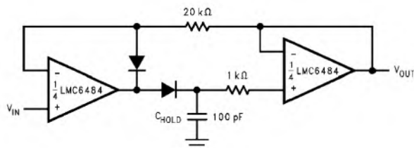
Bild 6: Low-Voltage-Spitzendetektor
