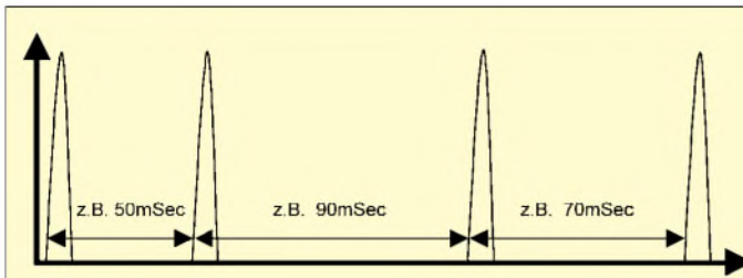
Bild 74: PIM-Übertragung der Werte 50, 90 und 70
