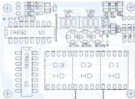
Bild 9: Bestückungsplan DVM
