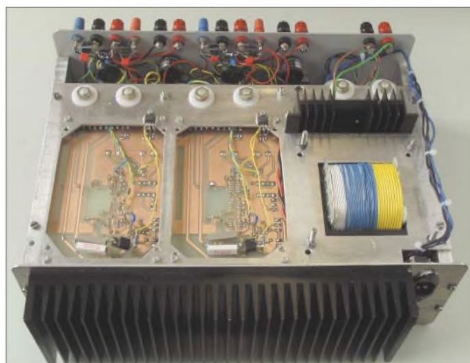
Bild 12: Ansicht des Musteraufbaus von der Unterseite
