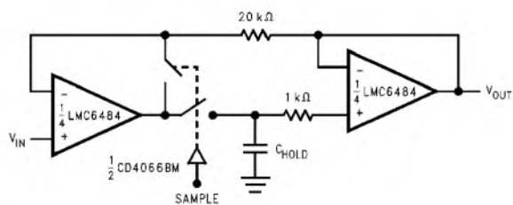
Bild 7: Rai-to-Rail-Sample-&-Hold-Schaltung
