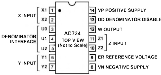
Bild 2: Pinbelegung
