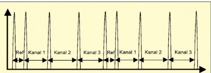
Bild 75: Übertragung mehrerer Kanäle per Pulsintervallmodulation
