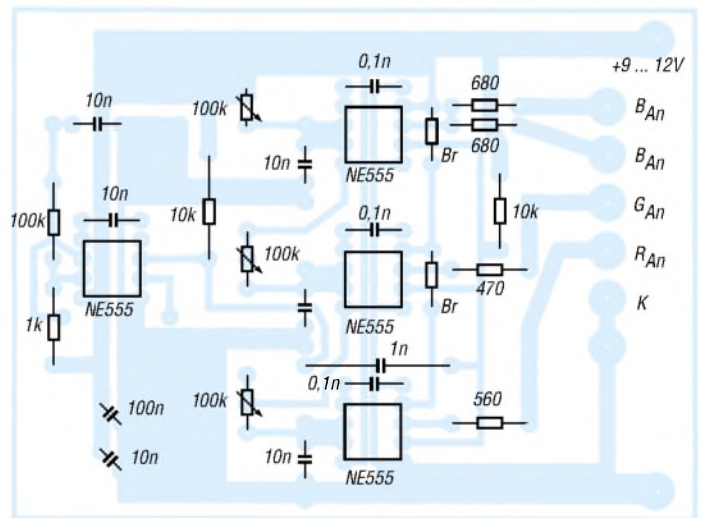
Bild 6: Bestückungsplan zur Platine aus Bild 5
