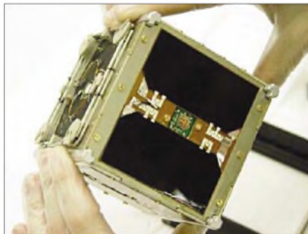
Ein CubeSat in geöffnetem Zustand in den Händen eines Technikers. Foto: AMSAT-USA
