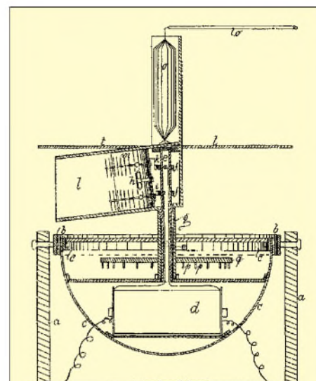
Bild 2: Die Hauptzeichnung von C. Hülsmeyers „Radar“-Patent. Unten eine kardanische Aufhängung abc. Darüber montiert ist der Kasten I mit der Sendeanenne und die Empfangsanenne o. Die Anordnung ist um den Zapfen e drehbar. aus Patent DE 165 546
