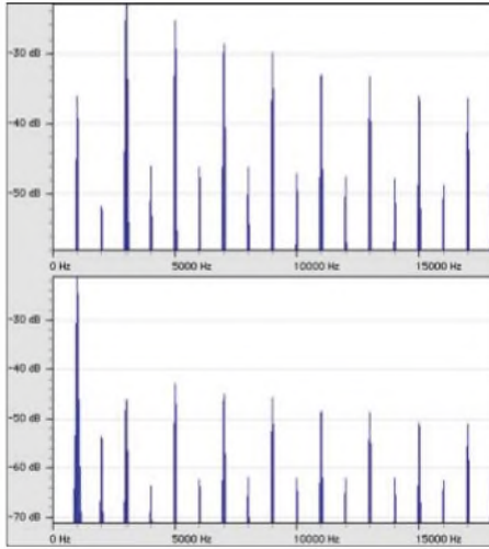
Bild 14: Harmonische Verzerrungen bei einem Halbleiterverzerrer für Gitarren bei unterschiedlichen Aussteuerungen
