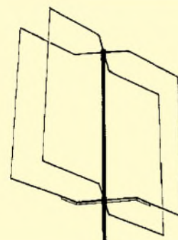
Bild 9: Diese Antenne nach HB9CV ist robust und kompakt. Der Reflektor-Direktor-Abstand darf bis 0,05 \lambda reduziert werden!
