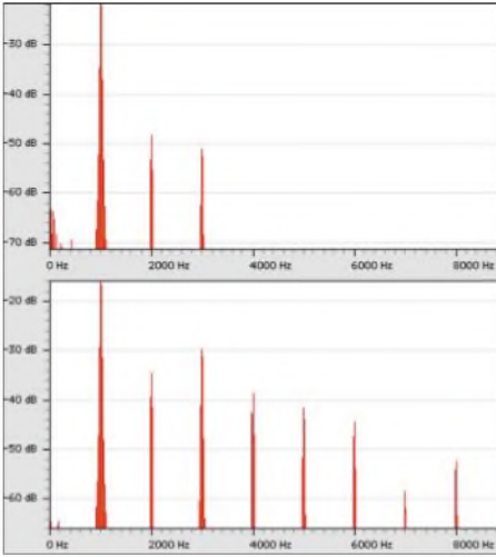
Bild 12: Harmonische Verzerrungen in einem Röhrenverzerrer für Gitarren bei unterschiedlichen Ansteuerungen
