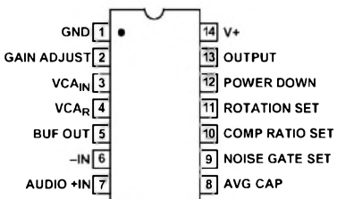
Bild 2: Pinbelegung
