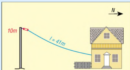
Bild 1: Die Fuchs-Antenne wird über einen Antennenkoppler direkt an den Senderausgang angeschlossen.
