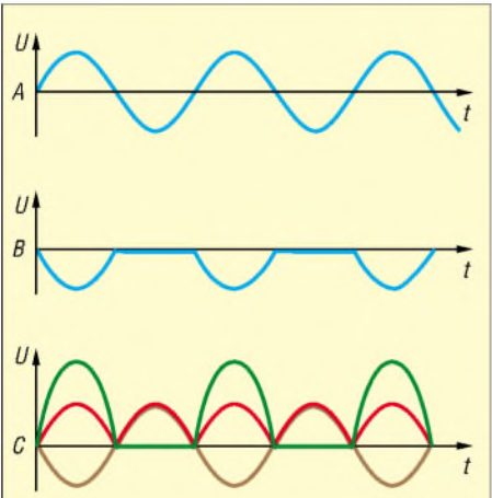
Bild 58: Zeitlicher Verlauf der Spannungen am Präzisions-Zweiweggleichrichter aus Bild 56 ohne Kondensator C A – Eingangsspannung U_a B – Signal an Anode von D2 C – Ausgangsspannung U_a an OpV2 (grün Signal aus B zweifach verstärkt/invertiert, braun U_a einfach verstärkt, rot resultierende U_a )
