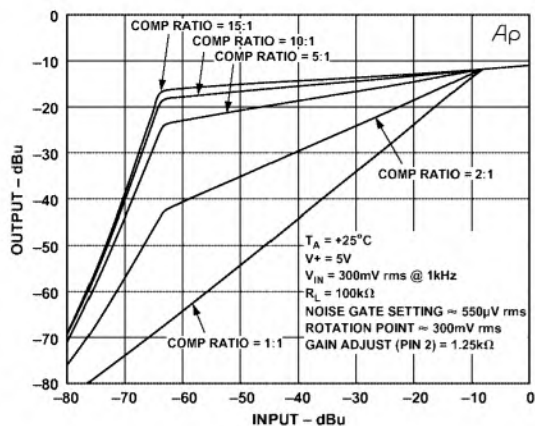
Bild 3: Ausgangspegel als Funktion des Eingangspegels in Abhängigkeit vom Kompressionsverhältnis
