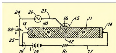
Bild 10: Die 1951 erstveröffentlichte Zeichnung eines Transistorverstärkers sieht recht unspektakulär aus.
