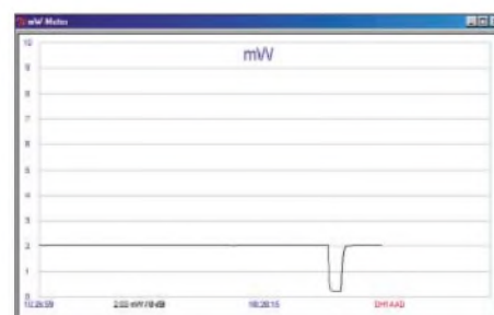
Bild 10: Bei Kontrollaufgaben bietet sich die zeitliche Darstellung der Leistung auf dem PC an.
