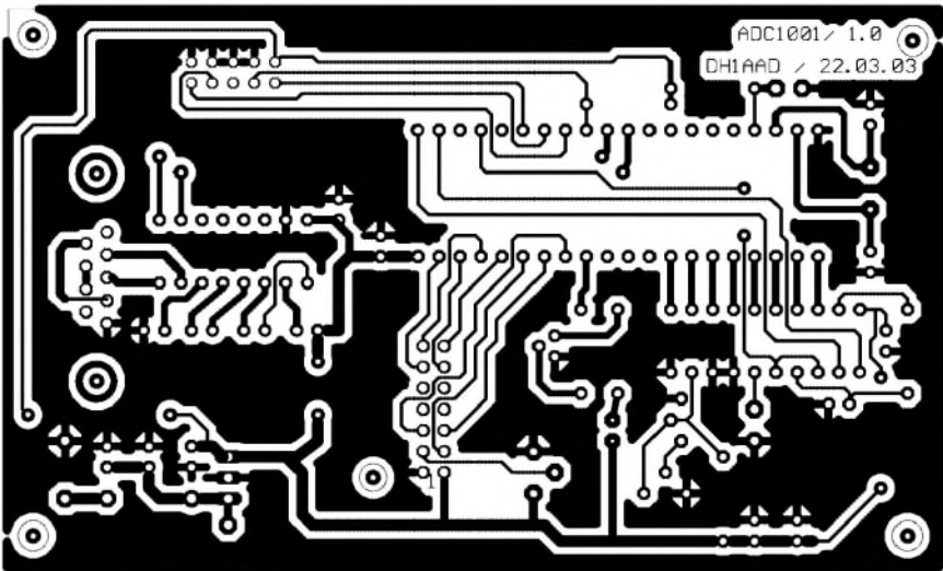
Bild 11: Layout der Controllerplatine (112 mm x 68 mm)
