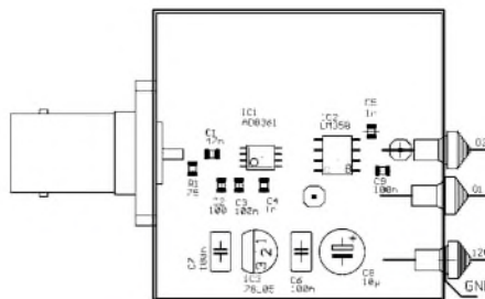
Bild 5: Layout des Messwandlers mit dem AD8361. Die Abmessungen der Platine betragen 35 mm x 35 mm.
