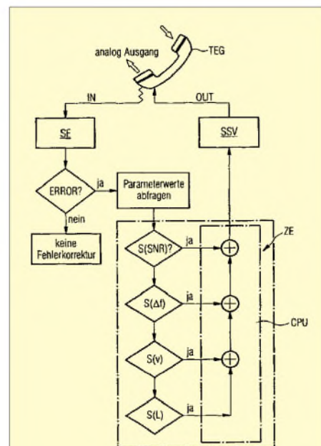
Bild 12: Ein modernes MMI-Patent von Siemens beschreibt eine technische Sprachein- und -ausgabe. Dem Benutzer werden einfache Anweisungen gegeben, sodass seine Spracheingabe besser erkannt werden kann.
