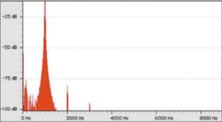
Bild 11: Harmonische Verzerrungen in einem Transistorendverstärker
