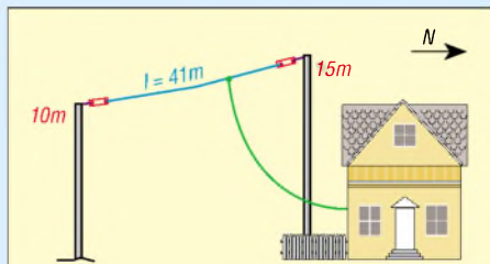
Bild 2: Die Windom-Antenne hat in der Urform nach VS1AA nur eine eindrahthige Speiseleitung.
