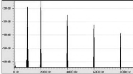
Bild 15: Klangspektrum bei asymmetrischer Verstärkung
