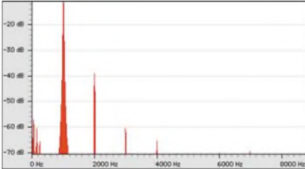
Bild 13: Harmonische Verzerrungen in einem Gitarrenverstärker mit Röhrenvorstufe
