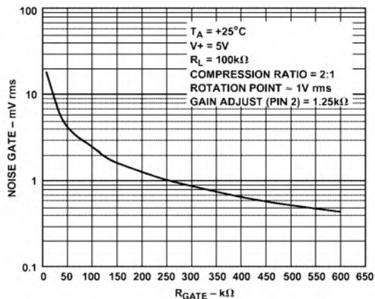
Bild 4: Rauschsperre als Funktion des Widerstands R_{GATE} (Anschluss 9 an U_B )
