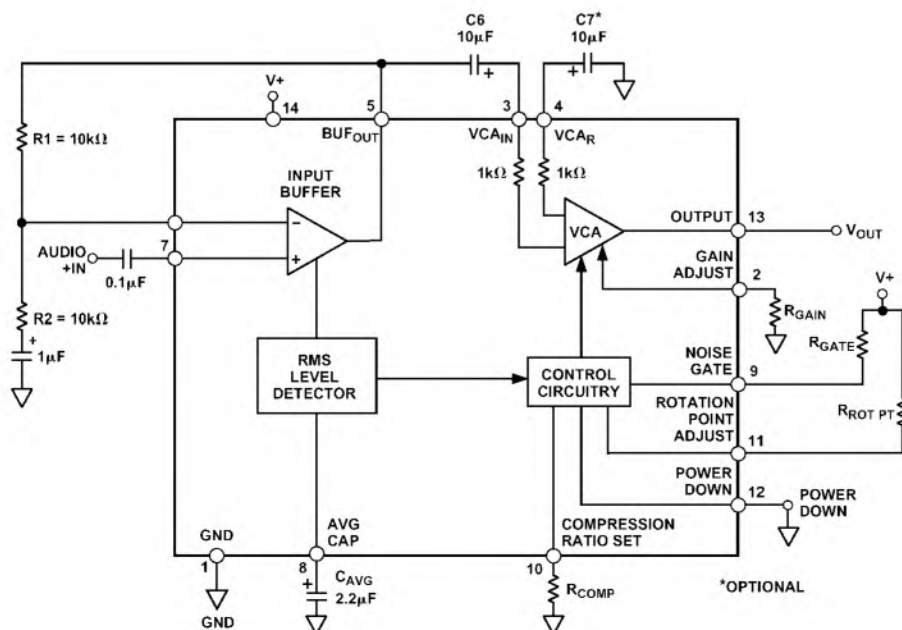
Bild 7: Typische Beschaltung
