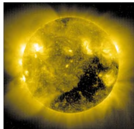
Bild 2: Ein transäquatoriales koronales Mammutloch in geoaktiver Position am 11. Mai 2003. Als Folge waren die DX-Bedingungen katastrophal.
