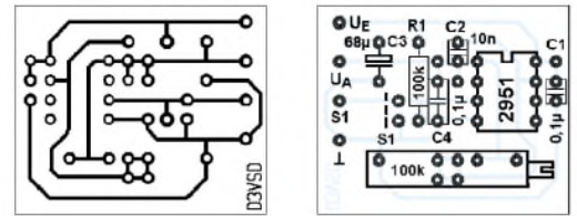
Bild 11: Layout und Bestückung der Platinenvariante 3 – D3VSD
