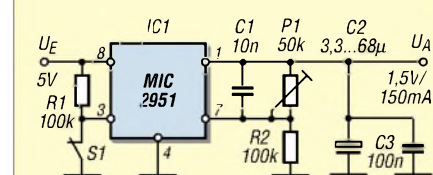
Bild 3: Die Variante 2 (D2VSD) erlaubt die Abschaltung der 1,5-V-Ausgangsspannung.
