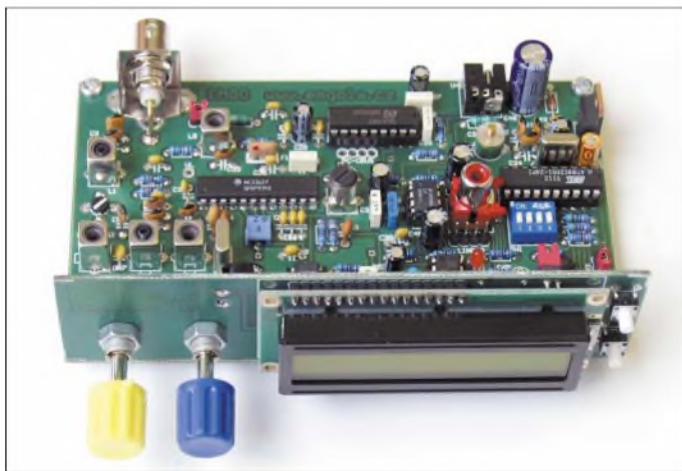
Bild 1: Die Grundplatine ist nur 137 mm × 84 mm groß und dient als Montagebasis für die 137 mm × 37 mm messende Anzeige- und Bedienplatine. Durch den kompakten Aufbau entfallen fast alle Verdrahtungsarbeiten.
