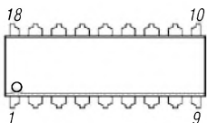
Bild 2: Pinbelegung
