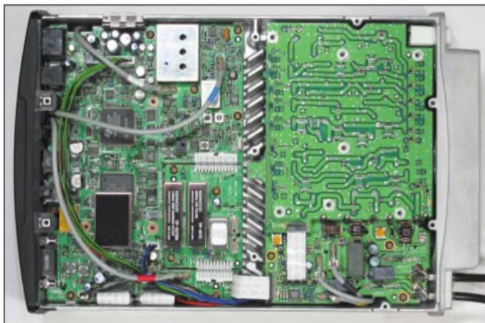
Bild 9: Blick von oben in den TS-480 (Schirmbleche abgenommen). Links unten sind hier zwei optionale ZF-Filter (1,8 kHz für SSB schmal sowie 500 Hz für CW) eingebaut; rechts daneben der Platz für einen TCXO (temperaturkompensierter Referenzoszillator). Interessant die mittigen Kühlrippen
