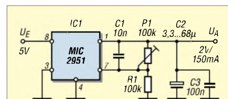
Bild 2: In der Variante 1 (D2VR) kann man eine Spannung von 1,5 bis 2 V einstellen.
