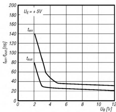
Bild 5: Ein- und Ausschalzeit des Schalters in Abhängigkeit von der Betriebsspannung
