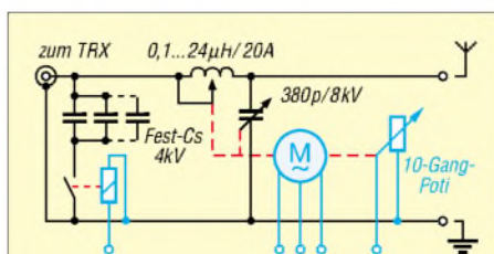
Bild 2: Schaltbild des vereinfachten Antennentuners einschließlich Steuerungselementen (blau) und mechanischer Kopplung (rot)
