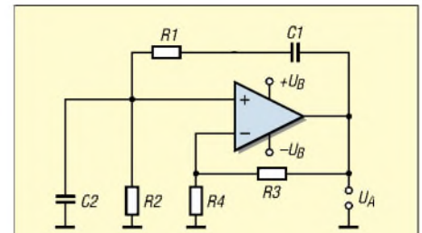
Bild 2: Prinzipschaltung eines Sinusoszillators mit Wien-Brücke
