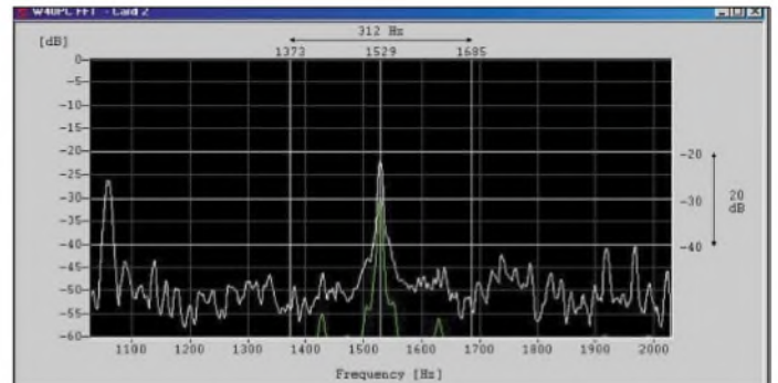
Bild 5: So sollte der Träger eines fabrikneuen Gerätes aussehen, wenn sich die Ionosphäre im Normalzustand befindet.
