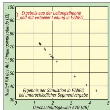
Bild 6: Realteil RA des Antenneneingangswiderstands in \Omega , aufgetragen über dem Durchschnittsgewinn AVG. Die Zahlenwerte stammen aus einer Dipolsimulation mit angeschlossener Zweidrahtleitung, siehe Tabelle 1. Eine verbindende Kurve lässt sich ohne Probleme auf den Wert bei \text{AVG} = 0 \text{ dB} extrapolieren und erreicht dort den wahren Wert RA = 94 \Omega .
