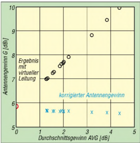
Bild: 7 Antennengewinn G in dBi und korrigierter Antennengewinn G_{korr} = G - AVG , aufgetragen über dem Durchschnittsgewinn AVG. Die Zahlenwerte stammen aus einer Dipolsimulation mit angeschlossener Zweidrahtleitung, siehe Tabelle1. Werden die Punkte durch Geraden verbunden, so lässt sich der gesuchte Gewinnwert bei AVG = 0\text{ dB} zu G = 5,8\text{ dBi} bestimmen.
