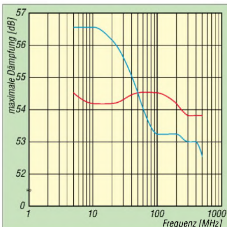
Bild 6: Die maximale erreichbare Dämpfung erreicht im Frequenzbereich von 5 bis 500 MHz je nach verwendeter Pin-Diode Werte zwischen 52,6 und 56,6 dB. Eine BA479 (rote Kennlinie) schnitt in punkto Linearität gegenüber einer BA595 (blaue Kennlinie) besser ab.
