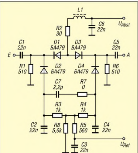
Bild 2: Vier Pin-Dioden gestatten im Abschwächer die kontinuierliche Einstellung der Dämpfung.
