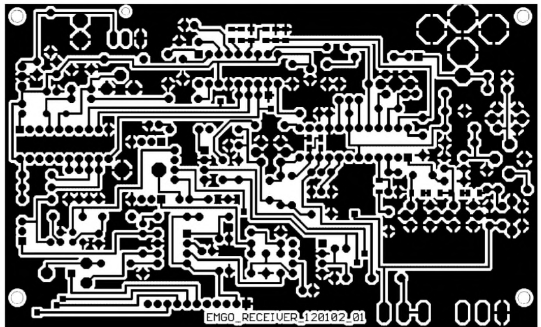
Bild 6: Leiterseite der doppelt ka- schierten Hauptplatine
