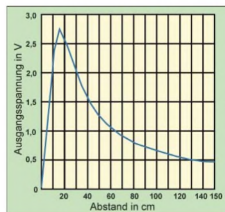
Bild 1: Zwischen Distanz zum Messobjekt und Ausgangsspannung des Sensors besteht ein nichtlinearer Zusammenhang.
