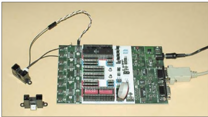
Bild 3: Der Sensor arbeitet mit einer positionsempfindlichen Fotodiode nach dem Triangulationsprinzip.
