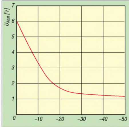
Bild 3: Dämpfungen größer als 20 dB sind erst bei Abstimmspannungen unter 1,76 V erreichbar, sodass der Hauptnutzungsbe- reich zwischen 1 und 2 V liegt. Die erfordert eine möglichst genau einstellbare Spannungsquelle mit Anzeigeinstrument oder die Ansteuerung per Software.
