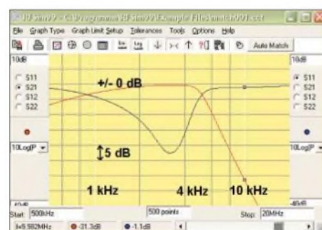
Bild 4: Frequenzgang der Schaltung nach Bild 3 (Y-Schritt = 5 dB)
