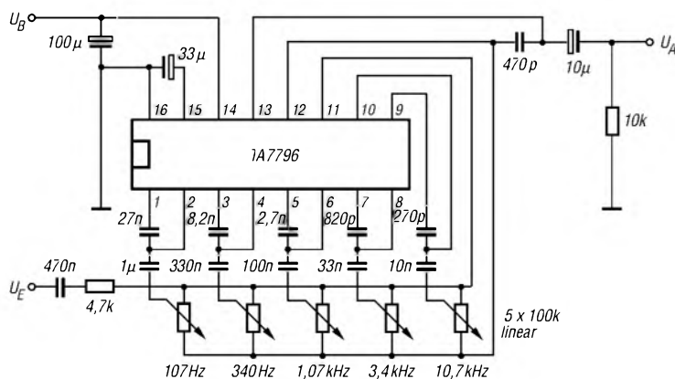
Bild 6: Nutzung des TA7796 zur Beeinflussung eines NF-Signals im Bereich von 50 Hz bis 2 kHz
