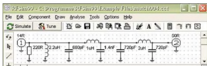
Bild 3: Der LC-Impedanzwandler in Kombination mit einem dreipoligen Tschebyscheff-Tiefpass
