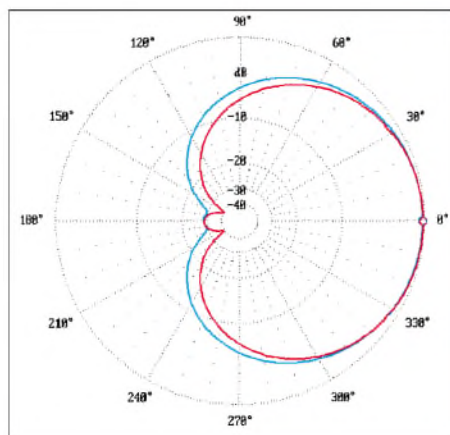
Bild 5: Azimut-(-E)-Diagramm (rot) der 12,5-Ω-Yagi (bei horizontaler Polarisation) und Elevations-(-H)-Diagramm (blau), 0 dB = 4,63 dBd
