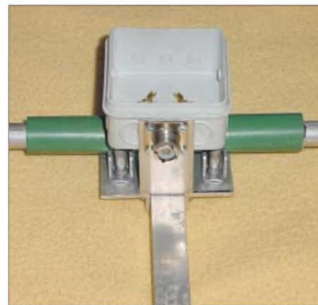
Bild 8: Aluminium-Winkel zum Erden der Koaxialbuchse
