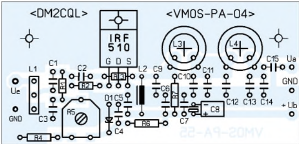
Bild 6: Bstückerungsplan der VMOS-PA
