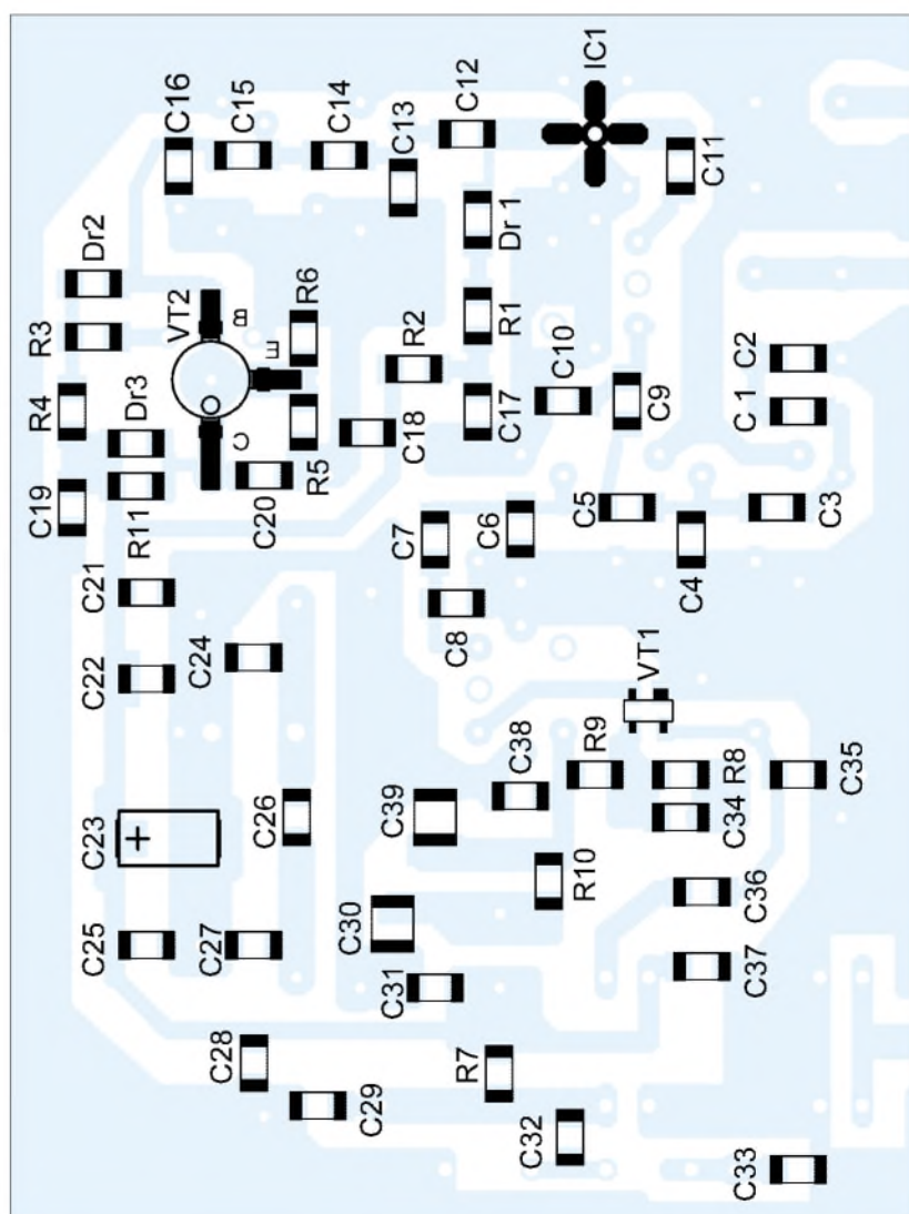
Bild 5: Bestückungsplan der Platine, M 2:1 dargestellt, auf die Leiterseite gesehen
