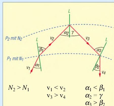
Bild 3: Prinzipielle Darstellung zweier Potenzialflächen – im Schnitt – mit einfallendem Funkstrahl. Die Flächen können in der Realität z.B. 200 km voneinander entfernt sein. Dabei wird die Krümmung des Funkstrahls der Übersichtlichkeit wegen nicht berücksichtigt.
