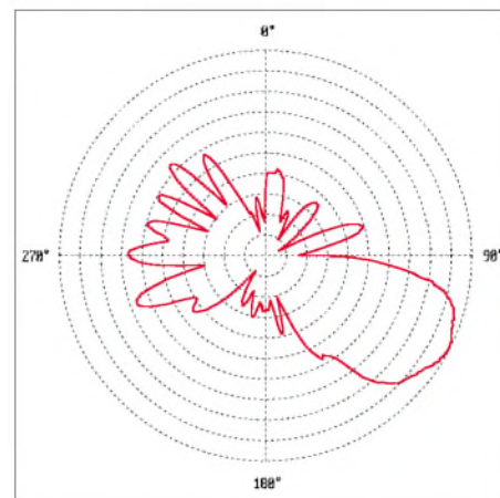
Bild 12: Azimutales Strahlungsdiagramm der 70-cm-Antenne von DJ1YQ im dB-linearen Maßstab, 3 dB pro Teilstich
