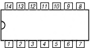
Bild 2: Pinbelegung (DIP14)
