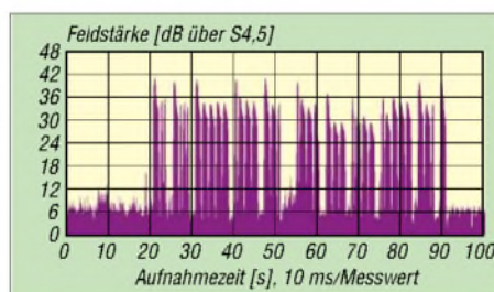
Bild 11: 70-cm-Bakensignal von DB0JG in JO31GT bei hoher Sendeleistung
