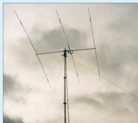
Bild 2: Hoch angebrachte Richtantennen, hier ein Mosley-Beam TA-33JRN für 20, 15 und 10 m, sorgen für eine flache Abstrahlung kurzer Wellen. Foto: DL2RD
