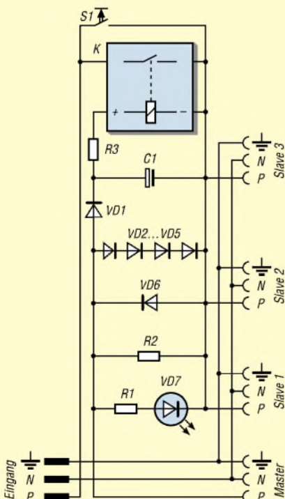
Bild 4: Stromlaufplan des Stromföhlers der Master-Slave-Schaltung mit dem Starttaster
