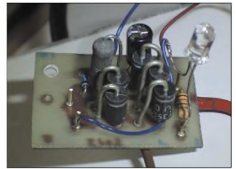
Bild 5: Stromföhlcr auf einer kleinen geätzten Leiterplatte Fotos: DL7JET
