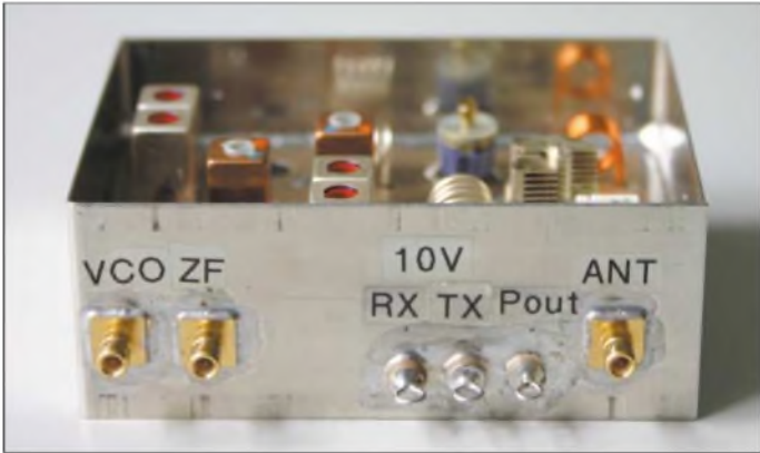
Bild 2: Das Frontend, hier ein Prototyp, findet in einem Weißblechgehäuse mit den Abmessungen (B \times H \times T) 74 mm \times 28 mm \times 55 mm Platz. Fotos: DF5SL
