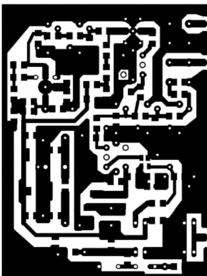
Bild 3: Layout der Platine, M 1:1, Abmessungen 72 x 54 mm²
