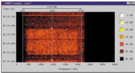
HFDL-System auf 18,117 MHz mit einer Baudrate von 1k8
