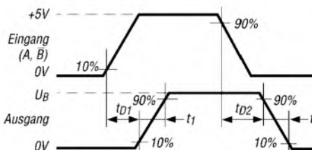
Bild 6: Zeitverhalten des Ein- und Ausgangssignals
