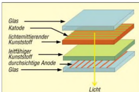
Bild 2: Eine OLED besteht aus mehreren dünnen halbleitenden Kunststoffschichten zwischen Glaträgern.
