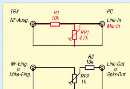
Bild 2: Verbindung zwischen Transceiver und Soundkarte
