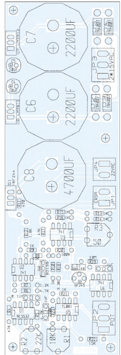
Bild 8: Bestückung der Platine für die Temperaturregelung
