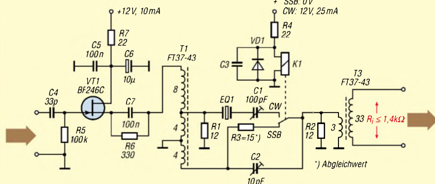
Bild 4: Quarzfilter mit hochohmigem Eingang und höherer Aufwärtstransformation. Einfügungsdämpfung = 0 dB; sonst wie bei Bild 1.
