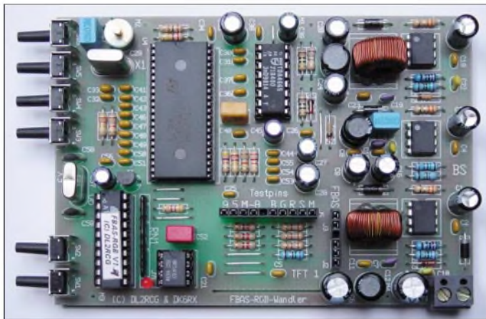
Bild 1: Die komplett bestückte Umsetzerplatine lässt sich über Lötstifte direkt hinter dem TFT-LC-Display befestigen.
