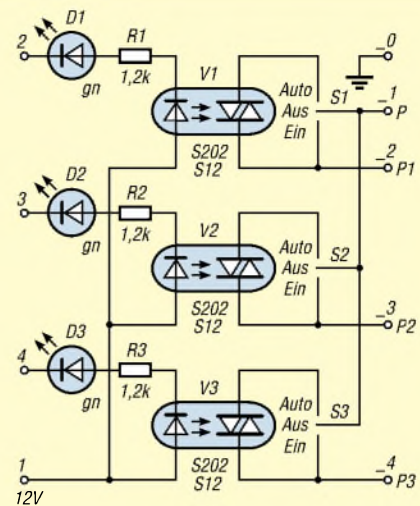
Bild 18: Beleuchtungs- und Lüftersteuerung
