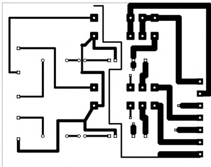
Bild 19: Layout der Rollladensteuerung
