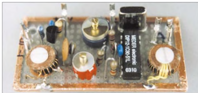
Bild 5: Aufbau des erweiterten Filters Fotos: DL7HG
