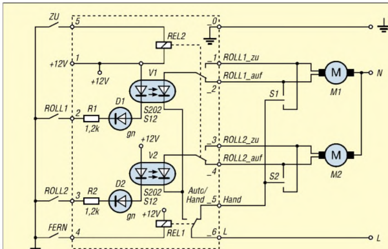
Bild 17: Rollladensteuerung
