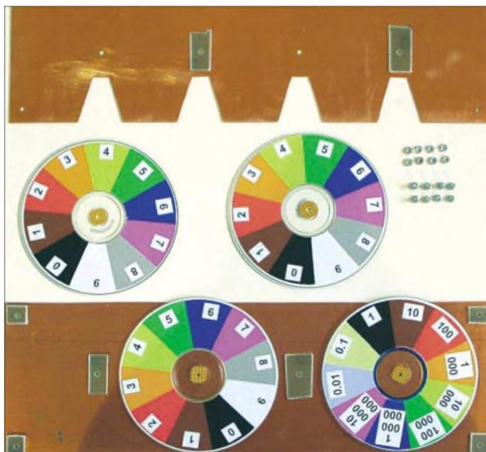
Übersicht der Einzelteile der Widerstandsuhr Foto: AATiS
