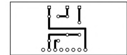
Bild 26: Layout des Lichtsensors
