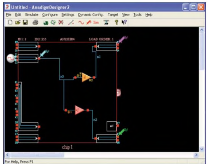
Bild 7: Das vom virtuellen Signalgenerator kommende Rechtecksignal wird differenziert, integriert und mit dem Oszilloskop betrachtet.
