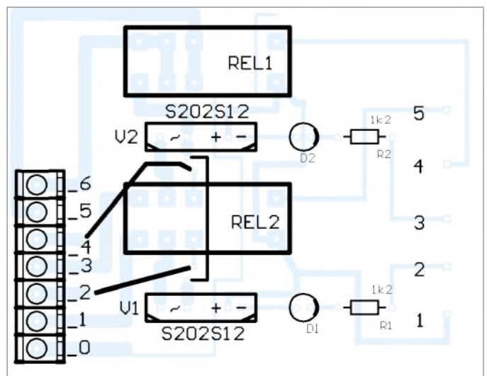
Bild 20: Bestückung der Platine für die Rollladensteuerung
