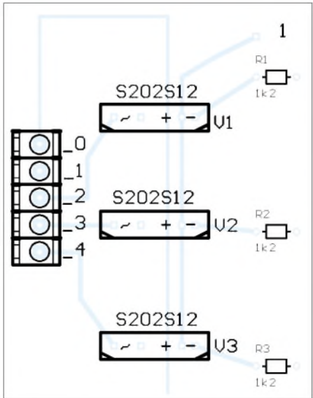
Bild 29: Bestückung der Schaltstufe für Beleuchtung und Lüfter
