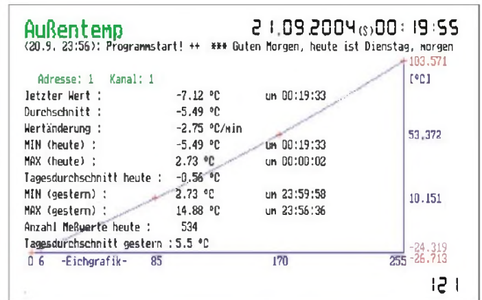
Bild 30: Im Datenlogger sind die Spannungsverläufe des Helligkeitssensors und der drei Temperatursensoren zu erkennen.
