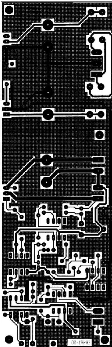
Bild 6: Unterseite der doppelt kaschier-ten Leiterplatte
