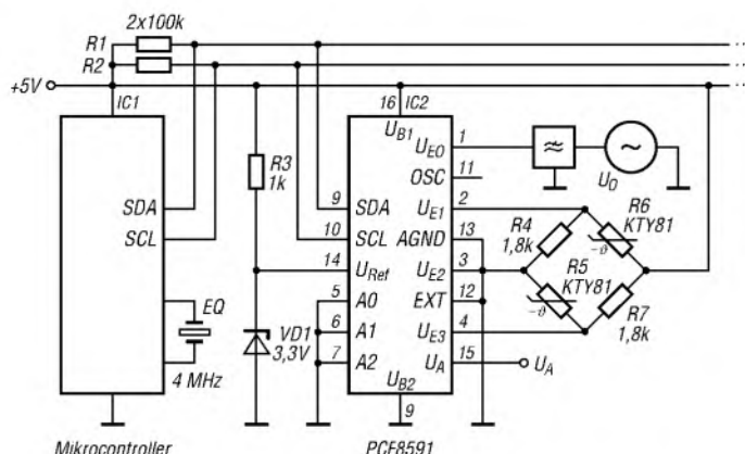
Bild 6: Nutzung des PCF8591 zur Übertragung analoger Eingangssignale verschiedener Quellen über einen I²C-Bus
