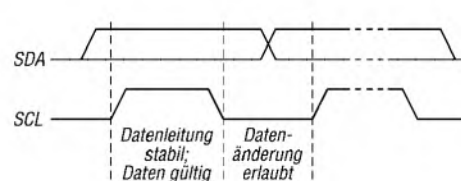
Bild 4: Bit-Transfer und Gültigkeit der Daten
