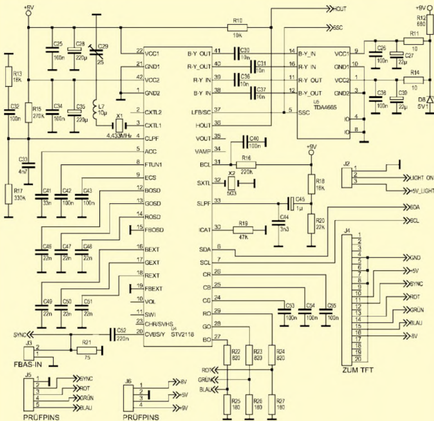
Bild 3: Herzstück der Umsetzbaugruppe ist der STV2118 im Videoteil.
