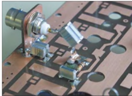
Bild 6: Eingang des Messaufbaus nach Bild 3 auf der Platinenunterseite; die Masseseite beherbergt die Ausgangsbeschaltung und schirmt diese vom Eingang ab.
