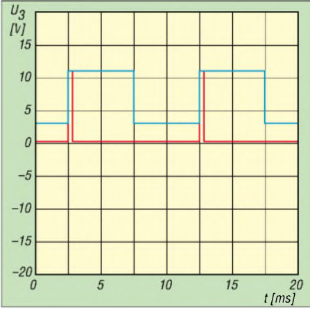
Bild 4: Je nach eingestellter Temperatur gibt IC3 bei niedrigen Werten kurze (rot) und bei hohen Werten lange Heizimpulse (blau) ab.
