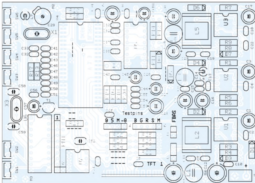
Bild 7: M1 bis M4 in der Bestückung dienen für die Befestigung am Display.
