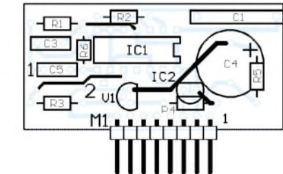
Bild 25: Bestückung des Windstärkesensors
