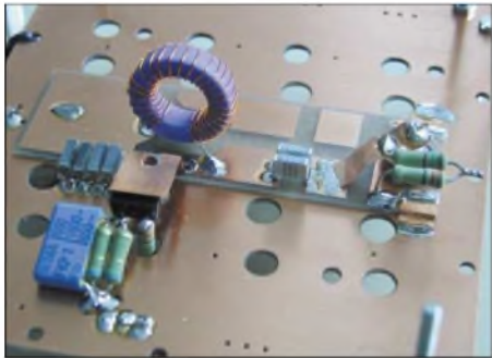
Bild 5: Messaufbau eines einzelnen Verstärkers gemäß Bild 2 ohne Parallelkompensation und Schutzbeschaltung; Ausgangsseite, Kühlkörper demontriert.
