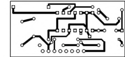
Bild 24: Layout des Windstärkesensors
