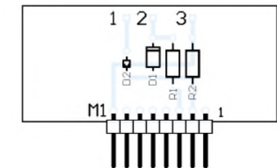
Bild 27: Bestückung des Lichtsensors
