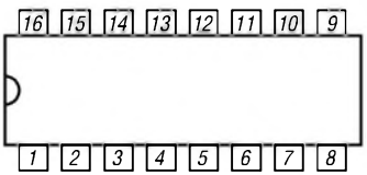
Bild 2: Pinbelegung (DIP16)
