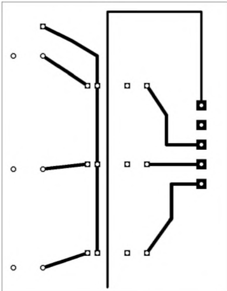
Bild 28: Layout der Schaltstufe für Beleuchtung und Lüfter
