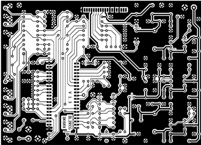
Bild 6: Layout der einseitig kaschierten Umsetzerplatine
