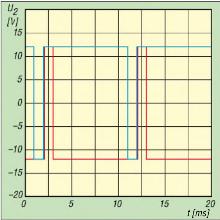
Bild 3: Ausgangsspannung an IC2 bei voller Heizleistung (blau) und nach dem Erreichen der eingestellten Temperatur (rot)
