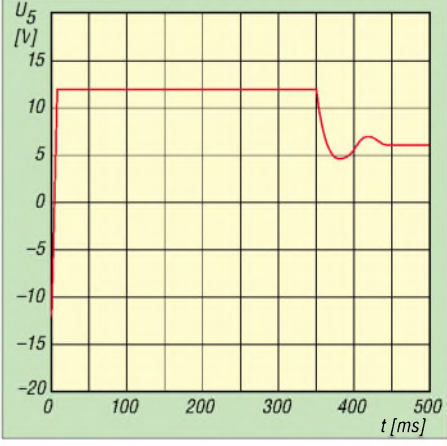
Bild 5: Das Einschwingverhalten der Regelung, hier nach 350 ms, lässt sich durch Variieren von R23 beeinflussen.
