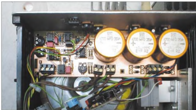
Bild 1: Die Temperaturregelung lässt sich eigenständig betreiben oder z.B. zusammen mit einer Luftpumpe für Heißluftlötkolben in ein Gehäuse integrieren. Zur besseren Darstellung wurde die Pumpensteuerung zeitweise demontiert.
