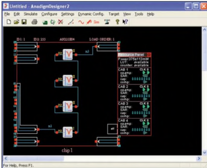
Bild 7: Das vom virtuellen Signalgenerator kommende Rechtecksignal wird differenziert, integriert und mit dem Oszilloskop betrachtet.
