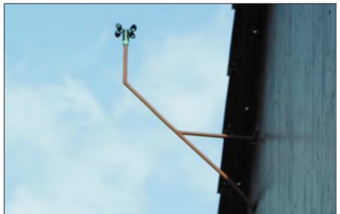
Bild 15: Anbringung des Windstärkesensors im Außenbereich an einem Ausleger
