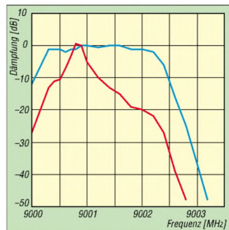
Bild 3: Frequenzgang des CW-Filters zusammen mit einem SSB-Filter älterer Bauart
