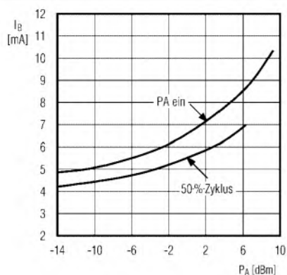
Bild 3: Betriebsstrom in Abhängigkeit von der Ausgangsleistung bei verschiedenen Modi; f_A = 433 \text{ MHz}
