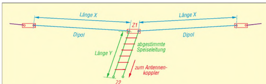
Bild 4: Grundschematische Darstellung einer symmetrisch gespeisten Doppel-Zepp-Antenne
