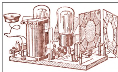
Bild 8: „Zwei Lampen“-Radio aus dem Baukasten Radio-Technik von 1930
