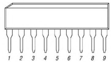
Bild 2: Pinbelegung (SIP9)
