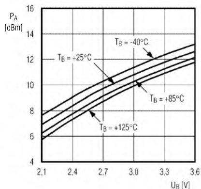
Bild 5: Ausgangsleistung in Abhängigkeit von der Betriebsspannung; f_A = 433 \text{ MHz}
