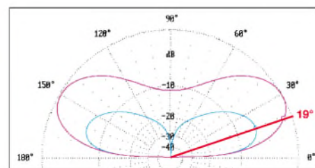
Bild 14: Vertikale Strahlungsdiagramme der Vertikalantenne (blau) und eines Halbwelldipols in 10 m Höhe (violett) über realem Grund auf 14,25 MHz; 0 dB = 6,9 dBi
