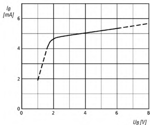
Bild 3: Abhängigkeit des Betriebsstroms von der Betriebsspannung
