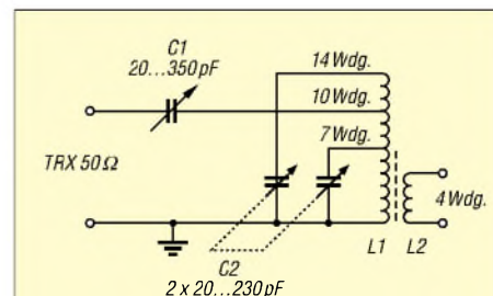
Bild 3: Grundsaltung des Z-Match
