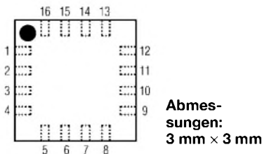
Bild 2: Pinbelegung (QFN16)
