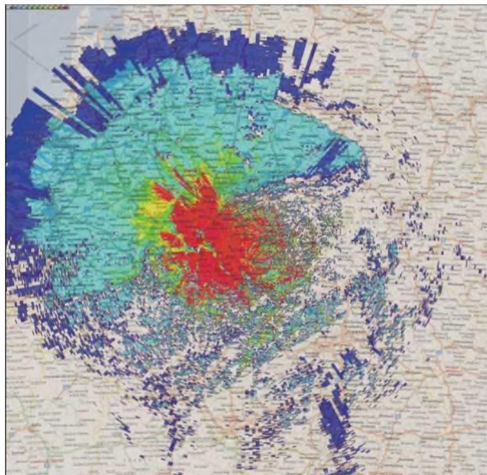
Bild 4: Interferenz zwischen den 70-cm-Relais DB0RR (erwünscht) und DB0HAT; rot = Empfang, blau = Störung (Signalunterschied weniger als 10 dB).
