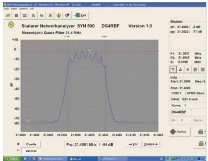
Bild 3: Screenshot der Bediensoftware während des Wobbels eines 21,4-MHz- Quarzfilters Fotos und Screenshots: DG4RBF
