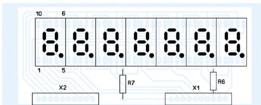
Bild 7: Bestückung der Anzeigeplatine
