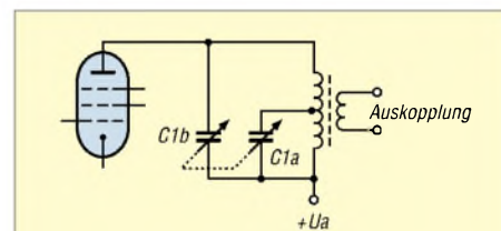
Bild 2: Multiband-Tankkreis mit nur einem Abstimmeelement nach W6MUR
