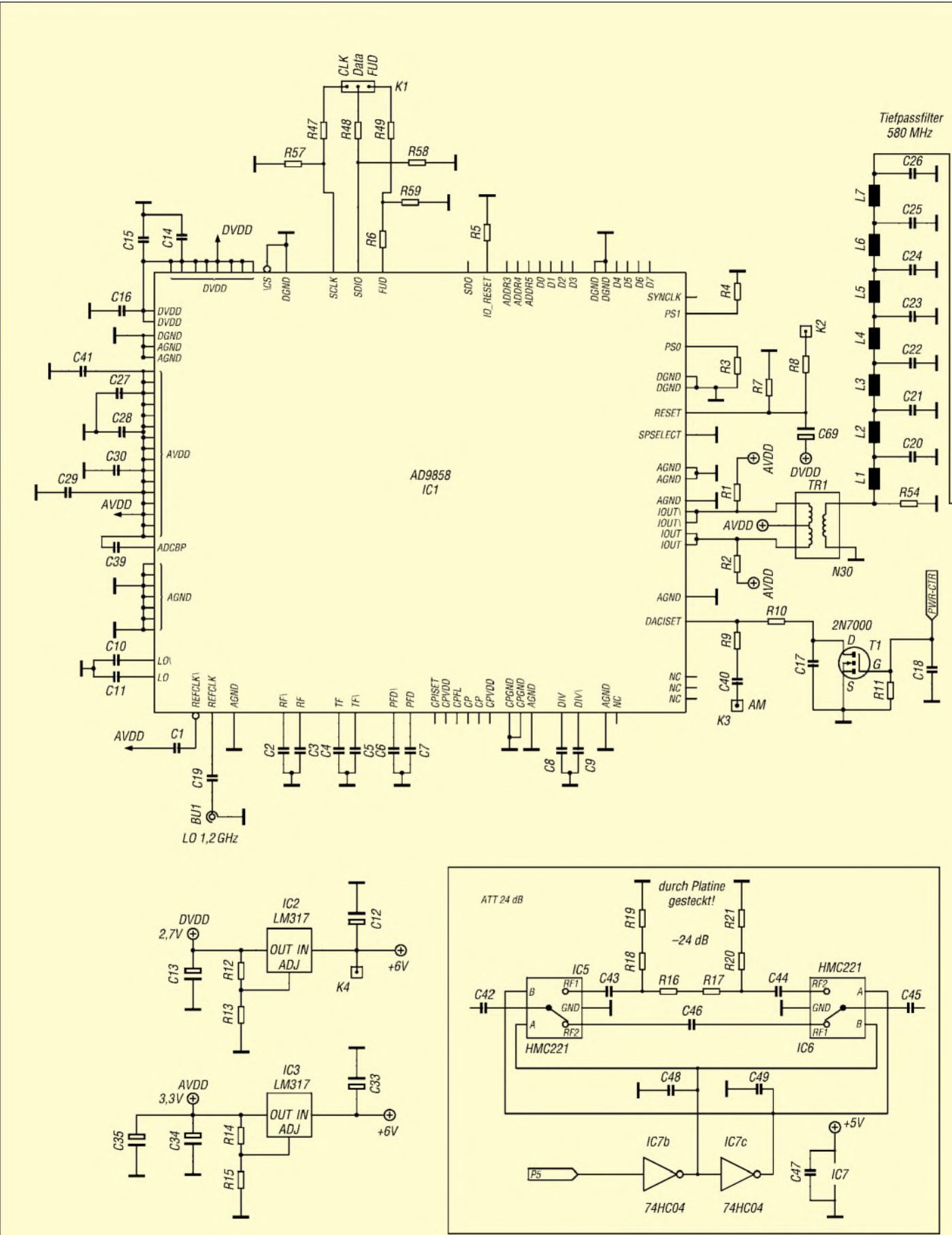
Bild 5: Schaltbild für den DDS-Signalgenerator auf S. 148–149
