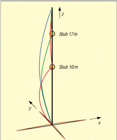
Bild 8: Stromverteilung auf der Dreibandantenne in der EZNEC-Simulation; f = 14,25 MHz (blau), 18,165 MHz (grün) bzw. 28,5 MHz (rot)
