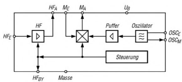
Bild 1: Blockschaltbild des TA7358AP
