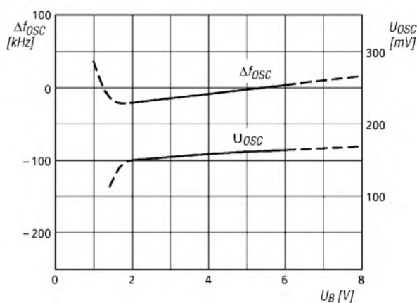
Bild 6: Frequenzänderung des lokalen Oszillators und der Oszillatorspannung in Abhängigkeit von der Betriebsspannung
