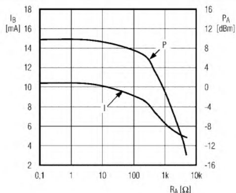
Bild 4: Betriebsstrom und Ausgangsleistung in Abhängigkeit vom Ausgangswiderstand; f_A = 433 \text{ MHz}
