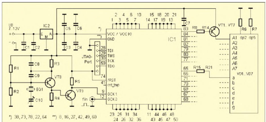
Bild 4: Stromlaufplan des 200-MHz-Frequenzzählers mit LED-Anzeige
