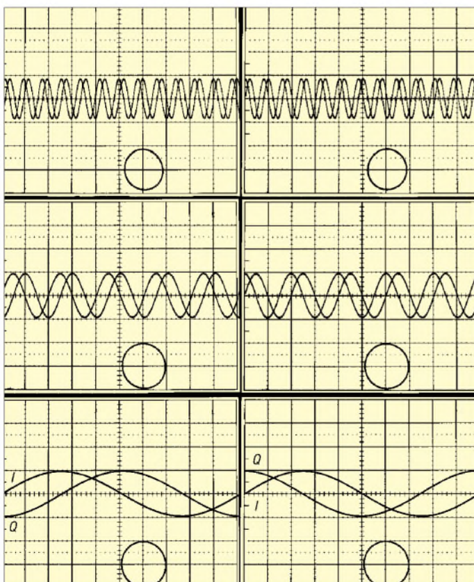
Bild 12: Gleichzeitige Darstellung der beiden NF-Signale I und Q sowie der Lissajousfigur auf einem Oszilloskop; horizontal 500 \mu s/Div., vertikal 10 mV/Div. Linke Spalte: f_{IF} > f_{LO} , NF-Signal I gegenüber Q um 90^\circ voreilend; rechte Spalte mit f_{IF} < f_{LO} , Q gegenüber I um 90^\circ voreilend. Die Phasenverschiebung beträgt unabhängig von der Frequenz immer 90^\circ .
