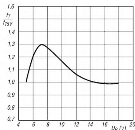
Bild 6: Abhängigkeit der auf f_{osc} bei U_B = 5 \text{ V} normierten Oszillatorfrequenz von der Betriebsspannung
