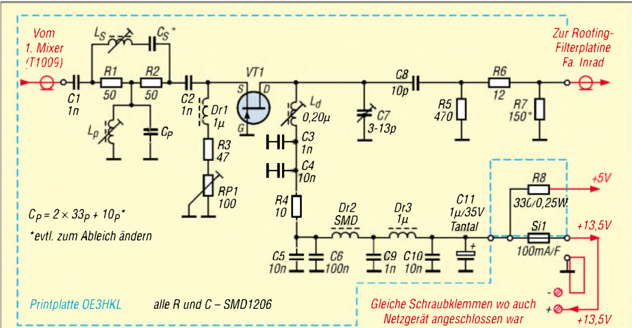
Bild 2: Schaltplan des Anpassverstärkers mit T-Diplexer, Bauelemente siehe Tabelle 1
