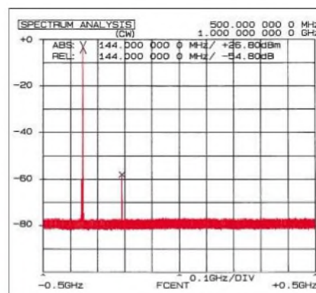
Bild 6: Ausgangsspektrum der PA bei Eintonaussteuerung und Vollast; die Unterdrückung der 1. Oberwelle beträgt 54,8 dB, die 2. geht hier schon im Rauschen unter.
