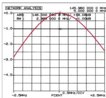
Bild 4: Frequenzgang des Vorverstärkers, die 1-dB-Bandbreite beträgt 2,88 MHz beim Testmuster; die in DL ausgelieferten PAs werden für 145 MHz Mittenfrequenz abgeglichen.
