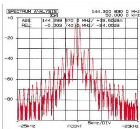
Bild 7: Ausgangsspektrum der PA bei Zweitonaussteuerung, Summen-Ausgangsleistung 350 W, IMD3 = 30,0 dB bezogen auf Einton-Aussteuerung
