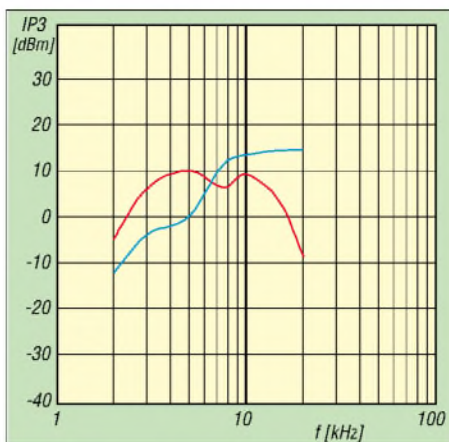
Bild 5: Änderung des IP3 mit dem Abstand der Messträger für eine (zu kleine) 7x7-mm 2 -Spule im Drainkreis; rot: Pegel des IM-Signals P_{im} = -117 dBm; blau: Pegel des IM-Signals P_{im} = -130 dBm
