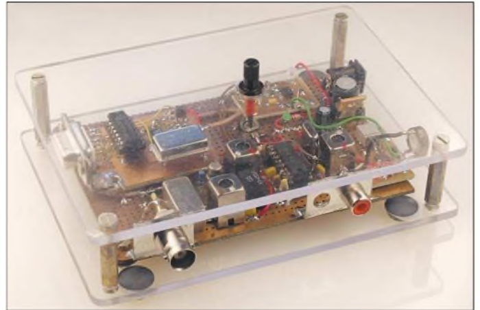
Bild 3: Versuchsstadium des Empfängers
