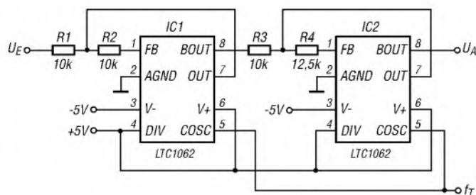
Bild 9: Kaskadiertes Bandpassfilter
