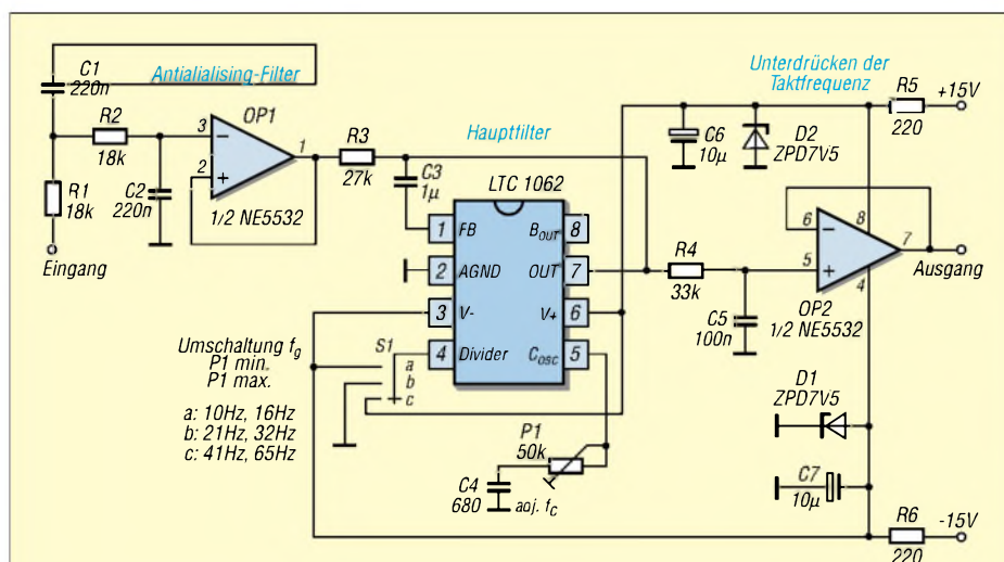
Bild 11: Gesamtschaltung des ELF-Filters mit Antialiasing-Filter, SC-Hauptfilter und Taktfrequenz-Unterdrückung
