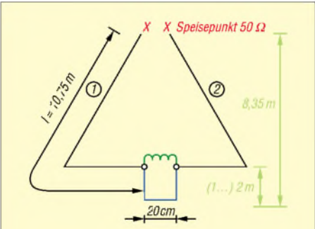
Bild 1: Prinzipdarstellung der Loop; blau – 20 m, grüne Spule – 30 m; für 40 und 15 m ist die Verbindung zwischen beiden Drahtenden aufgetrennt; Maße für Blankdraht.
