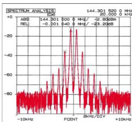
Bild 5: Ausgangsspektrum des Vorverstärkers bei zwei um 1 kHz auseinander liegenden Eingangssignalen à -15 dBm; der IM3 beträgt 23,2 dB; daraus folgt IP3 = 8,8 dBm.
