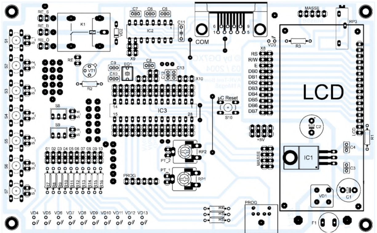
Bild 4: Bestückung der Experimen- tierplatine
