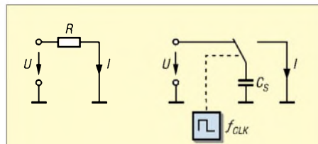
Bild 1 (links): Der Strom I wird bestimmt durch die Höhe der Spannung U und den Widerstandswert R .
