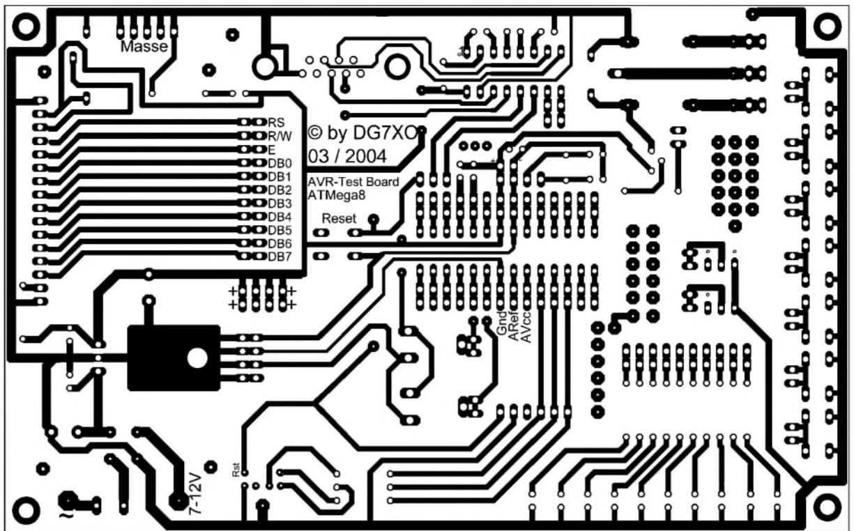
Bild 3: Layout der Experimentier- platine
