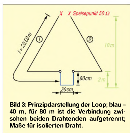
Bild 3: Prinzipdarstellung der Loop; blau – 40 m, für 80 m ist die Verbindung zwischen beiden Drahtenden aufgetrennt; Maße für isolierten Draht.
