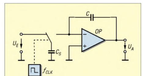
Bild 4: Hier wurde der Widerstand R des Integrators aus Bild 3 durch eine geschaltete Kapazität ersetzt.
