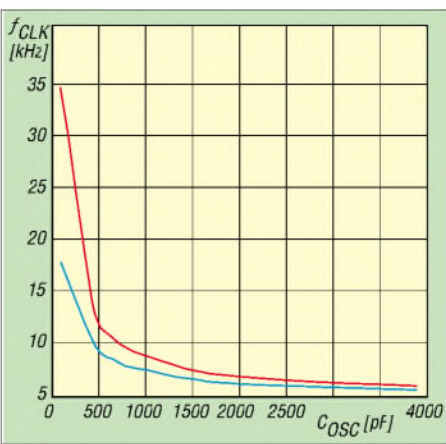
Bild 7: Gegenüberstellung der mithilfe des Datenblatts errechneten Frequenz (rote Linie) und der gemessenen Frequenz (blaue Linie) für f CLK in Abhängigkeit vom externen Kondensator C OSC (Pin 5 nach Masse)
