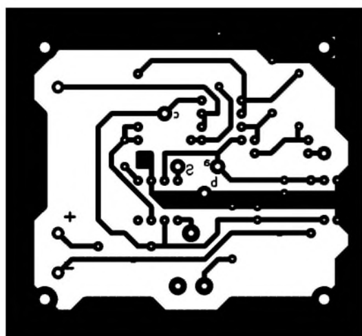
Bild 13: Leiterseite der einseitigen, 69 mm x 64 mm großen Platine SC-Filter gemäß Bild 11, M 1:1
