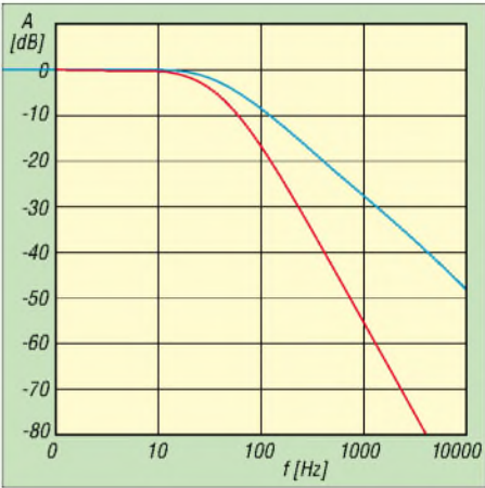
Bild 9: Frequenzgänge der Tiefpassfilter aus Bild 8 (blaue Linie) und aus Bild 10 (rote Linie)
