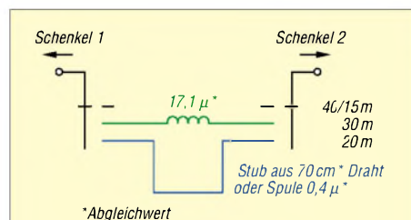
Bild 2: Mögliche Aufbauvariante für den Umschaltkasten; die beiden Ebenen des Umschalters können auch durch Relais ersetzt werden.
