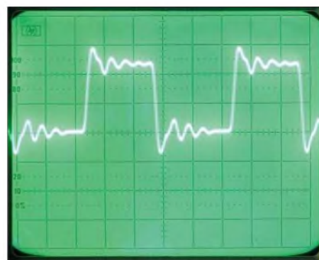
Bild 5: Oszillogramm der 10-MHz-Referenzfrequenz mit 0,2 V/Div nach 10:1-Tastkopf
