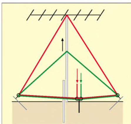
Seilführung beim Aufbau; Umlenkrollen an den Heringen und das Zusammenfassen der Seile einer Ebene vereinfachen den Aufbau sehr.
