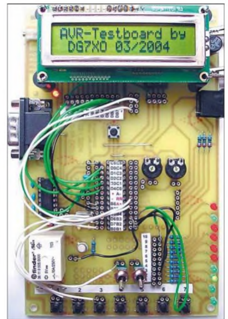
Bild 2: Entwicklungsboard für den ATmega8 im Einsatz Foto: DG7XO
