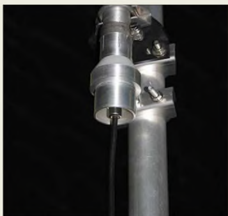
Mit modernen Produktionstechnologien verbessert hofi die jahrzehntelang bewährten Fritzel-Antennen – hier die neue wassergeschützte Einspeisung der Groundplanes.
