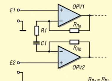
Bild 12: Durch Einfügen eines Kondensators ist der Verstärker für Wechselspannungen modifizierbar.
