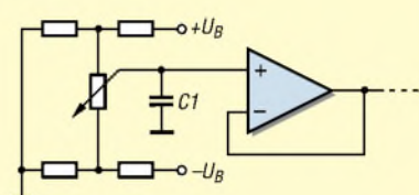
Bild 9: Maßnahmen 2 zur Offseiteinstellung bei externer Kompensation
