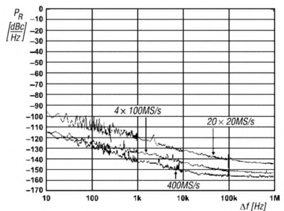
Bild 8: Phasenrauschen P_R in Abhängigkeit vom Abstand zur Ausgangsfrequenz f_A = 9,5 MHz bei verschiedenen Referenztakten
