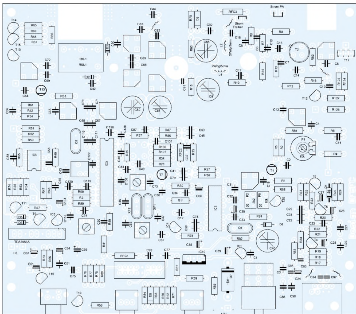
Bild 13: Die Oberseite der Hauptplatine mit dem Bestückungs- druck
