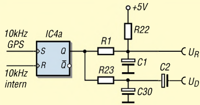
Bild 5: Die Regelspannungen U_R zur Frequenzeinstellung und die Spannung U_D für den Diskriminator werden von der FLL abgeleitet.
