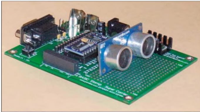
Bild 1: Versuchsaufbau auf einem Entwicklungs- board mit der Basic Stamp und einem Ping-Modul
