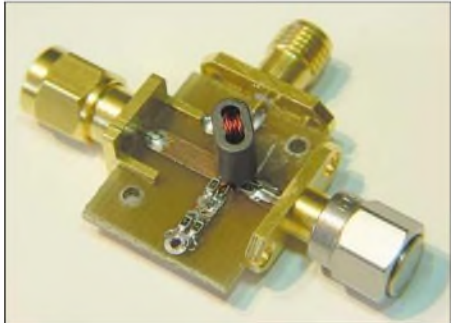
Bild 1: Fertig aufgebaute Messbrücke, noch ohne Masseplatte, rechts mit einem SMA-Abschlusswiderstand als Messobjekt versehen
