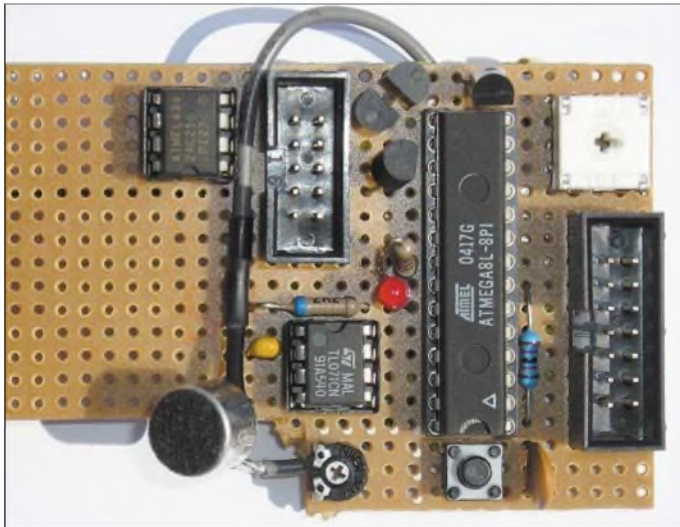
Bild 1: Prototyp des Rufzeichendecoders auf einer Lochrasterplatine
