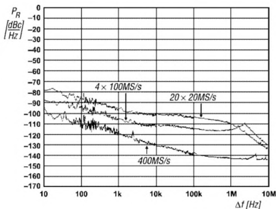
Bild 7: Phasenrauschen P_R in Abhängigkeit vom Abstand zur Ausgangsfrequenz f_A = 159,5 MHz bei verschiedenen Referenztakten
