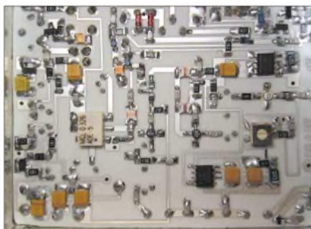
Bild 13: Platinenunterseite – wer noch nie Umgang mit SMD hatte, sollte zuvor Literatur hinzuziehen [6], [7] und mit anderen SMD-Bauelementen auf einer Probeplatine üben.
