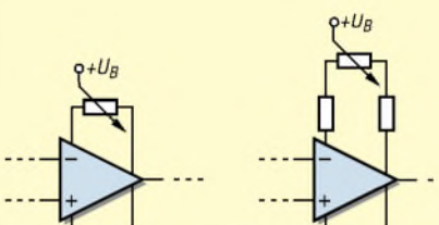
Bild 10: Beschaltung 1 bei interner Offseiteinstellung
