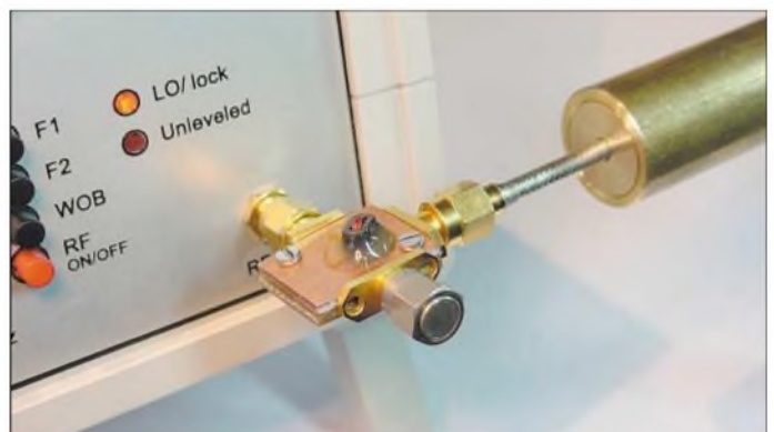
Bild 3: Messanordnung mit angeschlossenen Detektor (rechts) und einem SMA-Abschlusswiderstand (vorn) als Messobjekt (DUT).
