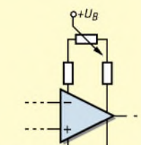
Bild 11: Beschaltung 2 bei interner Offseiteinstellung
