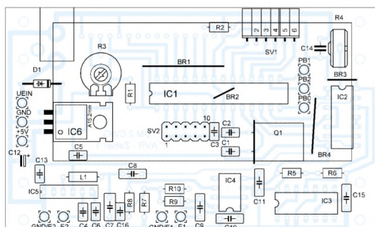
Bild 4: Bestückung der AVR- Zählerplatine
