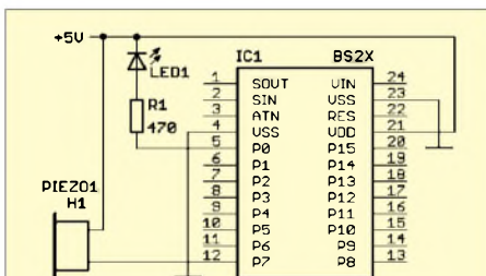
Bild 7: Als erste Lebenszeichen lassen wir eine LED blinken und eine Melodie abspielen.
