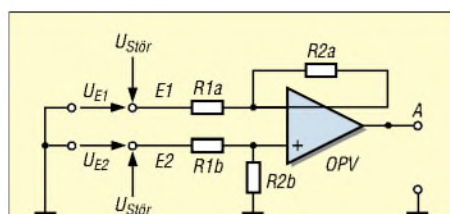
Bild 2: Differenzverstärker mit bezugs-potenzialgebundener Ankopplung
