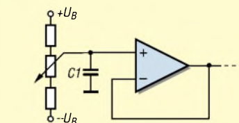
Bild 8: Maßnahmen 1 zur Offseiteinstellung bei externer Kompensation
