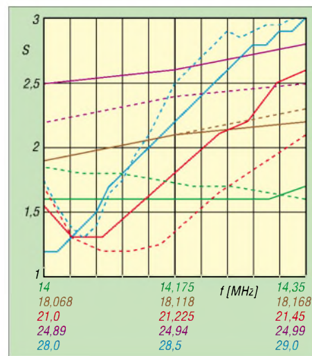
Bild 9: Gemessene Verläufe des SWV ohne Zwischenschaltung eines Antennentuners; gestrichelt: geänderte Herabführung der Speiseleitung, siehe Text
