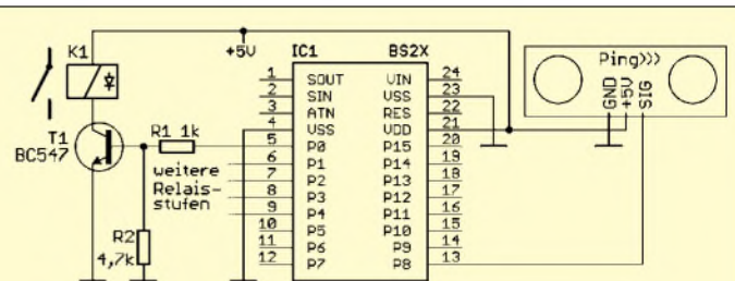
Bild 6: Durch eine Basic Stamp lassen sich mehrere Relaisstufen ansteuern und Ultraschallmodule abfragen.
