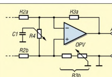
Bild 7: Maßnahmen zur Störunterdrückung
