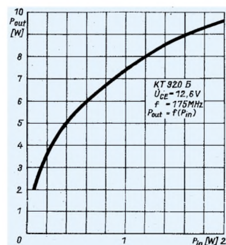
Bild 12: Leistungsverstärkung des KT920B bei 175 MHz [1]
