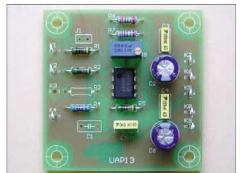
Bild 14: Platine UAP13 als Zweifach-Summierverserker beschaltet
