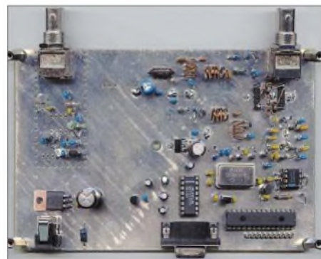
Bild 2: Die geringe Anzahl der Bauelemente gestattet auf einer Europakarte einen lockeren Aufbau ohne SMD und vor allem ohne jeglichen Drahtverhau. Foto: DK3WX
