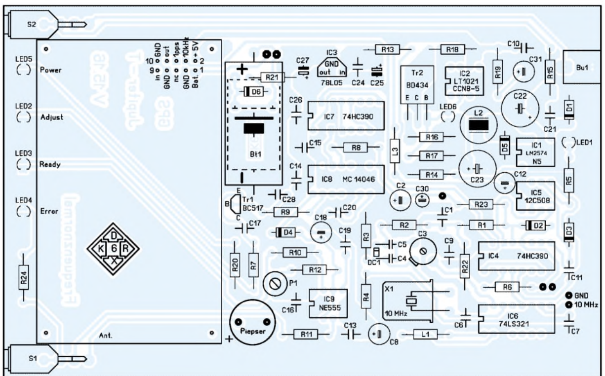
Bild 14: Bestückung des GPS-Frequenz- normalis – das GPS-Modul wird auf die PLatine aufgesteckt.
