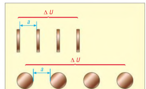
Bild 2: Vergleich des Platzbedarfs von Spulenwindungen aus Flachkupfer bzw. Rundmaterial; Windungsabstand a und HF-wirksame Oberfläche sind gleich.
