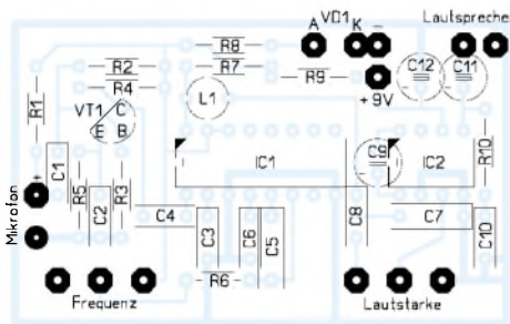
Bild 4: Bestückung der Platine des Fledermausdetektors
