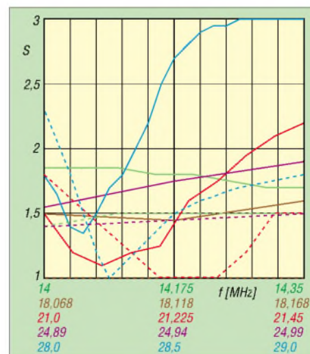
SWV-Verläufe bei DL2RD (durchgezogen) und DL6LAU (gestrichelt)
