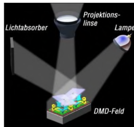
Das Licht wird vom DLP-Spiegel entweder durch die Linse auf die Leinwand oder auf einen Absorber im Gerät geleitet.
