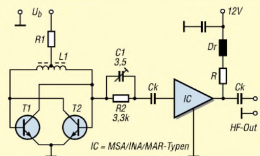
Bild 7: Oszillator mit Verstärkerstufe; zu den MMICs siehe Bauele- mente-Infoma- tionen FA 9/03 sowie S. 1035 f.
