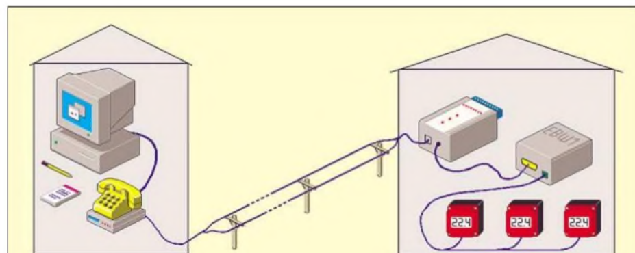
Bild 3: Mit dem Modem IAM80 der Fa. Greisinger und dem ebenfalls angebotenen Pegelwandler EBW1 ist eine Konfiguration und Abfrage von Datenloggern der Serie Easy Bus auch über größere Entfernungen möglich.
