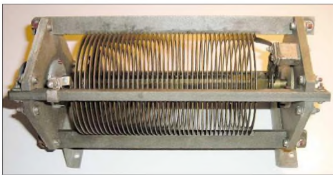
Bild 1: Rollspule russischer Fertigung
