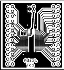
Bild 17: Bestückungsseite der Adapterplatine.
