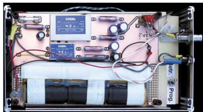
Bild 15: Stromversorgungs- platine im eingebauten Zustand
