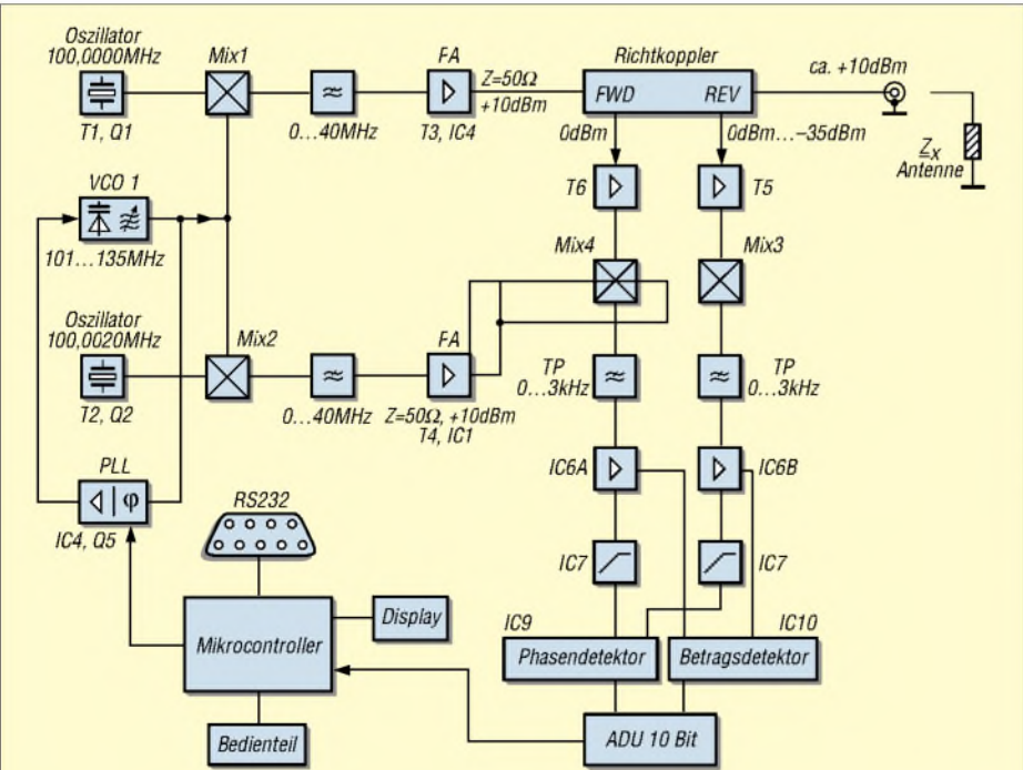
Bild 1: Komplettes Blockschaltbild des Antennenanalysators AA
