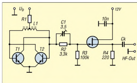
Bild 6: Oszillator mit FET-Puffer
