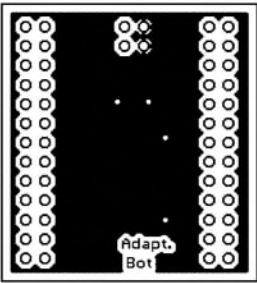
Bild 16: Lötseite der Adapterplatine.
