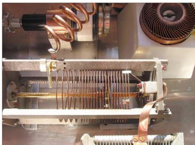
Bild 4: Umgebaute Rollspule mit separater 10-m-Spule in einer GS35-Endstufe; nach Ausbau des unbenutzten Wicklungsteils wird eine Spreizung der Windungen zum heißen Ende hin möglich.
