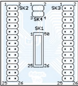
Bild 18: Bestückung der Adapterplatine
