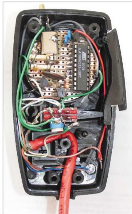
Bild 5: Innenleben des in ein Mikrofon eingebauten Prototyps; Herz der Schaltung ist ein Mikrocontroller ATME1 AT90S2313.
