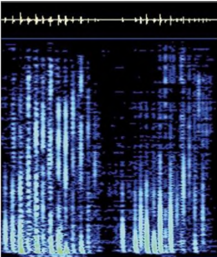
Bild 8: Sonogramm einer Zwergfledermaus
