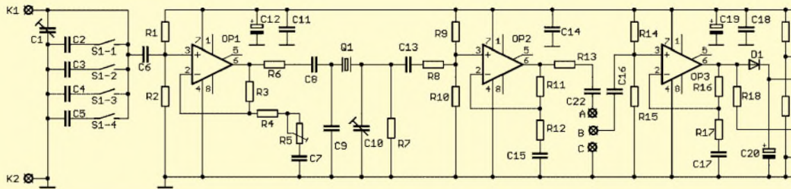
Bild 19: Stromlaufplan der Platine GE1
