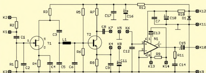
Bild 21: Stromlaufplan der Platine SEP1
