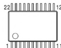
Bild 1: Pinbelegung (SOP22)
