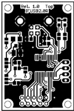
Bild 5: Bestückungsseite der 45,72 mm x 30,48 mm großen, zweiseitig kaschierten Leiterplatte
