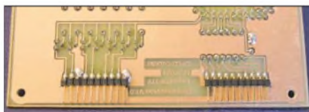
Bild 2: Unter die Hauptplatine werden abgewinkelte Steckerleisten gelötet.
