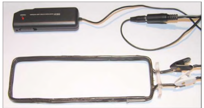
Bild 14: Übers Radio geschoben, überträgt der Koppelrahmen Mittelwellensignale induktiv auf die Ferritantenne.
