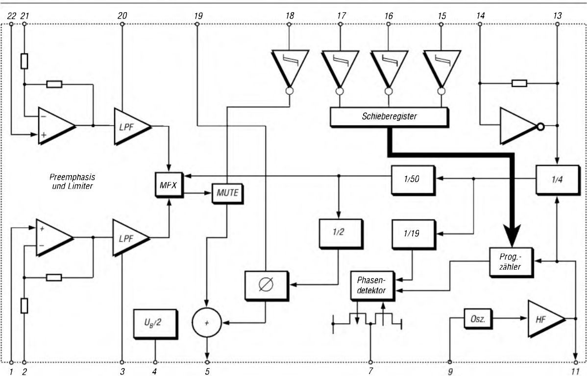
Bild 2: Blockschaltbild des BH1415F
