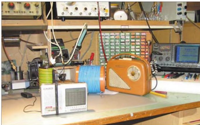
Bild 14: Übers Radio geschoben, überträgt der Koppelrahmen Mittelwellensignale induktiv auf die Ferritantenne.
