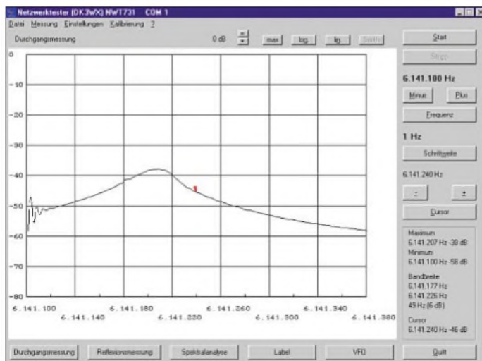
Bild 5: Screenshot einer Quarzresonanzkurve mit dem NWT
