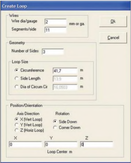
Bild 1: Das Fenster Create Loop (Schleife erzeugen) mit den Grunddaten der ersten dreieckigen Schleife. Durch Anklicken von OK sind die Drähte im Handumdrehen definiert.
