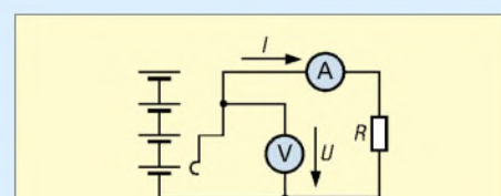
Bild 4: Anordnung zur Messung des Zusammenhangs zwischen Spannung und Stromstärke bei konstantem Widerstand
