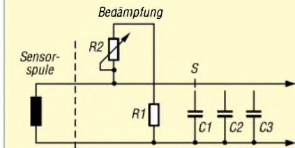
Bild 29: Prinzip der Frequenzbereichsumschaltung der Sensorspule
