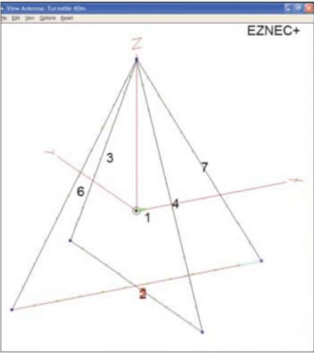
Bild 2: Die beiden Dreieckschleifen aus den Drähten 2, 3, 4 und 5, 6, 7 sind vertikal um 5 cm gegeneinander verschoben, sodass sich die beiden Dreiecksspitzen oben nicht berühren. Draht 1 ist ein Hilfsdraht, der die Quelle trägt und der später gelöscht wird.
