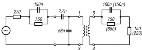
Bild 4: Erzielung eines flachen Frequenzgangs während des Sendens und Empfangens bei Beschaltung mit der komplexen CTR21-Referenz-Impedanz. Typische Werte sind ±0,5 dB im Frequenzbereich von 300 Hz bis 3,4 kHz. Die Werte in Klammern ergeben eine optimal flache Durchgangskurve zu Gunsten einer etwas geringeren Rückflussdämpfung.
