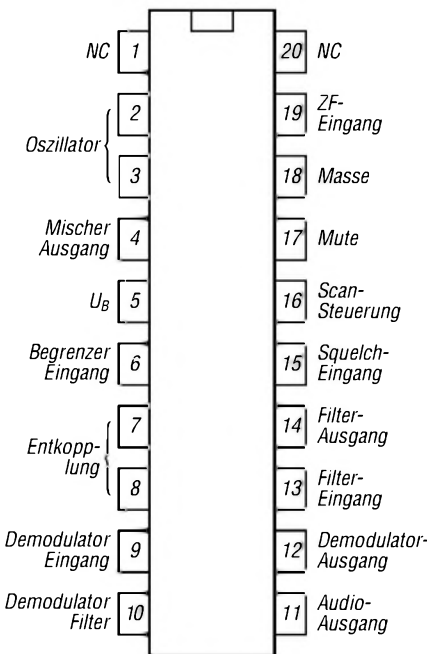
Bild 2: Anschlussbelegung des SMD-Gehäuses
