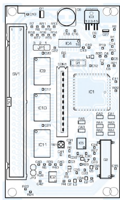
Bild 8: Bestückung der DDS-25-Platine
