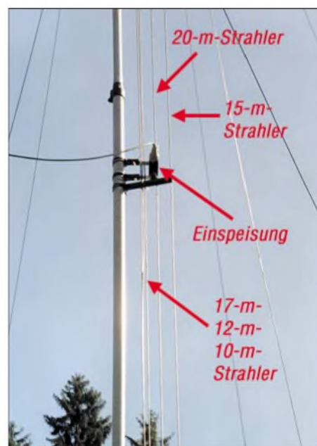
Bild 11: Anordnung der einzelnen Strahler in der Nähe des Speisepunktes
