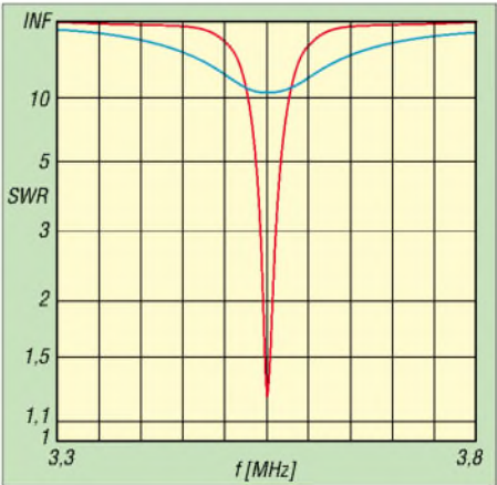
Bild 14: Blau – Welligkeit der Drehkreuzantenne für das 80-m-Band bei direktem Anschluss an ein 50-Ω-System. Die hohe Welligkeit rührt von der Fehlanpassung des niedrigen Resonanzwiderstands Z_A = 4,6 \Omega an 50 Ω her. Rot – Welligkeit bei breitbandiger 1:10-Anpassung von 5 Ω an ein 50-Ω-System. Die Schmalbandigkeit der Kurve ist eine Folge der für das 80-m-Band zu geringen Antennengröße.
