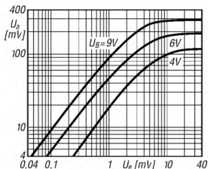
Bild 3: Spannung an Pin 3 bzw. 4 über U_B
