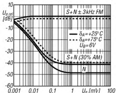
Bild 5: Relative Ausgangsspannungen über U_B
