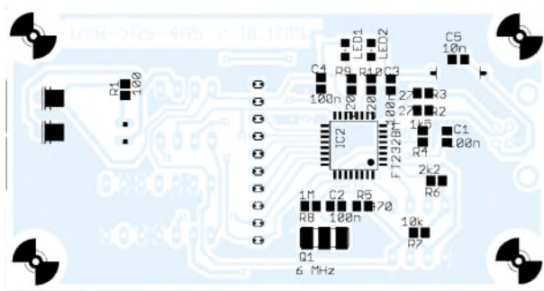
Bild 6: Bestückungs- plan Kupfer- seite
