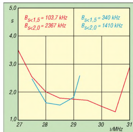
Bild 4: Doppelstrahlerelemente (rot) versus Einzelemente (blau), simuliert
