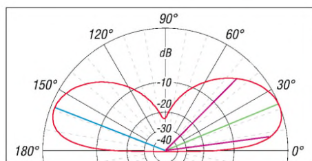
Bild 16: Strahlungsdiaagramm bei Betrieb im 80-m-Band; der Abstrahlwinkel ist mit 22° sehr gut für DX-Betrieb geeignet, der Gewinn der Antenne (äußerer Ring -14,7 \text{ dBi} ) ist aber völlig ungenügend.
