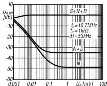
Bild 6: Relative Ausgangsspannungen über U_B
