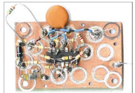
Bild 4: Schaltkreise in DIL-Gehäusen lassen sich bei der Ugly-Construction-Methode ebenfalls einsetzen, wenn sie z.B. rücklings auf die Platine aufgeklebt und dann verdraht werden.
