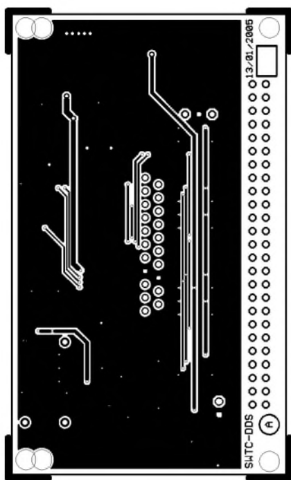
Bild 6: Layout der Platinenoberseite
