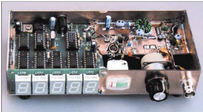
Bild 1 : Ansicht des zum Allweckzähler er- weiterten einfachen CMOS-Zählers
