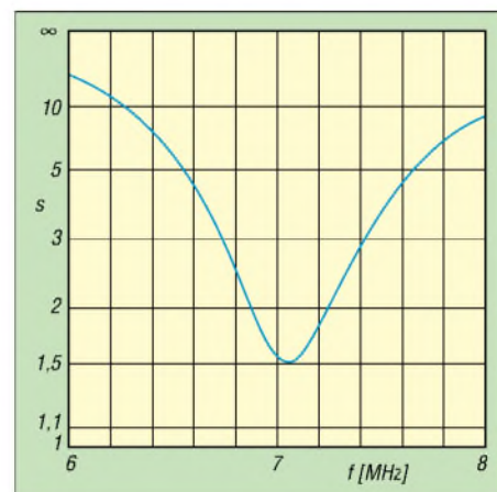
Bild 23: Welligkeit s der Antenne (12)Drehkreuz(11m;c=3m)40m.ez in Abhängigkeit von der Frequenz im 40-m-Band
