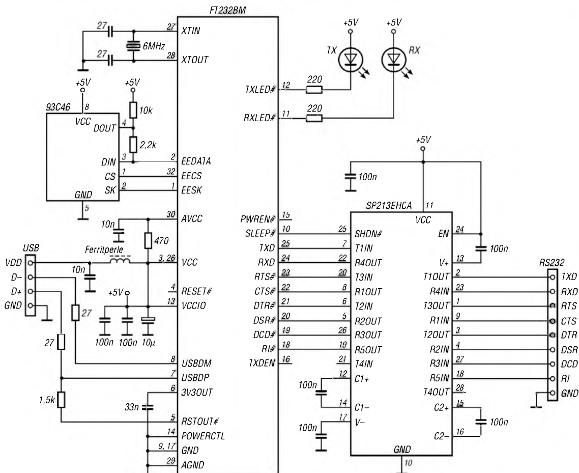
Bild 3: FT232RL als Umsetzer zwischen einer USB- und einer RS232-Schnittstelle
