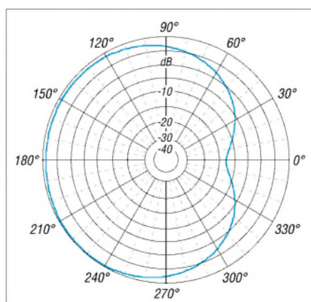
Bild 6: Horizontales Strahlungsdiagramm eines mit \alpha = 50^\circ abgespannten Slopers über schlecht leitfähigem Boden; der äußere Ring entspricht G = 1,2 dBi; Erhebungswinkel \theta = 31^\circ .
