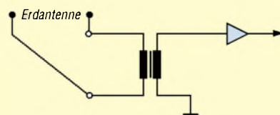
Bild 7: Antennenankopplung über einen Übertrager
