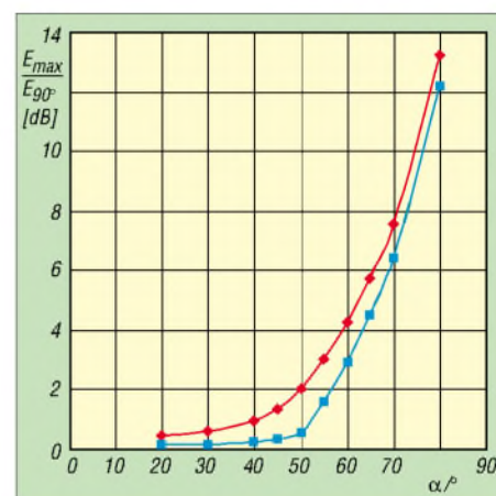
Bild 7: Unterdrückung der Steilstrahlung gegenüber dem Maximum der Strahlungskeule für gute (blau) und schlechte (rot) Bodenleitfähigkeit
