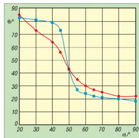
Bild 3: Erhebungswinkel \theta der Strahlungskeule eines Slopers in Abhängigkeit des Abspannwinkels \alpha für gute Bodenleitfähigkeit (blau, Land) bzw. schlechte Bodenleitfähigkeit (rot, Stadt)
