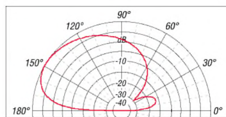
Bild 10: Vertikales Strahlungsdiagramm einer Sloper-Antenne mit Metallmast als Reflektor über schlecht leitendem Grund; der äußere Ring entspricht G = 2 dBi.
