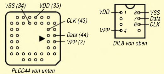
Bild 3: Besonders bei SMD-Bauteilen ist die Programmierung innerhalb der Anwenderschaltung via ICSP-Schnittstelle erforderlich. Zwei als Beispiele herausgesuchte IC-Gehäuse zeigen, wie das ICSP-Kabel anzuschalten ist.
