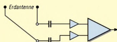
Bild 8: Ein Instrumentationsverstärker wird für die Antennenanpassung benutzt. Bei netzbetriebenen Folgegeräten hat sich allerdings ein nachgeschalteter Übertrager bewährt.
