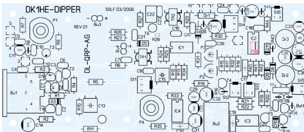
Bild 5: Bestückungsplan der Dipmeters Dip-It ; auf der Unterseite der doppelseitigen Platine ist lediglich der SMD- Kondensator C39 zu bestücken, hier rot eingezeichnet. Download des Platinen- layouts bzw. Bezug der Platine: [2]
