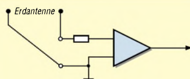
Bild 6: Anpassung der Erdantenne an einen batteriebetriebenen Empfänger ohne Verbindung zu Schutzgeerdeten Folgegeräten
