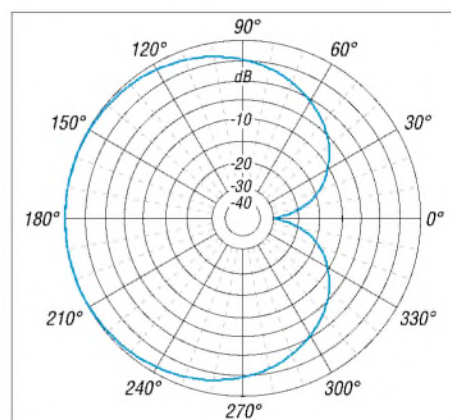
Bild 11: Horizontales Strahlungsdiagramm eines Slopers mit Metallmast als Reflektor über schlecht leitendem Boden; der äußere Ring entspricht G = 2 dBi; Erhebungswinkel \theta = 34^\circ .
