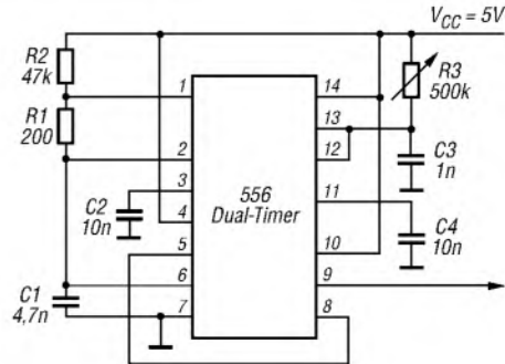
Bild 5: Durch die an den Pin /BL angeschlossene Timer-schaltung lässt sich durch Veränderung von R3 die Helligkeit der Anzeige steuern.
