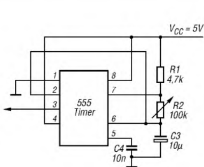
Bild 4: Durch den Timer am Anschluss /BL ist die Realisierung einer mit etwa 2 Hz blinkende Anzeige möglich.
