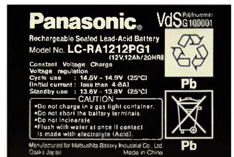
Bild 2: Neben Warnhinweisen und Umweltvorschriften sind auch Parameter für die korrekte Ladung auf dem Gehäuse aufgedruckt.
