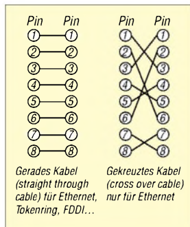
Bild 5: Im Netzwerk werden gerade und gekreuzte Kabel verwendet. 1/2, 3/6, 4/5 und 7/8 sind in jedem Fall untereinander verdreht.
