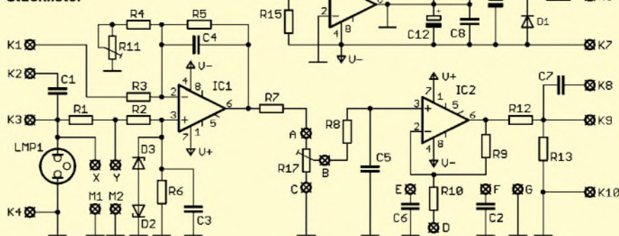
Bild 5: Stromlaufplan von ZV2; für die beschriebene Applikation erfolgt eine Teilbestückung nach Stückliste.
