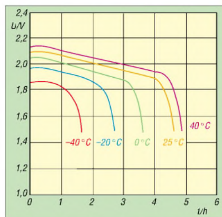
Bild 5: Zeitlicher Verlauf der Zellenspannung eines Bleigel-Akkumulators bei einem Entladestrom von I_L und unterschiedlichen Umgebungstemperaturen.
