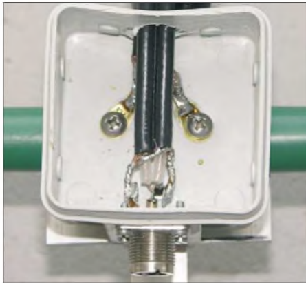
Bild 3: Strahlerdose mit angeschlossener Anpassleitung; zwischen den Lötösen liegt, hier verdeckt, ein Metalloxid-Schichtwiderstand 18 kΩ / 2 W zum Schutz vor statischen Aufladungen.
