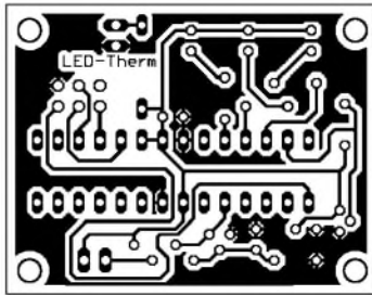
Bild 3: Die Platine für Durchsteckmontage ist 45,1 mm × 35,2 mm groß.
