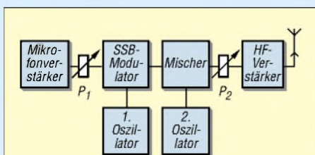
Bild 41: Prinzip eines SSB-Senders
