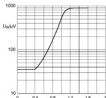
Bild 5: Rauschspannung U_R am Ausgang in Abhängigkeit von der Steuerspannung U_C
