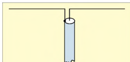
Bild 1: Symmetrischer Dipol, gespeist mit unsymmetrischem Koaxialkabel
