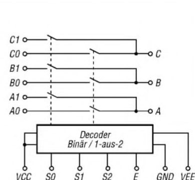
Bild 3: Blockschaltbild des 74HC4053
