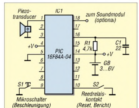
Bild 4: Schaltung des Simulators mit Bewegungssensor, Ausgabe- und Abfragemöglichkeiten
