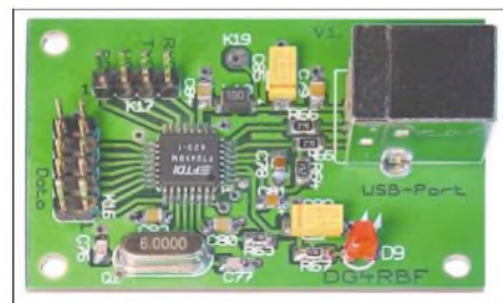
Bild 18: Die USB-Schnittstellenplatine ist nur für die Kopplung mit einem PC erforderlich. Soll der Netzwerkanalysator als reines Standalone-Gerät arbeiten, kann sie entfallen.
