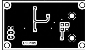
Bild 9: Für das RS485-Interface ist eine zweiseitige Platine erforderlich.
