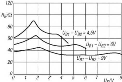
Bild 6: Einschaltwiderstand R_E in Abhängigkeit von der Eingangssignalspannung U_E bei unterschiedlichen Betriebsspannungen
