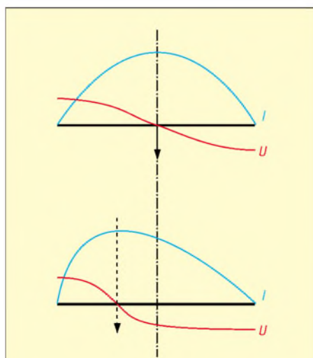
Bild 2: Oben: symmetrischer Halbwellendipol mit Strom- und Spannungsverteilung bei Resonanz, die Speisung erfolgt in der Mitte; unten: Dipol mit unsymmetrischer Strom- und Spannungsverteilung, gespeist mit außermittig angebrachtem Koaxialkabel
