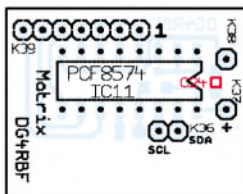
Bild 13: Bestückung der Matrixtastaturplatine
