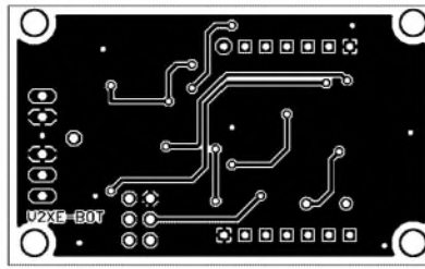
Bild 6: Die Unterseite der Kompassplatine besitzt große Masseflächen.
