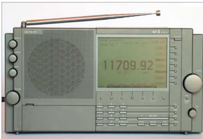
Bild 1: Auf der rechten Hälfte der Gehäusefront umrahmen 35 Tasten und ein Wippschalter das mit einem Format von 116 x 85 mm 2 für einen tragbaren Weltempfänger ungewöhnlich große Punktmatrix-LC-Display mit abschaltbarer Hintergrundbeleuchtung, das sich am besten direkt von vorne ablesen lässt.
