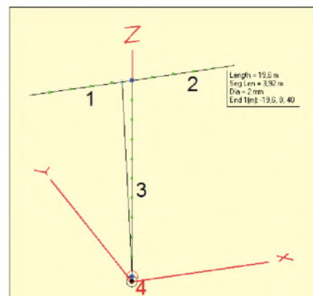
Bild 3: Horizontal aufgehängter Dipol, simuliert mit zweimal fünf Segmenten; der Anschlusspunkt des feldstörenden Koaxialkabelaußenleiters (Draht3) liegt genau in der Dipolmitte (blaues Quadrat), das virtuelle Kabel ist deutlich links davon in der Mitte des letzten Segments von Draht1 angeschlossen; das eingeschobene erläuternde Bild für die Draht- und Segmentlängen erscheint im Antennenbild beim Anklicken des Drahtes 1 bzw. 2. (1)Dipolspeisung.ez.
