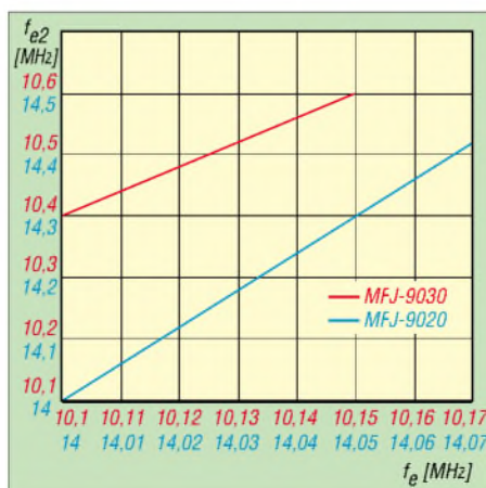
Bild 2: Nebenempfang f_{e2} durch Oszillatoroberwellen-Mischung
