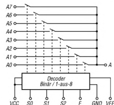
Bild 1: Blockschaltbild des 74HC4051
