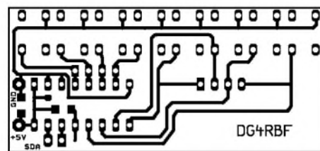
Bild 16: Layout der sich seitlich vom LC-Display befindlichen Tasterplatine
