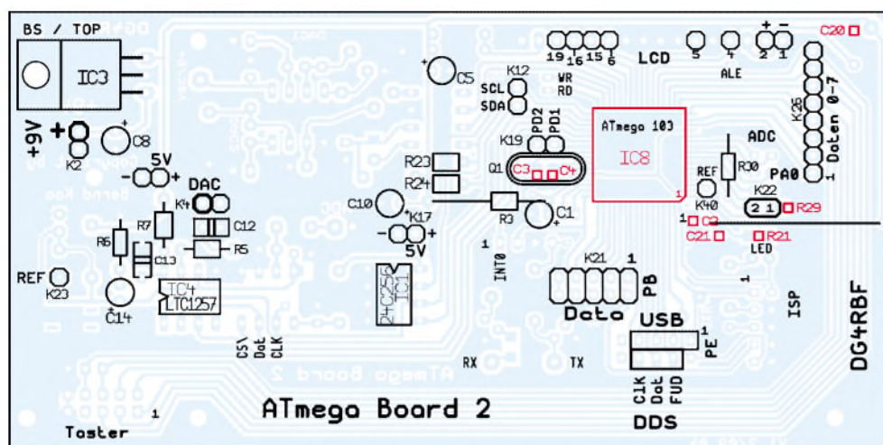
Bild 19: Bestückung des Mikrocontroller-Boards; die rot dargestellten Bauteile sind auf der Unterseite aufzulöten. Das Layout der einseitigen Platine ist unverändert [1] zu entnehmen.
