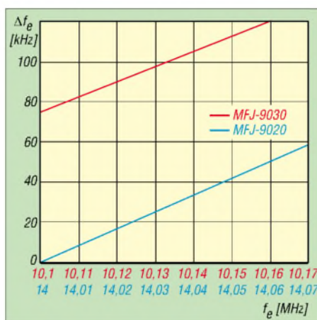
Bild 1: Doppelempfang von f_o um \Delta f_e (tiefer) durch Oszillatoroberwellen-Mischung (beim MFJ-9030 nicht einstellbar)
