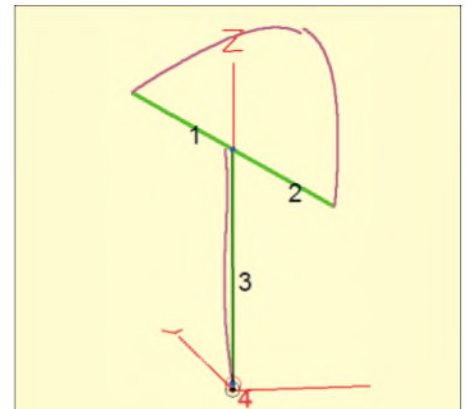
Bild 6: Schräg aufgehängter Dipol – diese Aufhängung erzwingt eine Unsymmetrie. (3)Dipol(50m-30m).ez
