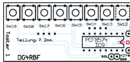
Bild 17: Bestückung der sich seitlich vom LC-Display befindlichen Tasterplatine
