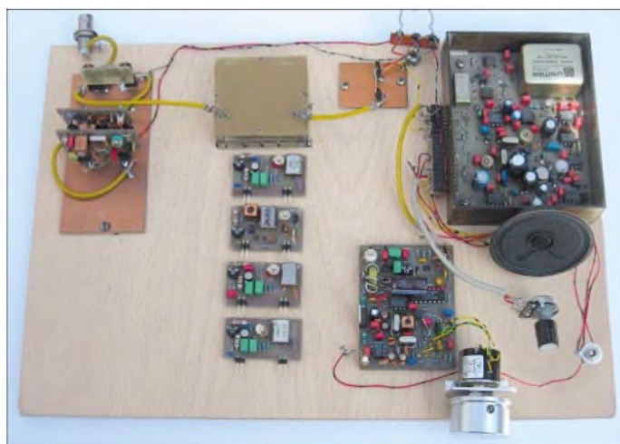
Bild 6: Versuchsaufbau – links oben 17-dBm-Eigenbaumischer, darunter LO-Treiber, davor ein Bandsetz-oscillator-Steckmodul; in der Mitte das Helix-Filter, darunter vier weitere XO-Steckmodule; rechts ein älterer SSB-Exciter, darunter 48-MHz-PLL-VFO
