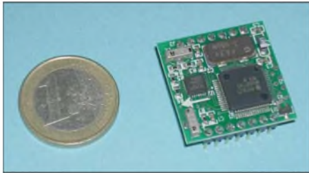
Bild 1: Der Kompasssensor V2XE im Größenvergleich mit einer 1-€-Münze
