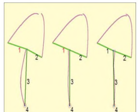
Bild 7: Stromverteilungen für drei unterschiedliche Speisepositionen beim schräg aufgehängten Dipol nach Bild 6; links: Kabelanschluss bei x = 2 m, Mitte: Anschluss bei x = 0 (Dipolmitte), rechts: Anschluss bei x = -0,8 m mit einem Minimum des Mantelstroms (3)Dipol(50m-30m).ez
