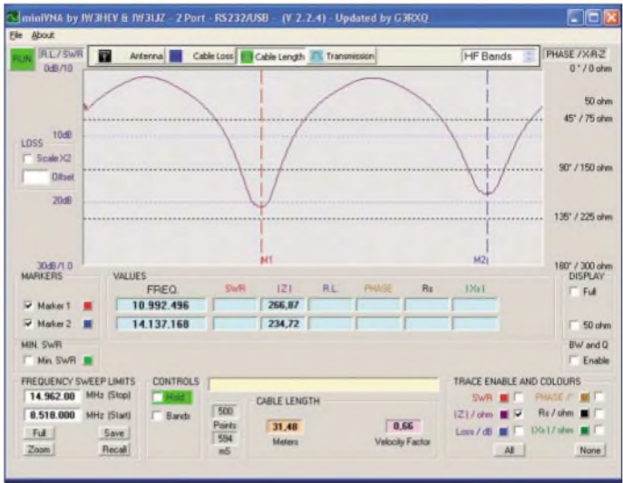
Bild 3: Messung der Kabellänge
