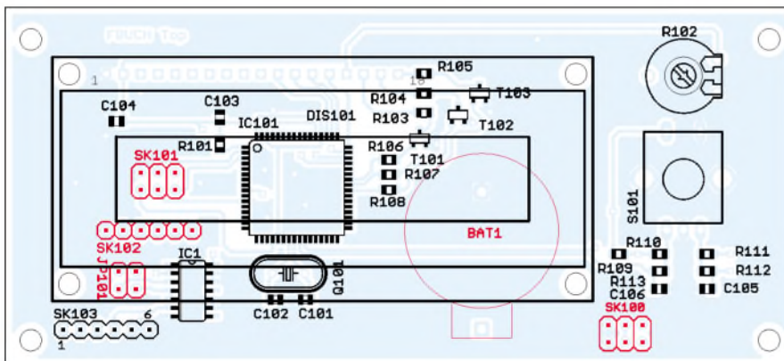
Bild 14: Das Display ist über Abstandshalter der Controllerplatine zu befestigen. Die rot markierten Steckverbinder und der Batteriehalter werden von der Lötseite aus bestückt.
