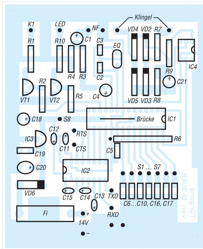
Bild 6: Bestückung der Steuerleiterplatte
