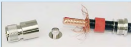
Bild 5: Nach dem Entfernen des Mantels muss man die Schirmung entflechten.
