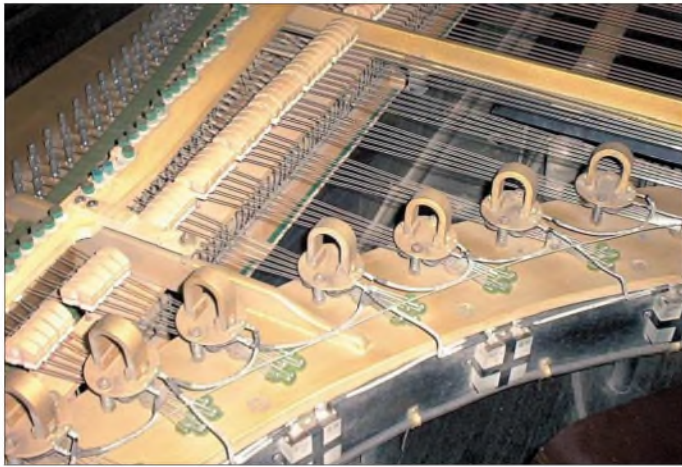
Bild 4: Tonabnehmer und Filterkondensatoren
