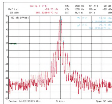
Bild 10: Intermodulation bei 14 MHz und mit 1000 W PEP
