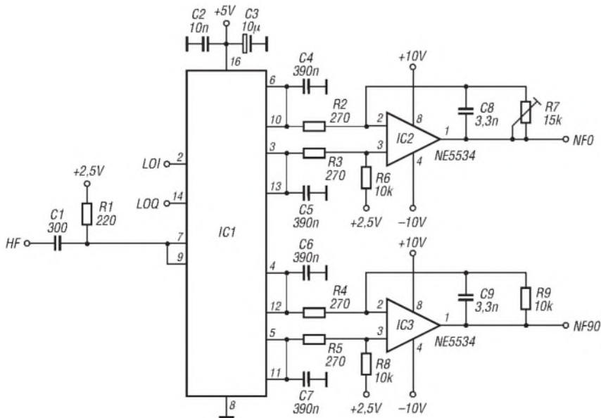
Bild 4: Tayloe-Mischer mit einem FST3253; als Lokaloszillator sind zwei um 90° phasenversetzte Signale erforderlich.
