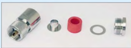
Bild 3: Die Reihenfolge dieser fünf Teile ist bei der Montage der UHF-Stecker einzuhalten.
