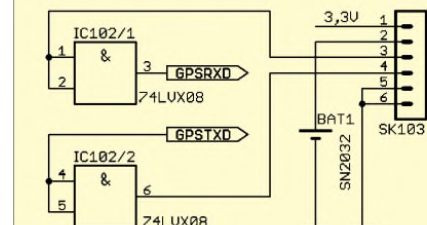
Bild 11: Zur Pegelanpassung zwischen GPS-Modul und Controllerbaugruppe verwenden wir eine Hälfte des 74LVX08.
