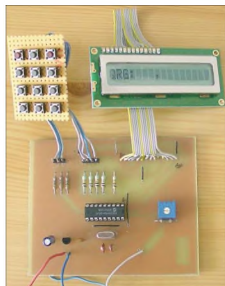
Bild 10: Tastatur und Display sind über kurze Drähte anzustecken. Fotos: DL9DWR
