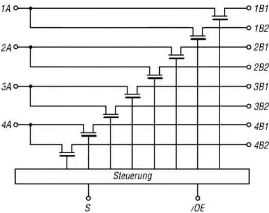
Bild 2: Blockschaltbild des FST3257
