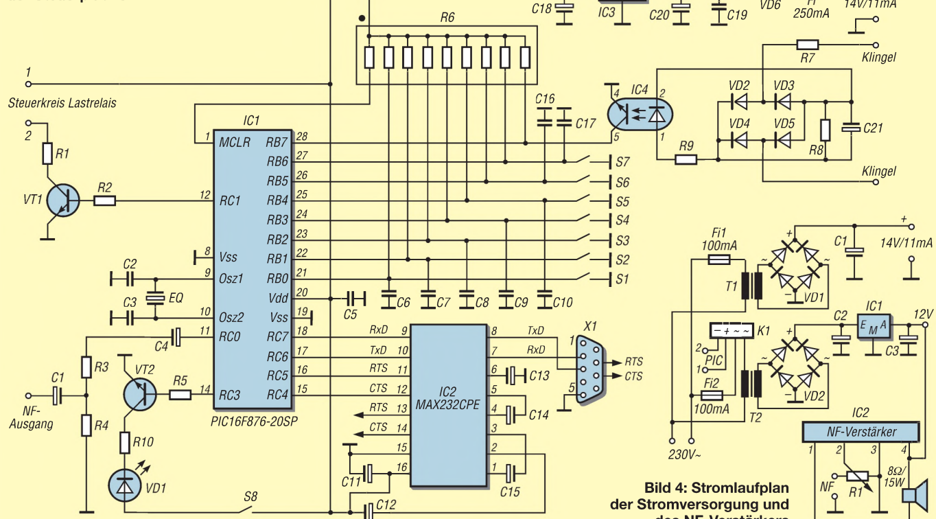
Bild 3: Stromlaufplan der Steuerplatine
