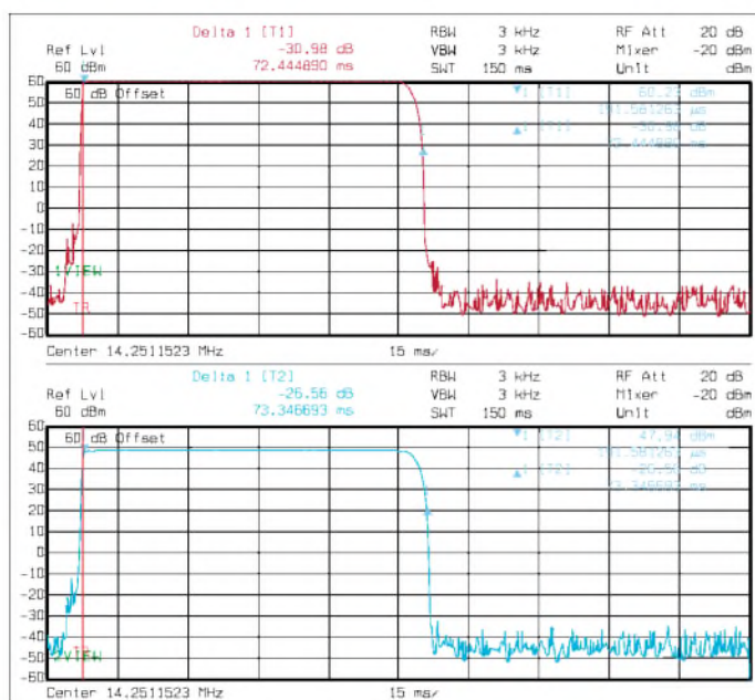
Bild 7: Verkürzung eines CW-Punktes bei Voll-BK: oben Ansteuersignal, unten Ausgangs- signal der Alpin 100 Fotos und Screenshots: DL3KH
