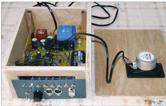
Bild 1: Die Melodieklänge sind in ein Holzgehäuse einzubauen, da es einen guten Klang wiedergibt und hohen Berührungsschutz bietet.
