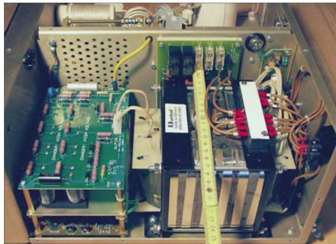
Bild 5: Der Netztrans- formator dominiert die Spannungs- versorgungs- Baugruppe.
