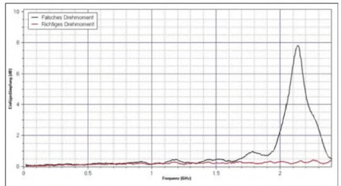
Bild 11: Einfügedämpfung von 0 bis 2,4 GHz an einem Koaxialkabel mit N-Steckern bei richtigem (rot) und falschem (blau) Anzugsmoment des Steckers an der Buchse Fotos und Screenshots: DG6RBP
