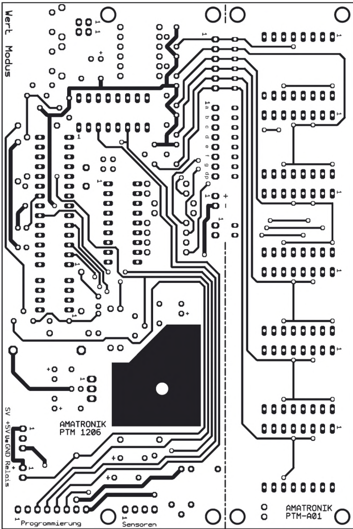
Bild 7: Layout der Bestückungsseite des Temperaturmoduls
