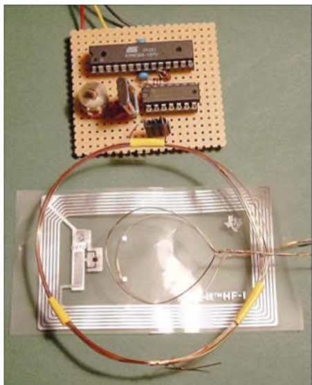
Bild 7: Ansicht der Sendeschialtung mit RFID-Tag und zwei Schnüffelsonden
