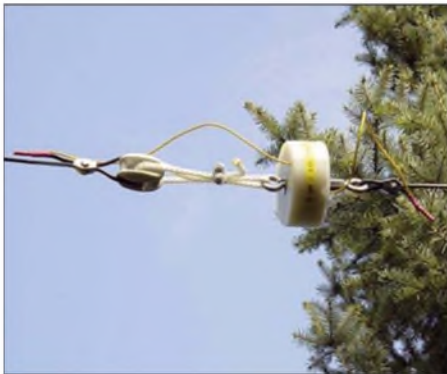
Bild 6: Detailaufnahme des Dämpfungselements im kurzen Schenkel
