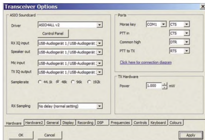
Bild 8: Nutzeroberfläche „MOKGK SDR Transceiver 1.1“
