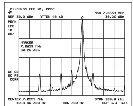
Bild 7: Schmalbandiges Sender-Ausgangsspektrum bei 1 W Dauerstrich (vertikal 10 dB pro Teilstich, horizontal 10 kHz, Mittenfrequenz f = 7,0559 MHz)
