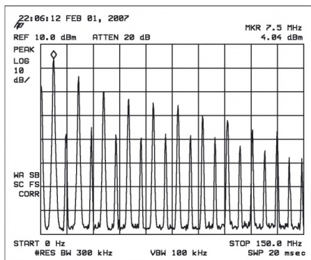
Bild 6: Ausgangsspektrum des QSE bei Ansteuerung für 1 W Dauerstrich (vertikal 10 dB pro Teilstich, horizontal 15 MHz, f = 0...150 MHz)
