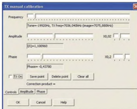
Bild 11: I/Q-Signalgenerator im Programm M0KKG SDR Transceiver 1.1 zum Abgleich der Seitenbandunterdrückung des Senders
