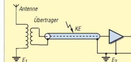
Bild 3: Der eingeschleifte Übertrager unterbindet den Ausgleichsstrom. Allerdings bewirkt der Schirm nun einen gewissen Antenneneffekt durch die kapazitive Einkopplung KE.
