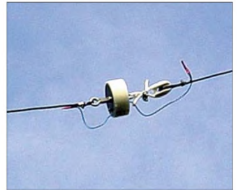
Bild 7: Detailaufnahme des Dämpfungselements im langen Schenkel
