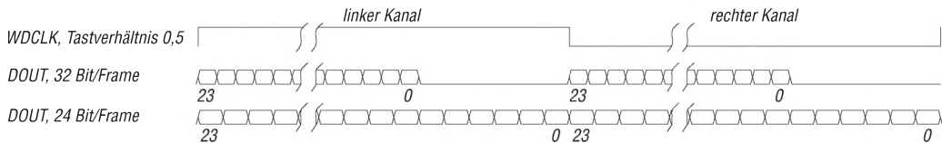
Bild 3: Datenformat des seriellen Ausganges
