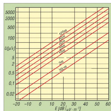
Bild 2: Zusammenhang zwischen elektrischer Feldstärke E im Raum, angegeben in \text{dB} bezogen auf 1 \mu V/m , und der Spannung U an einem mit R = 50 \Omega abgeschlossenen Isotropstrahler für Amateurfunkbänder 70 cm bis 160 m
