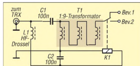
Bild 6: Fernbediente Umschaltung zweier Beverage-Antennen
