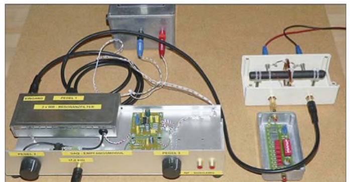
Bild 7: Anordnung der Empfangsbaugruppen für SAQ; rechts ist der Schleifenkoppler zu sehen. Die Antennenanschlüsse erfolgt über eine Zweidrahtleitung. Vor dem Koppler befindet sich die Platine VK2 zur Frequenzeinstellung mittels DIL-Schalters.
