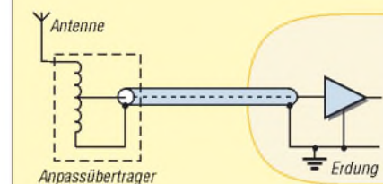
Bild 4: Verschleppung des Antennenbezugspekts in die Störzone, mit einhergehendem Antenneneffekt des Schirms.
