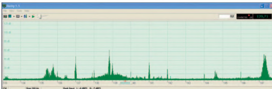
Bild 3: Der Screenshot von Rocky zeigt den Bereich von 133 bis 147 kHz. Deutlich sind (v. r. n. l.) DDH47 ( Deutscher Wetterdienst), DCF39 Burg, ein Amateurfunksignal auf 137 kHz und ein weiterer kommerzieller Sender bei 135 kHz zu erkennen. Foto und Screenshot: DK1KQ
