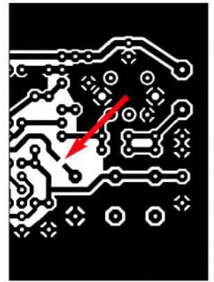
Bild 4: Im Layout- ausschnitt ist auf der Unterseite der Platine an der markierten Stelle der Leiterzug zum Oszillator aufzu- trennen.
