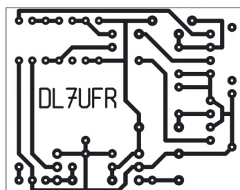
Bild 5: Layout des Wandler für die RS232-Schnittstelle
