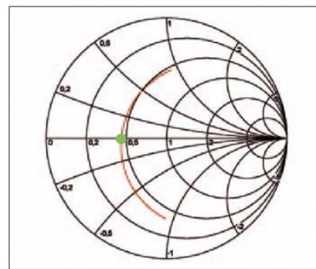
Bild 6: Impedanzverlauf der 10-m-Groundplane (ohne L-Netzwerk) von 27 bis 30 MHz, dargestellt im Smith-Diagramm; der grüne Punkt markiert 28,5 MHz.
