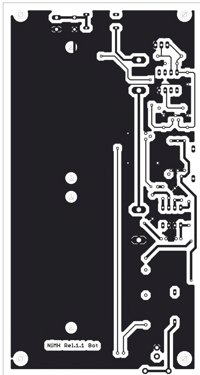
Bild 3: Layout der Unterseite der Ladebaugruppe
