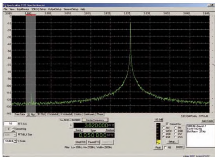
Bild 4: Darstellung eines 190 kHz breiten Ausschnitts des 80-m-Bands mit SpectraVue, links der CW- und rechts ein Teil des SSB-Bereichs
