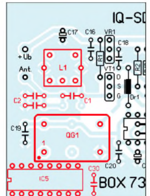
Bild 5: Wie dieser Teil der Bestückung zeigt, passen der zusätzliche IC und der Kondensator noch auf einer Uni- versalleiter- platte zwischen QG1 und Gehäuse- wand.
