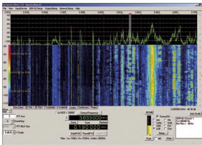
Bild 5: Testmessung mit zwei sinusförmigen Signalen mit Pegeln von -10 und -111 dBm am Eingang des SDR-IQ
