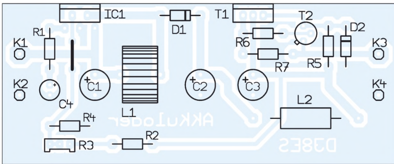
Bild 5: Bestückung erfolgt von der bis auf die Freisenkungen noch voll kaschierter Seite aus.
