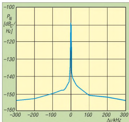
Bild 9: Phasenrauschen im Bereich von 14,274 MHz \pm 300 kHz, gemessen in SSB bei 2,4 kHz Bandbreite; siehe Text
