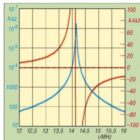
Bild 6: Impedanzverlauf des CWL-Traps für 20 m
