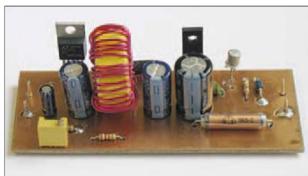
Bild 1: Der betriebsbereite Prototyp des Akkuladers, hier noch ohne Kühlfläche
