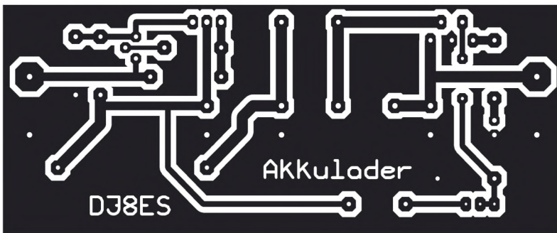
Bild 4: Layout der Leiterbahnseite der zwei-seitig kaschierten Platine des Akkuladers
