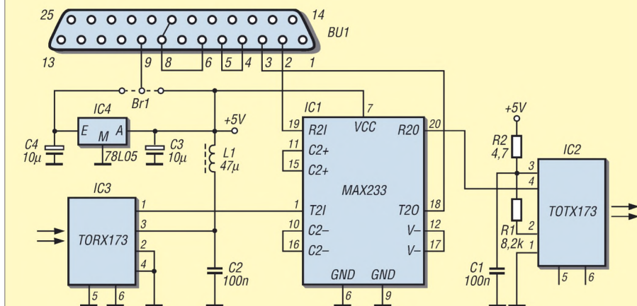
Bild 4: Stromlaufplan der Wandlerbaugruppe für die RS232-Schnittstelle
