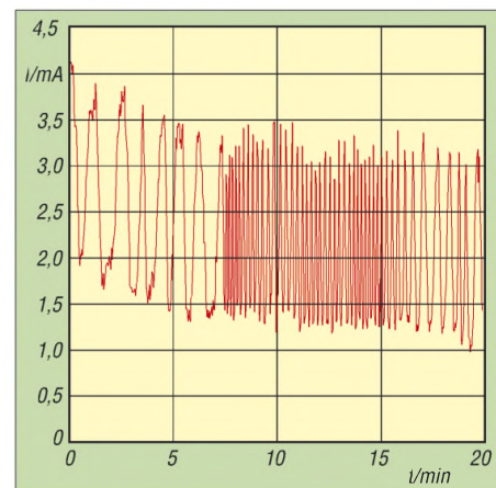
Bild 7: Der sich nach einiger Zeit einstellende Restladestrom unterliegt stets gewissen Schwankungen.
