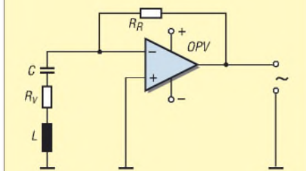
Bild 8: Reihenschwingkreis mit invertierendem Pufferverstärker
