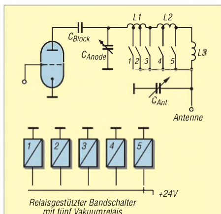
Bild 4: Prinzipschaltbild des Bandumschalters mit Relais. L1 ist die Spule für 10 bis 30 m, L2 deckt das 40-m- und das 80-m-Band ab und L3 das 160-m-Band. L2 und L3 sind im PA-Prototypen [3] mit jeweils zwei gestockten Ringkernen AMIDON T-300 realisiert.
