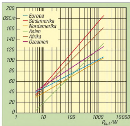
Bild 1: QSO-Rate in Abhängigkeit der Ausgangsleistung für die Sieger pro Kontinent im WPX-SSB-Contest 2001
