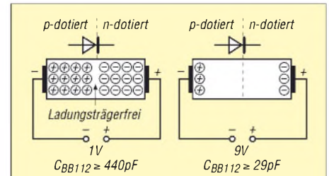
Bild 7: Prinzip der Kapazitätsdiode
