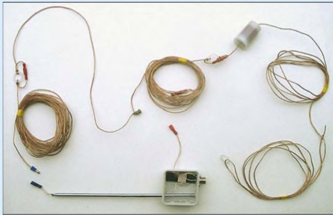
Bild 5: SQ-Vertikal vor dem Aufbau, links speisepunktseitiges Ende, unten Anschlusskasten mit Teleskopstab, Mantelwellensperre, PL-Buchse und Erddungsanschluss (rot), rechts oben Verlängerungsspule in der Filmdose, rechts unten das nach der Abspannöse umgeschlagene Drahtende zum Abgleich auf 80 m
