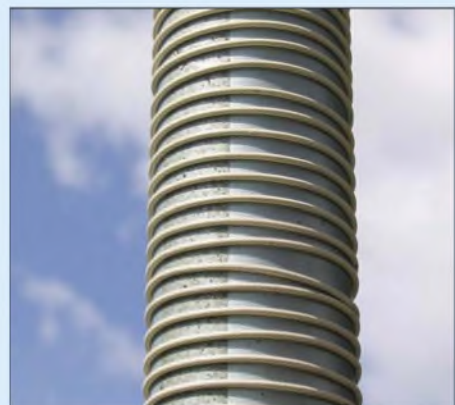
Bild 1: Teilansicht der mit isoliertem Draht, Außendurchmesser 1,25 mm, bei 4 bis 5 mm Steigung bewickelten Angelrute.
