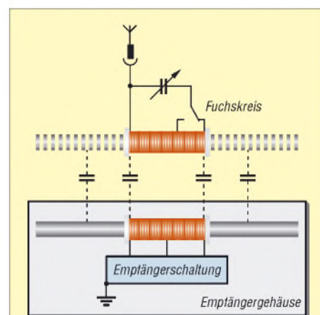
Bild 2: Stromlaufplan des Fuchskreises und Kopplung mit dem Empfänger
