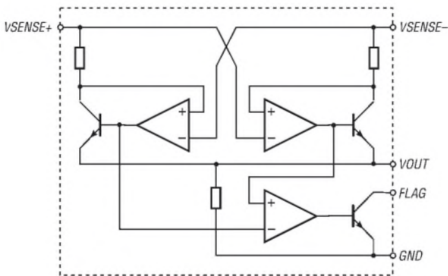
Bild 1: Blockschaltbild des ZXCT1041
