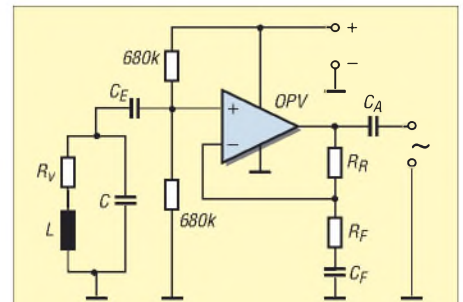
Bild 9: Parallelschwingkreis mit unipolar gespeistem Pufferverstärker; sein Eingangswiderstand wird von den beiden 680\text{-k}\Omega -Widerständen bestimmt.
