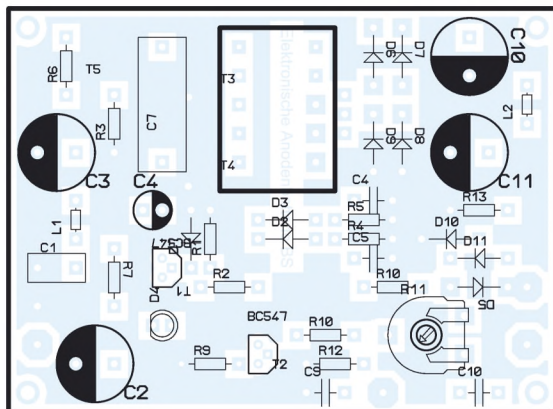
Bild 6: Bestückung der Oberseite der elektronischen Anodenbatterie
