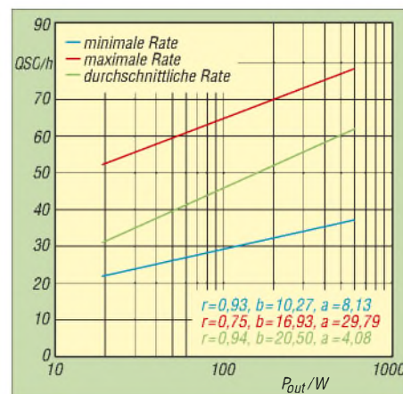
Bild 4: Minimale, durchschnittliche und maximale QSO-Rate für OE5XWM im WPX-Contest 2002, CW, in Abhängigkeit der Sendeleistung
