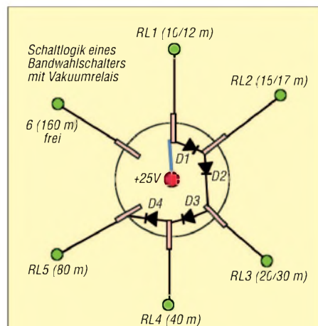
Bild 5: Schaltlogik zur Umschaltung der Bänder mit einem Drehschalter mit sechs Stellungen und nur einer Schaltebene: Schalter auf 1, schaltet Relais 1 und über die Dioden 1 bis 4 alle anderen Relais; Schalter auf 2 schaltet analog RL2 bis RL5; Schalter auf 3 schaltet RL3 bis RL5; Schalter auf 4 schaltet RL4 und RL5; Schalter auf 5 schaltet RL5; Schalter auf 6 schaltet kein Relais.
