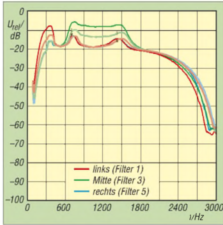
Bild 12: Charakteristik von drei der fünf Contour-Filter; die oberen Kurven entsprechen Anhebung 2 die unteren Anhebung 1.
