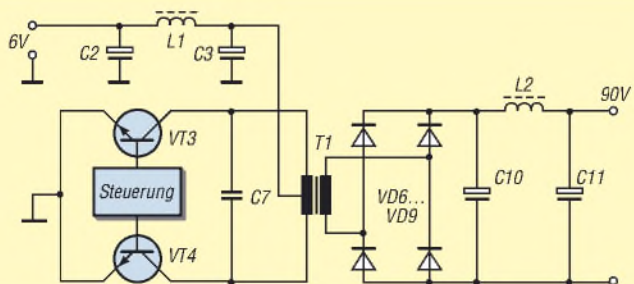
Bild 2: Aufbau eines Royer-Konverters; Der Transformator T1 und der Kondensator C7 bilden einen stark bedämpften Schwingkreis zum Abrunden der Schaltflanken des Gegentaktwandlers.
