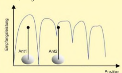
Bild 7: Ausnutzen der räumlichen Leistungsverteilung mit versetzten Diversity-Antennen
