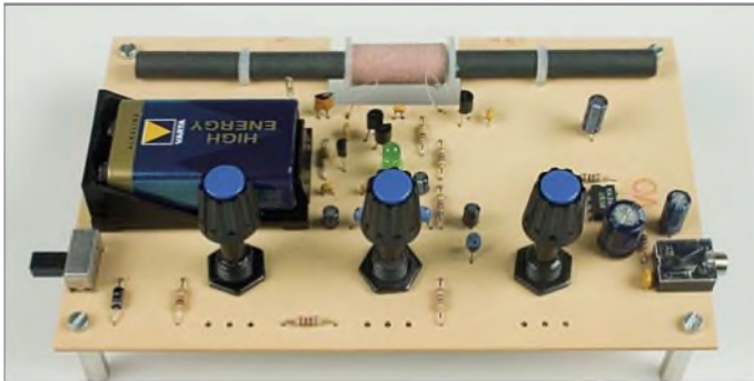
Bild 1: Ansicht der Musterplatte des Einkreisers; die Potenziometer werden direkt in der Leiterplatte verschraubt.
