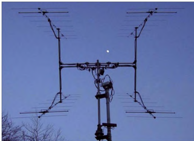
Meist zum Mond ausgerichtet: die Gruppe von vier Achtelement-Yagis bei Steffen, DD0VF
