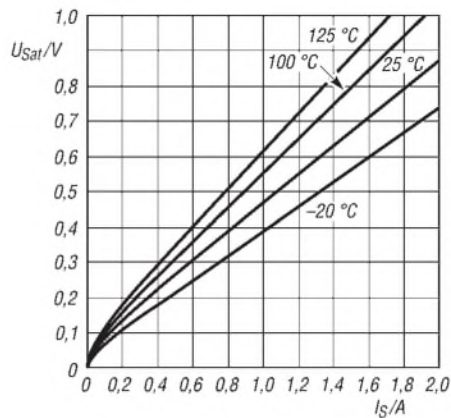
Bild 4: Sättigungsspannung U_{\text{Sat}} in Abhängigkeit vom Schaltstrom I_S bei unterschiedlichen Übergangstemperaturen
