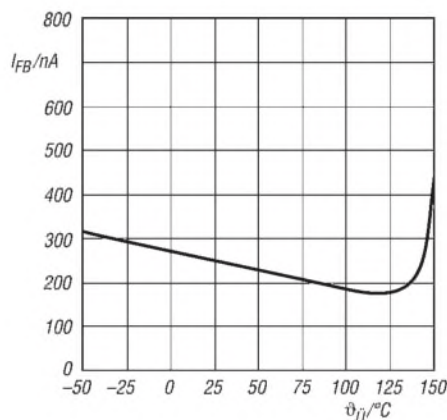
Bild 6: Rückkopplungsstrom I_{\text{FB}} in Abhängigkeit von der Betriebstemperatur, wenn die Rückkopplungsspannung U_{\text{FB}} identisch mit der Referenzspannung U_{\text{Ref}} ist
