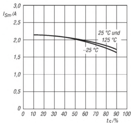
Bild 5: Maximaler Schaltstrom I_{\text{Sm}} in Abhängigkeit vom Taktzyklus t_S bei unterschiedlichen Übergangstemperaturen
