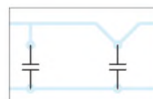
Bild 12: Ungeschickter (links) und geschickter (rechts) Anschluss eines Abblockkondensators
