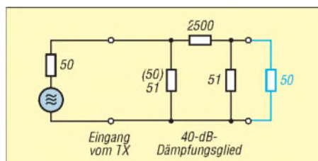
Bild 13: Schaltung des 40-dB-Dämpfungsgliedes; korrekte 40 dB nur bei Abschluss mit 50 \Omega (hier in Blau)!
