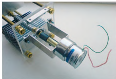
Bild 8: Gleichstrommotor
