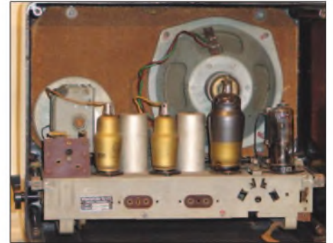
Bild 9: Innenansicht des Standard-Supers mit U-Topfröhren
