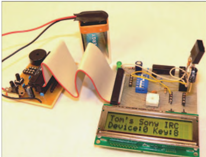
Bild 1: MikroKid2 mit angeschlossener Batterie und Experimentierboard Experiment 2 , hier mit einem Infrarotsensor
