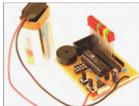
Bild 2: MikroKid2 mit Batterie und elf LEDs für erste Experimente; ohne LEDs dient die Anschlussleiste zum Anstecken der verfügbaren Erweiterungsboards.
