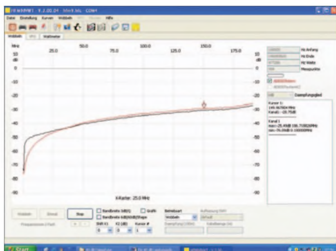
Bild 9: Messergebnis in der NWT-Betriebsart Z-Impedanz (schwarz 50 Ω, violett 2 × 100 Ω)
