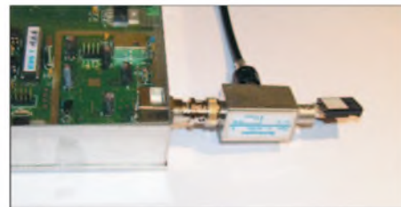
Bild 6: Messaufbau zur Messung der Reflexionsdämpfung gemäß Bild 5
