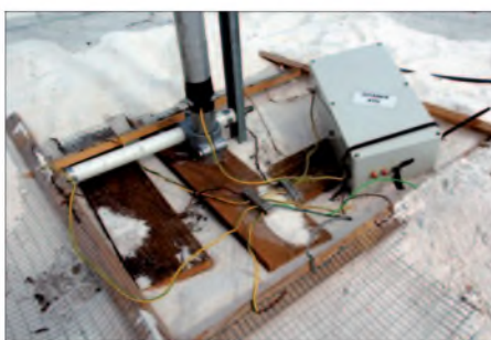
Wohl nicht ganz nach VDE; die Einspeisung der V160S-Vertikalantenne
