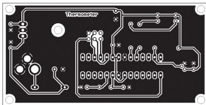
Bild 4: Die Platine des Thermometers ist 86,7 mm × 43,5 mm groß.
