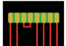
Bild 3: SMD-Pads ohne dazwischenliegende Stopplackstege; die stopplackfreie Fläche ist grün.
