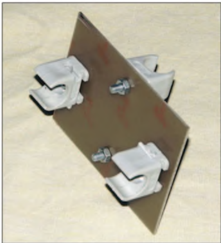
Bild 9: Halteplatte als Kreuzstück zur Befestigung des Booms an einer Angelrute
