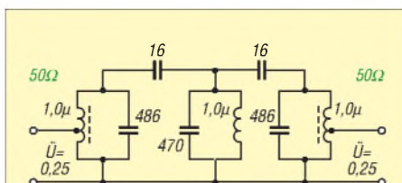
Bild 5: Entwurf des dreikreisigen LC-Bandpassfilters für 40 m, mit AADE Filter Design als „Coupled Resonator“-Bandpass
