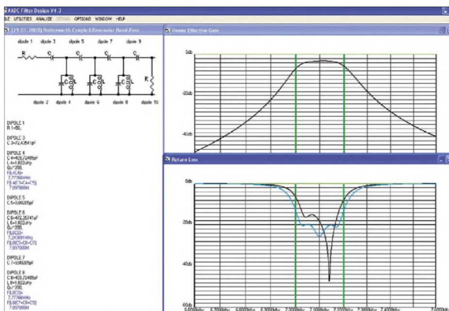
Bild 7: Entwurf des dreikreisigen LC-Bandpassfilters für 40 m, mit AADE Filter Design als „Coupled Resonator“-Bandpass; oben Durchgang, unten Reflexionsdämpfung, schwarz: Originalentwurf, blau: verfeinerter Entwurf von DK4SX (durch Fotomontage hier hinzugefügt)
