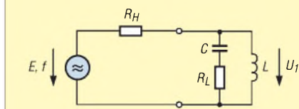
Bild 4: Bedämpfung mit einem in Reihe zum Kondensator liegenden Widerstand: U_1 = E/2
