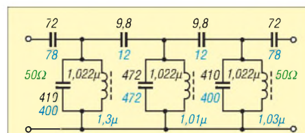
Bild 6: Schaltbild des dreikreisigen LC-Bandpassfilters für 40 m, Werte in Schwarz mit AADE Filter Design ermittelt, in Blau durch DK4SX auf bestmögliche Anpassung optimiert
