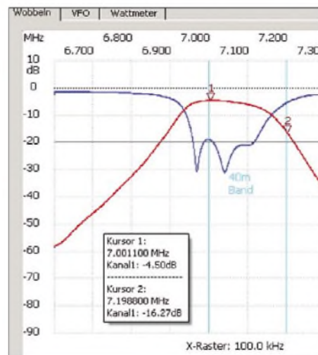
Bild 3: Durchgangsverhalten (rot) und Reflexionsdämpfung eines keramischen Filters SFE7.02, gemessen mit dem FA-NWT
