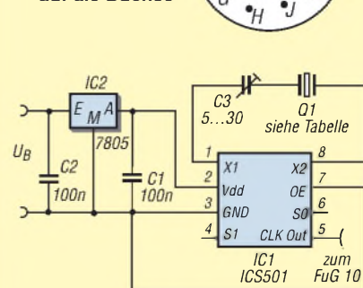
Bild 5: Stromlaufplan des mit dem ICS501 realisierten Quarzersatzes
