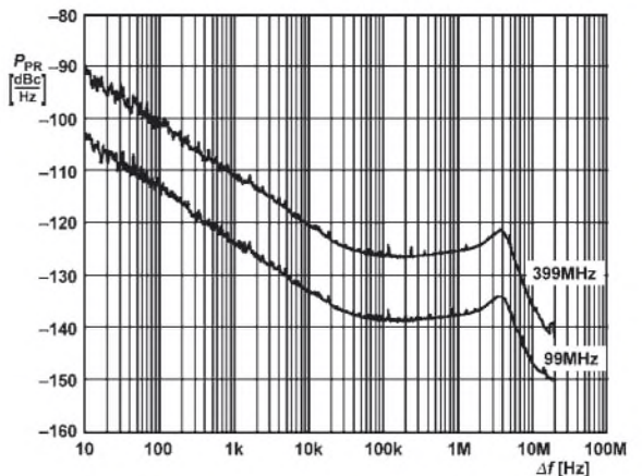
Bild 8: Restphasenrauschen in Abhängigkeit vom Frequenzabstand \Delta f bei Nutzung des HSTL-Treibers; f_A = 99 \text{ bzw. } 399 \text{ MHz} ; f_{\text{CLK}} = 1 \text{ GHz} , PLL mit 25 MHz versorgt
