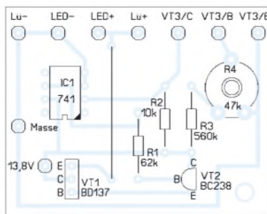
Bild 5: Bestückungs- plan der Lüfter- steuerung
