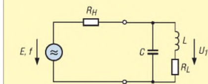
Bild 5: Gleichwertig zu Bild 4, wobei jedoch die Bedämpfung mit einem in Reihe zur Spule liegenden Widerstand erfolgt
