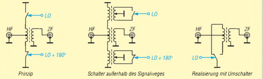
Bild 15: Links das Prinzip (Schalter noch im Signalweg), Mitte und rechts die möglichen Grundschaltungen
