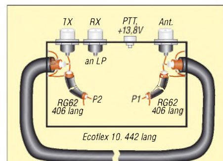
Bild 3: Schema des fertigen QRO-Umschalters. Die erforderlichen \lambda/4 -Stücke werden durch deutlich höher belastbare Kabelstücke realisiert. Der Mehraufwand im Vergleich zur Normalausführung ist minimal. Die RG62-Stücke passen mit in das Gehäuse, die Einführungen für das Umwegstück Ecoflex 10 sollten mit Silikon abgedichtet werden.
