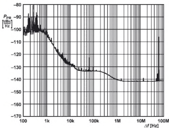
Bild 5: Restphasenrauschen in Abhängigkeit vom Frequenzabstand \Delta f am ungefilterten D/A-Umsetzerausgang; f_A = 311,6 \text{ MHz} ; f_{\text{CLK}} = 1 \text{ GHz} , PLL ausgeschaltet
