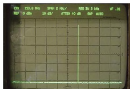
Bild 5: Ausgangssignal beim ersten Test der Hybrid-Platine mit externem 1-GHz-Takt
