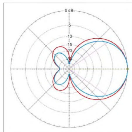
Bild 8: Horizontales (blau) und vertikales (rot) Strahlungsdiagramm im Freiraum bei 14,2 MHz, äußerer Ring entspricht 7,35 dBd.
