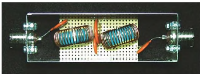
Bild 1: Musteraufbau des Filters für das 40-m-Band auf einer Lochasterplatte
