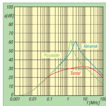
Bild 17: Vergleich der Einfügedämpfung dreier Kondensatoren mit jeweils 1 \mu\text{F} unterschiedlicher Bauformen Quelle: [11]
