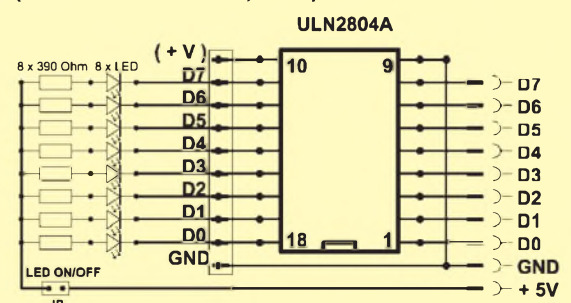
Bild 31: Schaltbild der Zusatzbaugruppe X04 (Port-A/B-Relaistreiber, LEDs)
