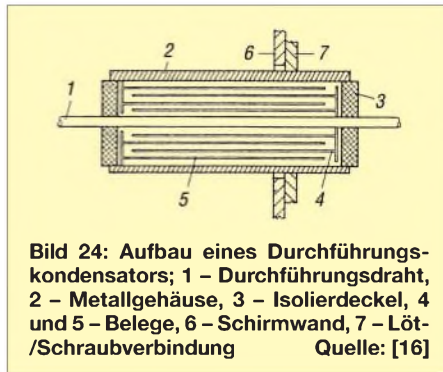
Bild 24: Aufbau eines Durchführungskondensators; 1 – Durchführungsdraht, 2 – Metallgehäuse, 3 – Isolierdeckel, 4 und 5 – Belege, 6 – Schirmwand, 7 – Löt-/Schraubverbindung Quelle: [16]
