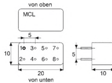
Bild 2: Pinbelegung
