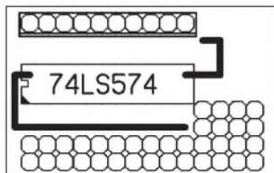
Bild 24: Bestückungsplan Platine X01
