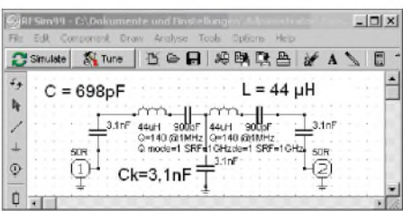
Bild 7: Entwurf des Bandpassfilters mittels RFSim99, normiert für 1 MHz und 50 \Omega
