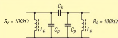
Bild 2: Klassisch: das Bandfilter mit Parallelschwingkreisen
