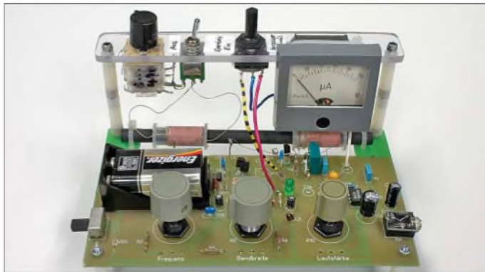
Bild 1: Musteraufbau des MW-Einkreis mit allen beschriebenen Verbesserungen; links oben sind Foliendrehkondensator und zweite Wicklung für die nur in Sendernähe notwendige Nachrüstung (8) zu erkennen.
