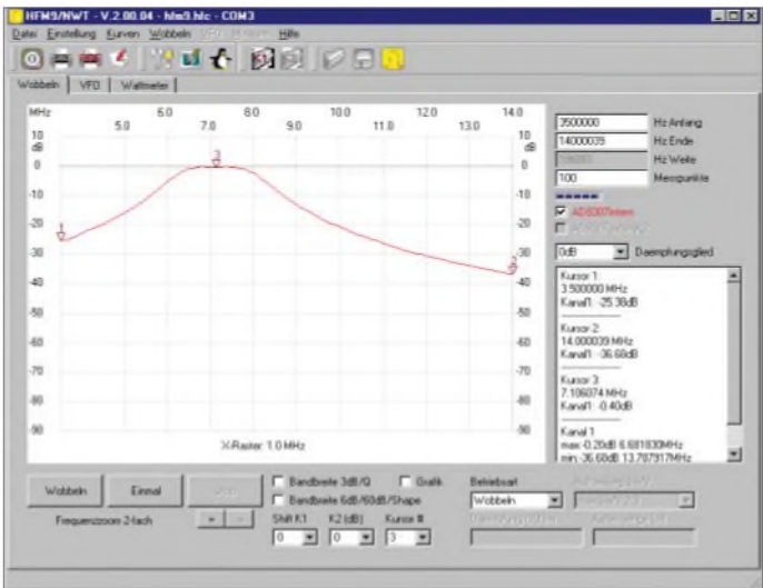
Bild 5: Abgleich der Serienschwingkreise mit dem FA-NWT auf die Resonanzfrequenz f_s
