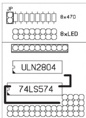
Bild 30: Bestückungsplan Platine X02
