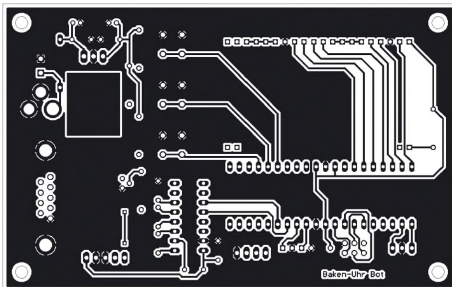
Bild 4: Layout der Lötseite; die Platine ist 120,5 mm × 76 mm groß.
