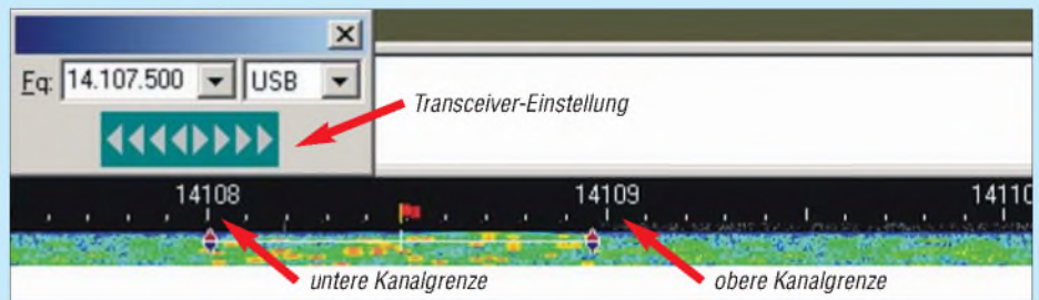
Bild 15: Beispiel zur Abstimmung; eingestellte Frequenz f_{\text{TRX}} (14 107,5 kHz) plus tiefster Ton (500 Hz) = untere Kanalgrenze (14 108 kHz); f_{\text{TRX}} (14 107,5 kHz) plus höchster Ton (1500 Hz) = obere Kanalgrenze (14 109 kHz)
