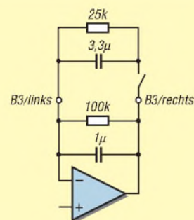
Bild 6: Möglichkeit zur Umschaltung der Verstärkung des Präzisionsgleichrichters auf der UAP6
