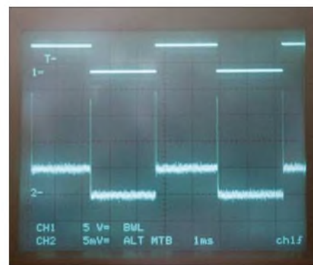
Bild 4: Relevante Signale auf dem Oszilloskop; oben das Referenzsignal, unten das Wechselspannungsausgangssignal bei 50 \mu\text{V} Eingangsspannung und einer Verstärkung von 100; C_2 = 330 \text{ pF} Screenshot: Franke
