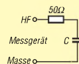
Bild 21: Einsatz eines aktiven Stehwellen- messgeräts zum Ermitteln der Eigen- resonanzfrequenz eines Kondensators
