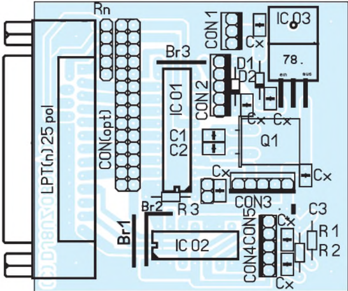
Bild 17: Bestückungsplan für die Platine Version C
