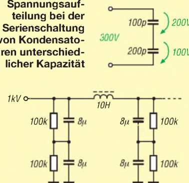
Bild 31: Verwendung von Widerständen als Spannungsverteilung zwischen den in Serie geschalteten Kondensatoren in der Siebung des Netzteils eines Röhrenverstärkers (Auszug) Quelle: [18]
