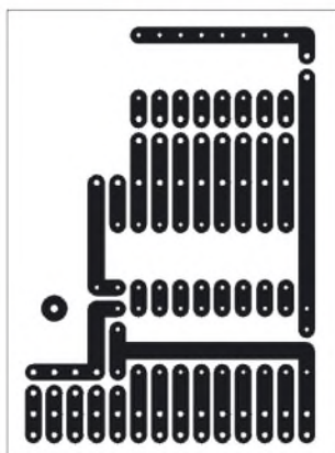
Bild 25: Layout der Platine X02
