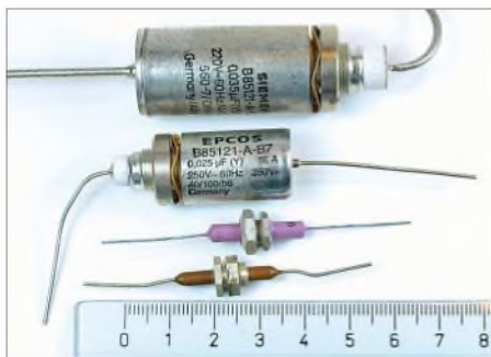
Bild 23: Verschiedene Ausführungen von Durchführungskondensatoren
