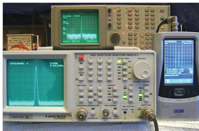
Bild 1: Die Testgeräte: links der HAMEG HM5014-2 [2], rechts der Thurlby-Thandar PA1301T [3], im Hintergrund der fast doppelt so breite und hohe Takeda Riken (Bj. 1984) als Referenz
