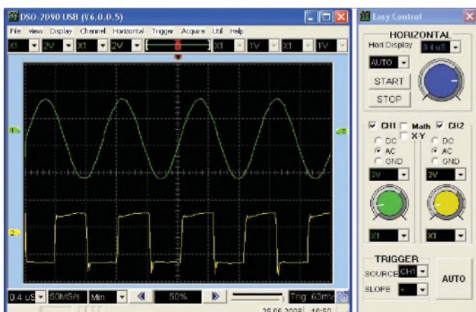
Bild 3: Die Bedienoberfläche des PC-Programms für das Voltcraft DSO-2090USB besteht aus zwei Fenstern.
