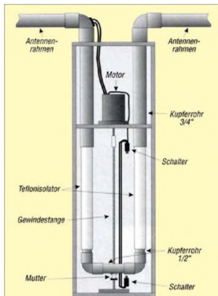
Bild 45: Konstruktionszeichnung für einen selbst gebauten Drehkondensator mit konzentrischen Rohren nach dem Prinzip des Schmetterlingsdrehkondensators Quelle: [23]
