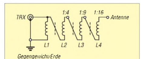
Bild 4: Prinzipschaltbild des Leitungsübertragers bis 1:16
