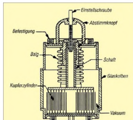
Bild 53: Typischer Aufbau eines Vakuumdrehkondensators Quelle: [24]
