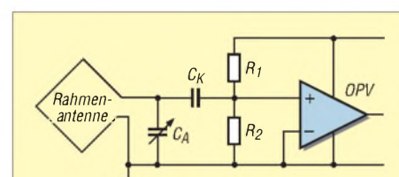
Bild 3: Ankopplung der Rahmenantenne (nur eine Windung gezeichnet) an den Folgeverstärker mit hochohmigem Eingang; die Bewertung von R_1 und R_2 erfolgt mit einigen Hundert Kiloohm.
