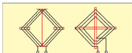
Bild 1: Wicklungsanordnungen von Rahmenantenne: prismatisch (links), spiralförmig (rechts)
