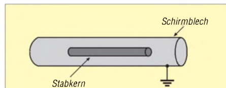
Bild 6: Eine gute Schirmung erfolgt bedämpfungsarm mit ausreichendem Abstand zur Antenne hin. Das Schirmblech sollte den Stabkern an beiden Enden einige Zentimeter überragen.
