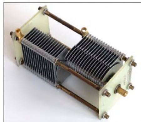
Bild 34: Schmetterlingsdrehkondensator von Annecke; aus dem Plattenabstand von zweimal 3 mm ergibt sich eine Spannungsfestigkeit von 8,4 kV bei 11 bis 110 pF. Das Prinzip des Schmetterlingsdrehkondensators mit zwei Statoren und einem isolierten Rotor dazwischen ist gut zu erkennen.
