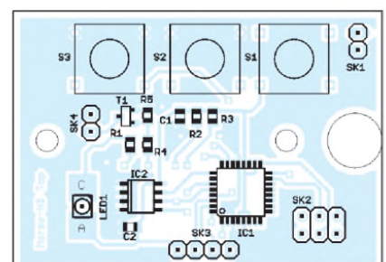
Bild 6: Die Bestückung erfolgt mit SMD-Bauteilen, um eine möglichst geringe Platingröße zu gewährleisten.
