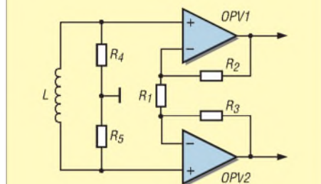
Bild 10: Ankopplungsprinzip einer Antennenspule ohne Anzapfung; die hochohmigen Widerstände R4 und R5 stellen den symmetrischen Bezug zum Massepotenzial her.
