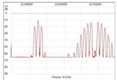
Bild 3: Ein AM- (links) und ein FM-Signal aus zwei Messsendern HP8654B, Modulation 1 kHz, bei 300 Hz Auflösungsbandbreite
