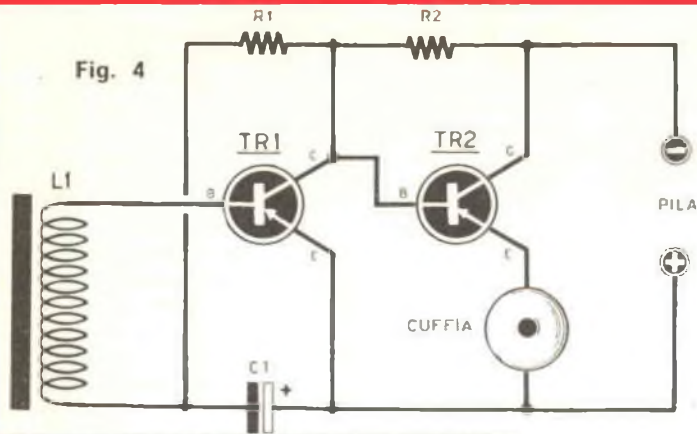
Fig. 4 - Schema elettrico del captatore a due transistor, adatto a coloro che desiderano maggiore potenza. Su questo montaggio è necessario, dopo l'uso, staccare un terminale della batteria.
