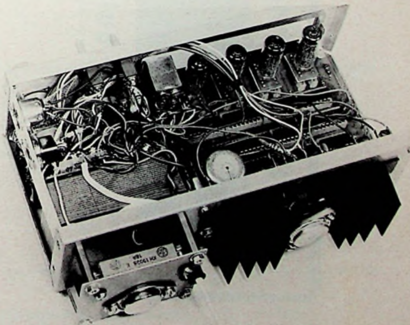
De serie weerstand van 18\Omega bevindt zich tussen de achterwand van de kast en de koelplaat. Let ook op de aluminium strip voor de chassisdelen.
