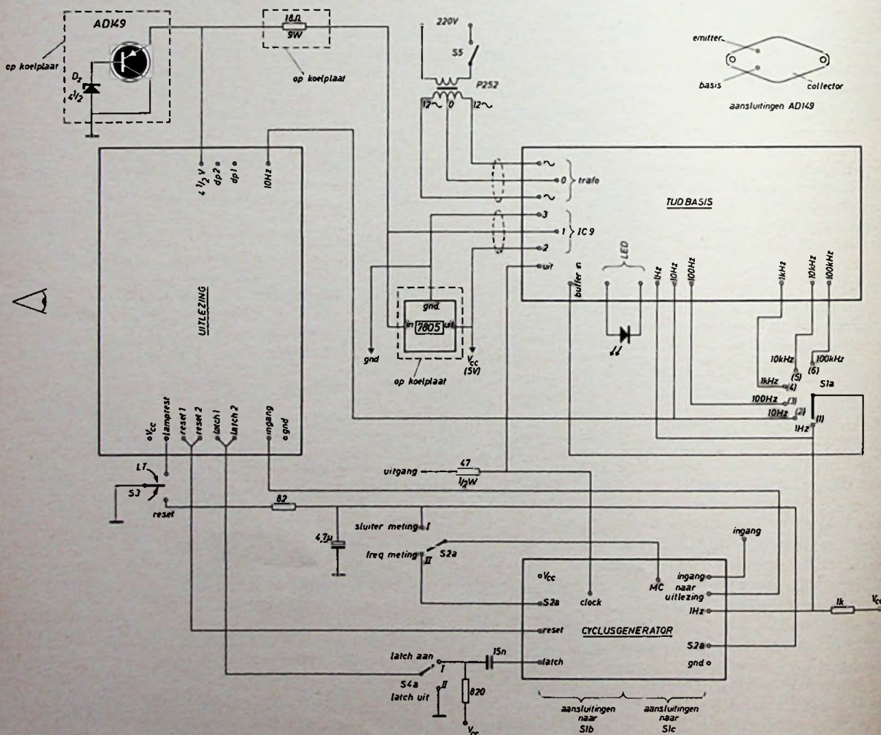
Fig. 2: Bedradingsschema. Bestudeer dit in combinatie met fig. 12 uit deel 2.
