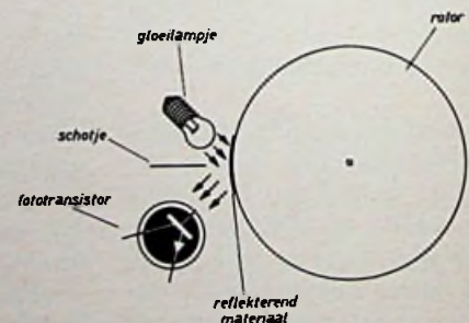
Fig. 7a: Toepassing van de optische detector als omwentelingsteller (in de stand frequentiemeter als toerenteller).
