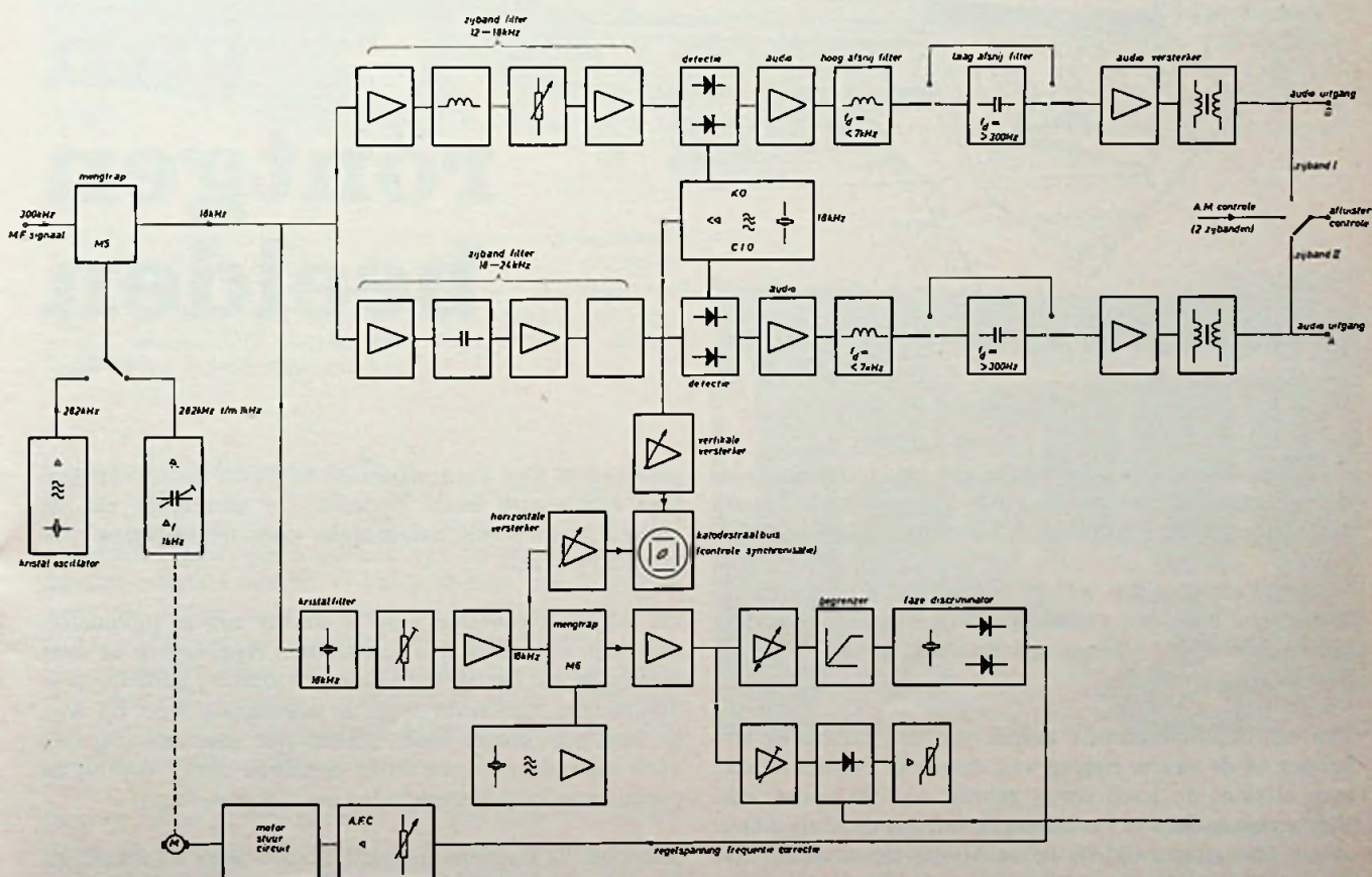
Fig. 11: het blokschema van het gedeelte voor enkelzijdig ontvangst NZ10.
