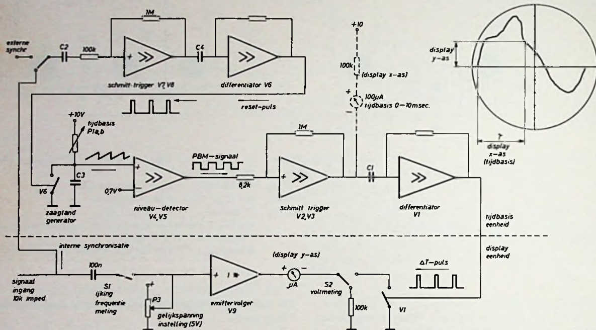
Fig. 6 Principeschema van de Frequentie-, Sample-voltmeter
