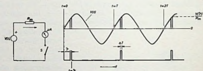
Fig. 3 Sample-voltmeter
