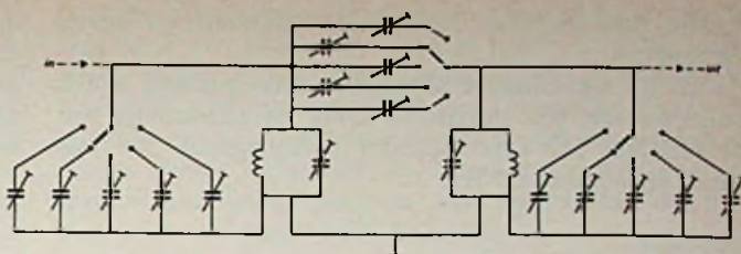
Fig. 10: prinsieschema van de omschakelbare m.f. bandfilters. (deze schakeling in de EK07 4x, 8 LC kringen)!
