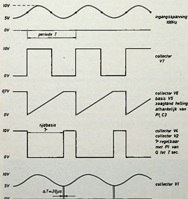
Fig. 5 Spanningsvormen Sample-voltmeter
