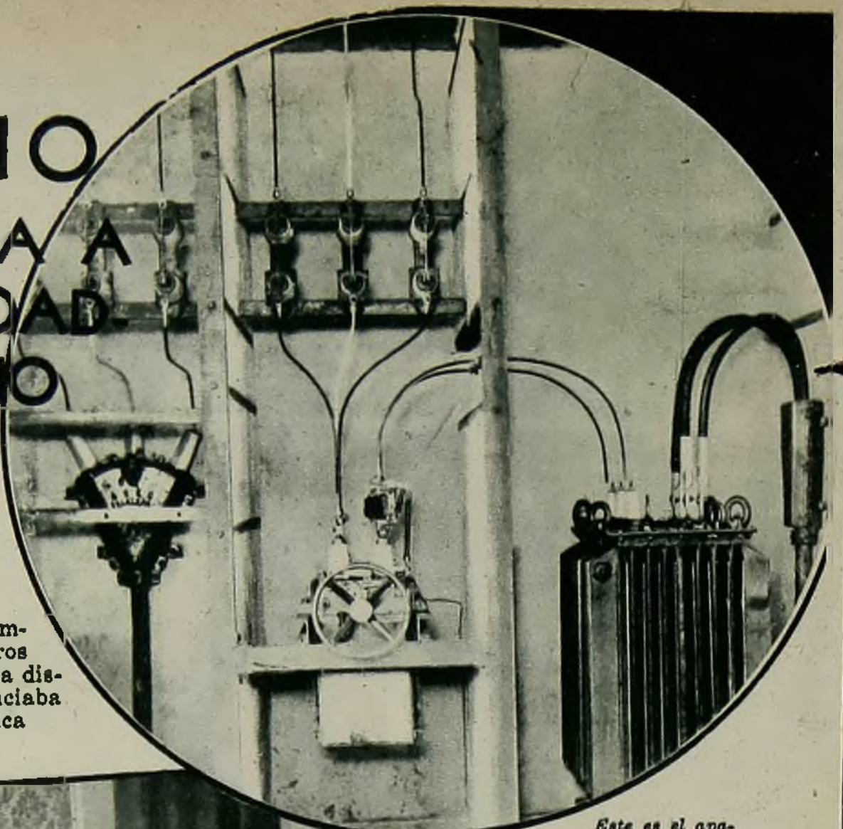
Este es el aparato de alta tensión del primer transmisor que tuvo Radio Nacional cuando estaba en Boyacá. Nótese la confección rudimentaria y "casera" de los aparatos.
