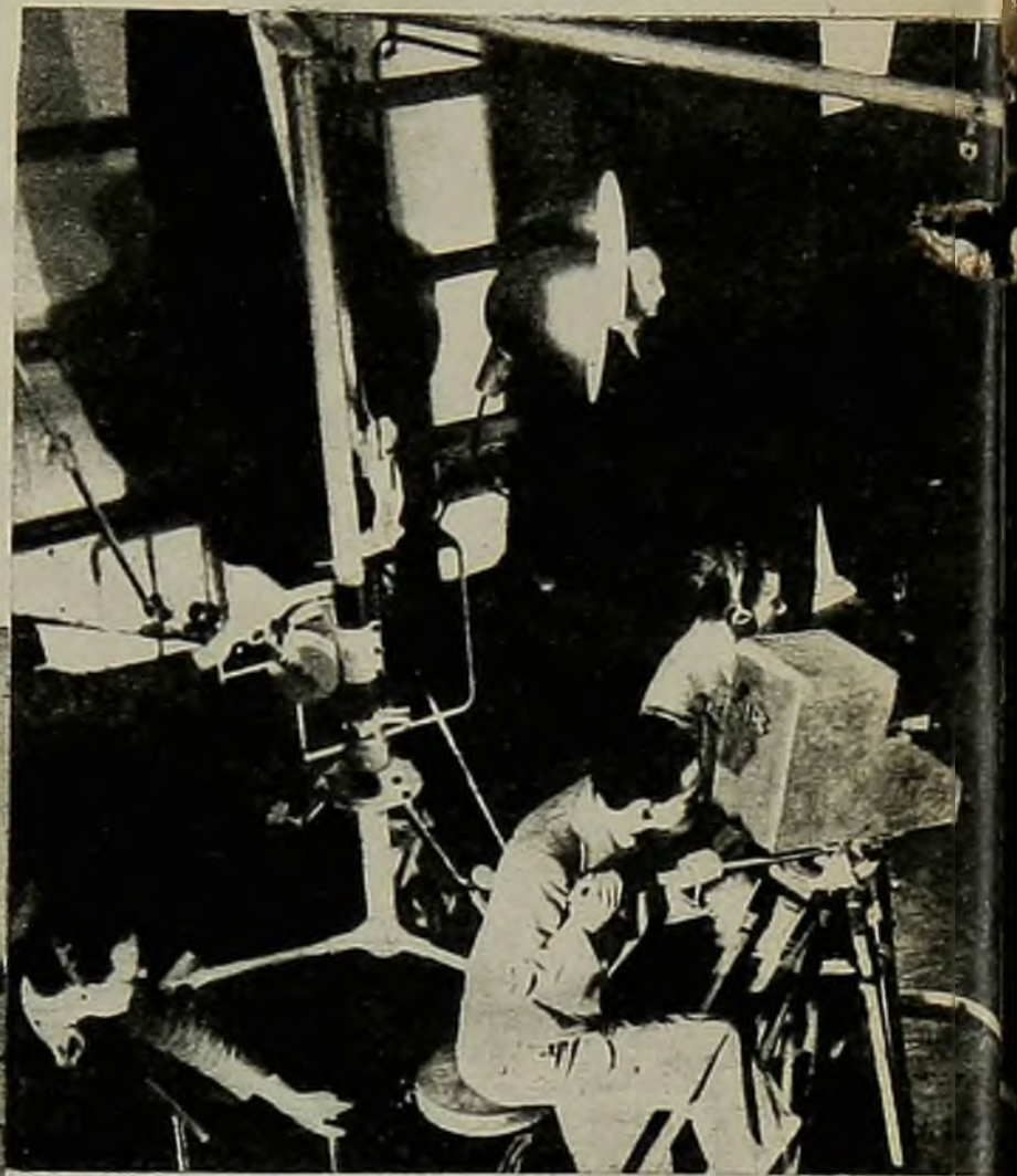
Estudio de una broadcasting de Londres mostrando el "Emiltron", aparato que sirve de cámara en las transmisiones de televisión que se efectúan diariamente.
