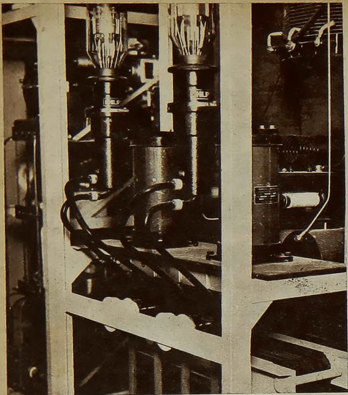
La etapa de poder del nuevo equipo, compuesto por dos válvulas de 5 kilowatts cada una.
