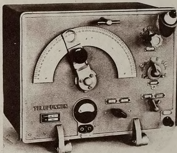
Transmisor de telefonía de 10 vatios
