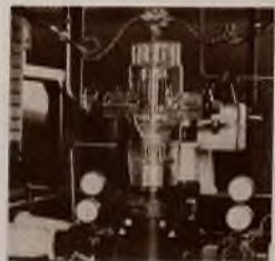
Válvula amplificadora Philips de 100.000 Watts empleada en la última etapa del equipo transmisor
