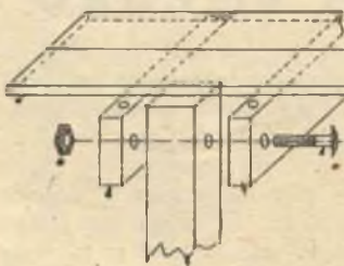
PARTICOLARE MONTAGGIO GAMBIE
