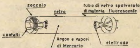
Fig. 1. — Come è costituito un tubo fluorescente.
