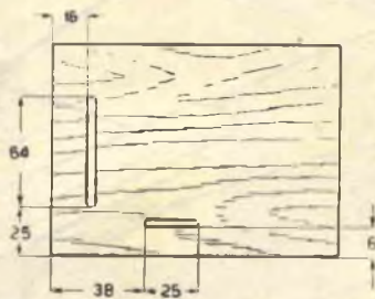
Fig. 3. — Sul coperchio si rende necessario praticare due asole per il passaggio dei partt. 1 e 20 (vedi fig. 1).
