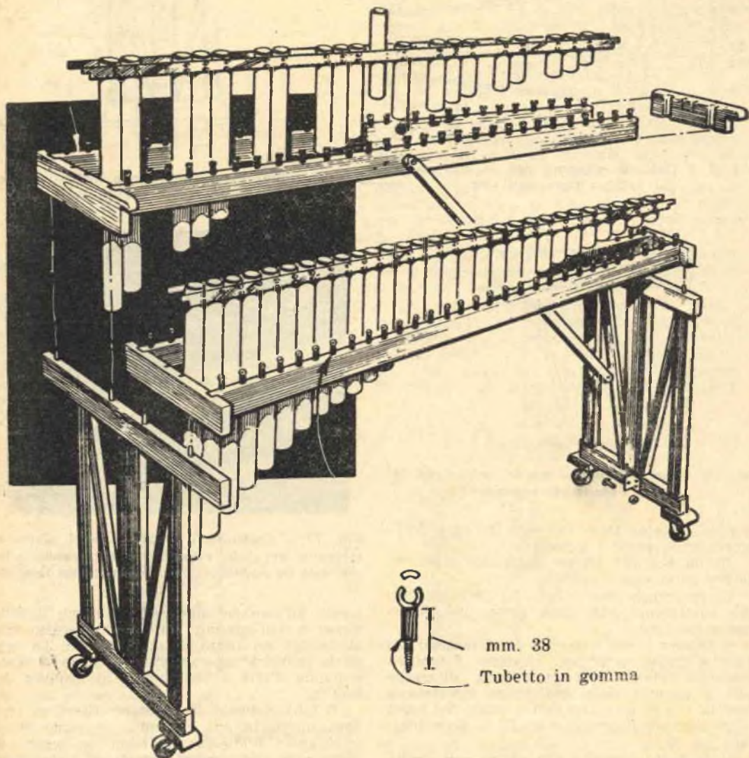
Fig. 13 - Il telaio della « MARIMBA » scomposto nei componenti. In basso: il particolare della vite ad occhio per l'appoggio dei due ordini di tastiera.
